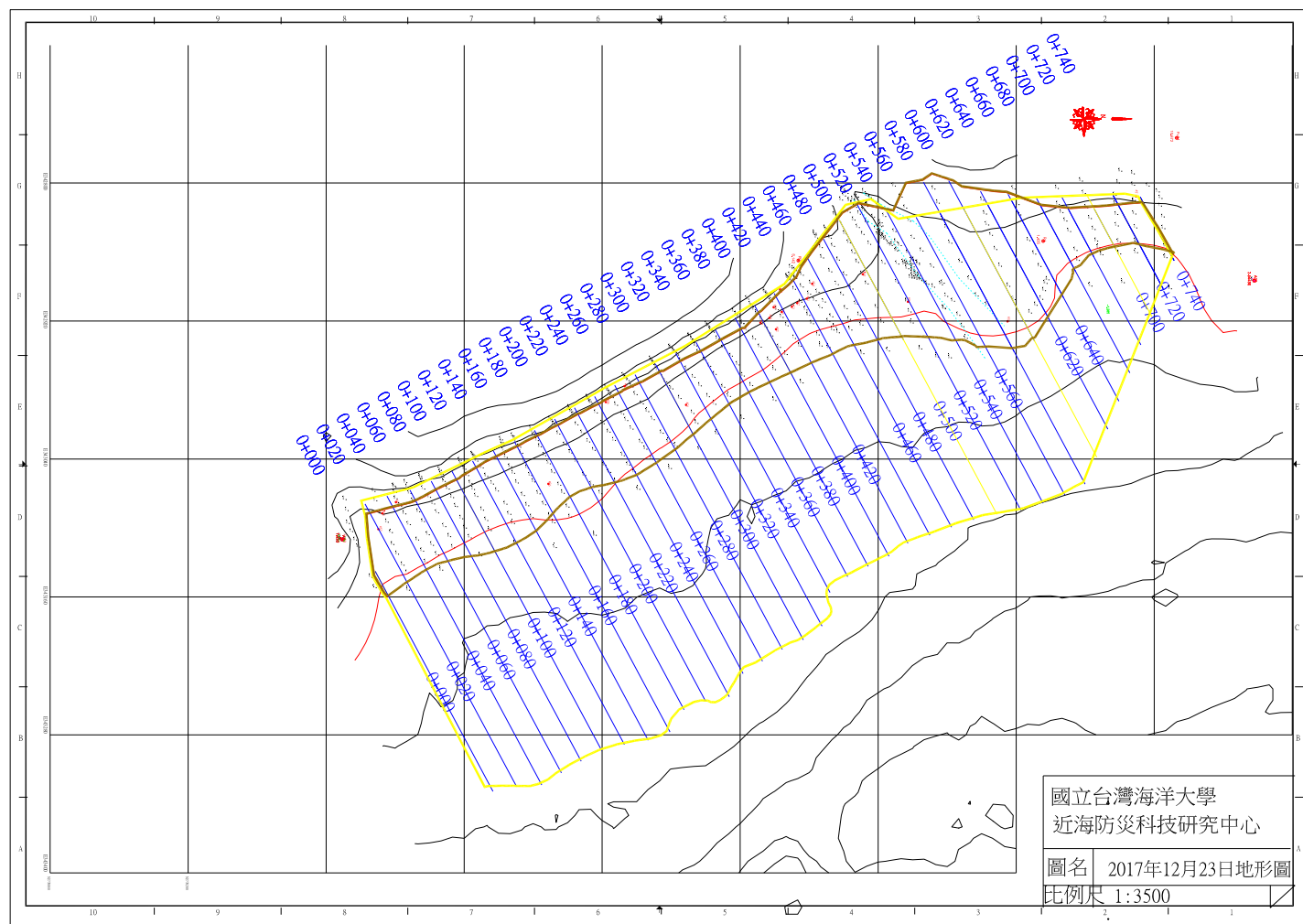
圖 4-1 2017 年 12 月 23 日監測地形圖
