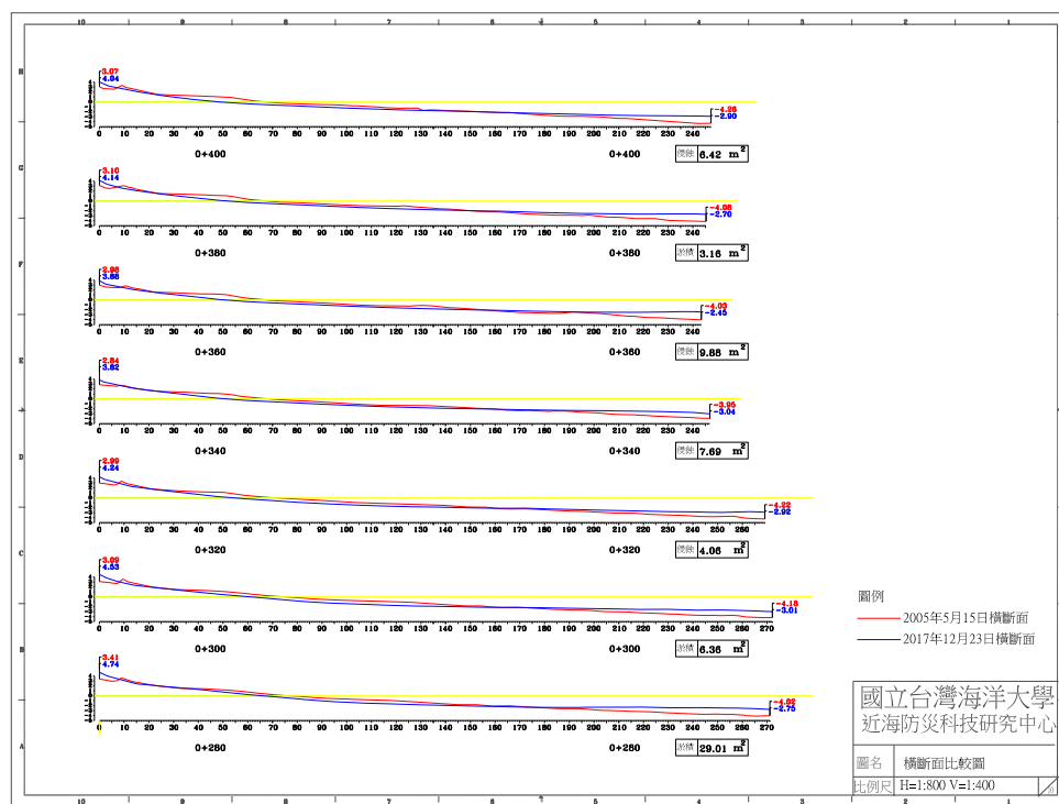
圖 4-5(d) 2017 年 12 月 23 日 B 監測區橫斷面比較圖
