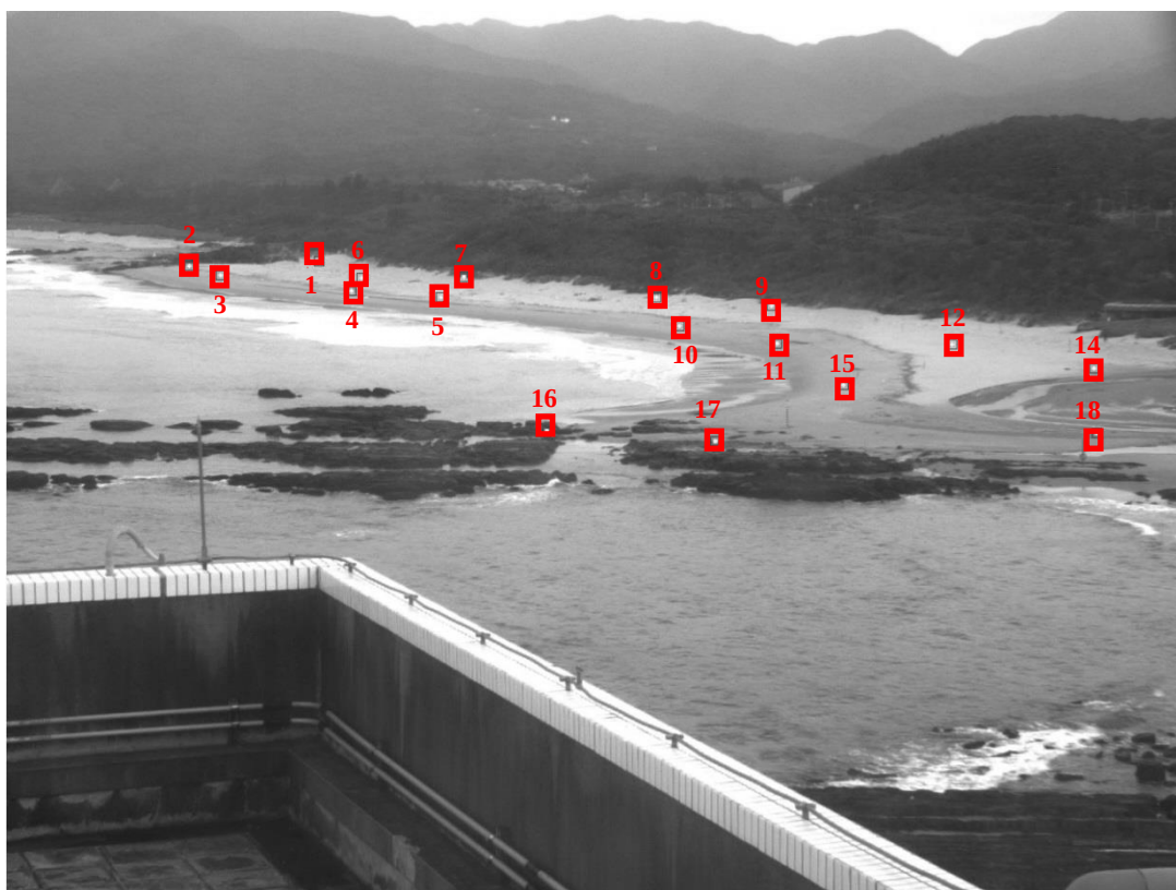
圖 3-20 視角 2(Cam2)地面控制點位置分佈圖例(2016/05/12)
