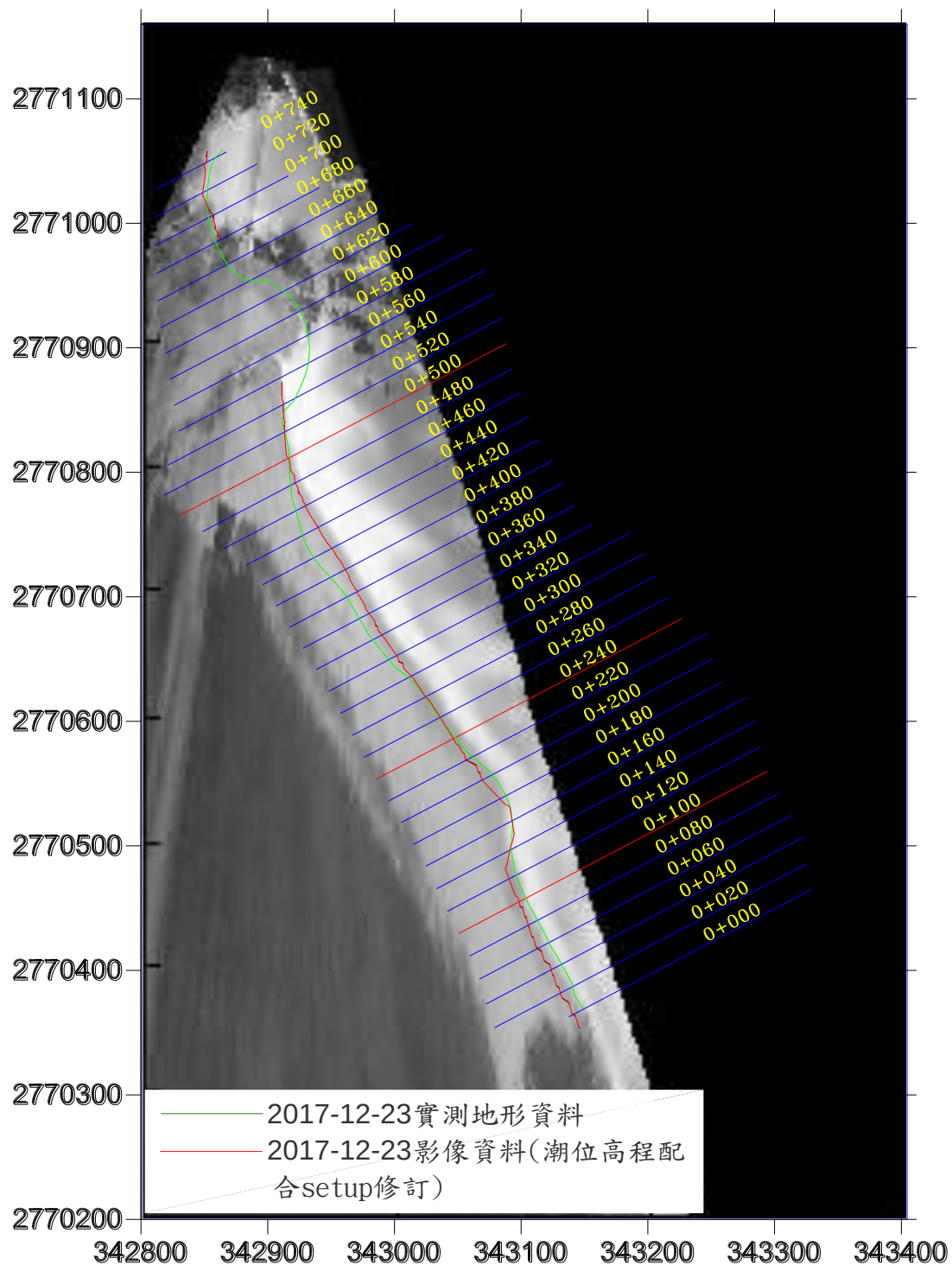
圖 3-22 水位線分析結果圖(2017/12/23)
