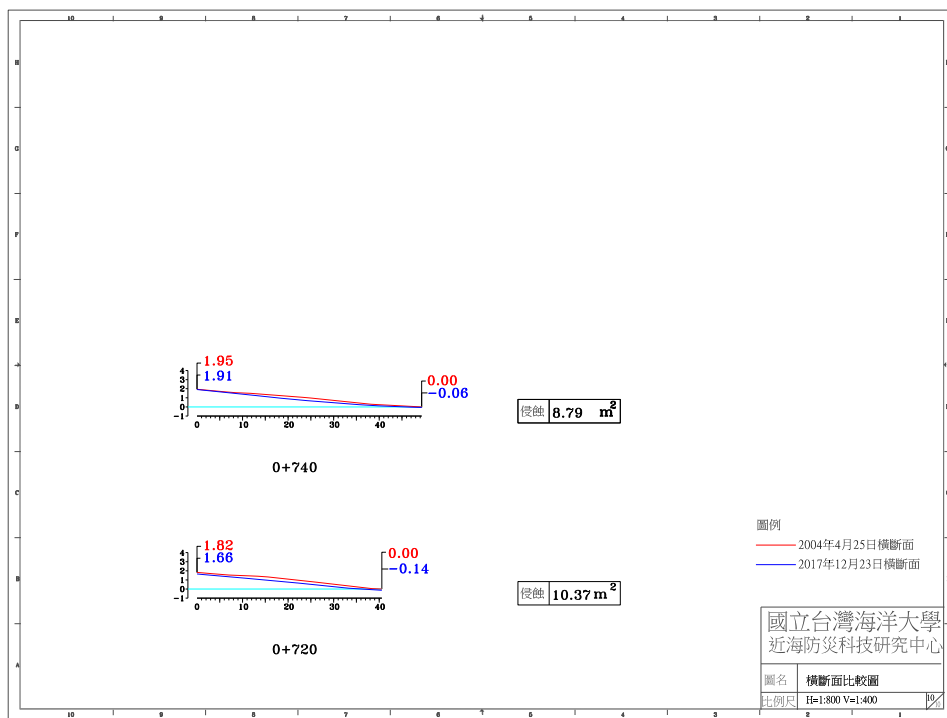
圖 4-4(a) 2017 年 12 月 23 日 A 監測區橫斷面比較圖
