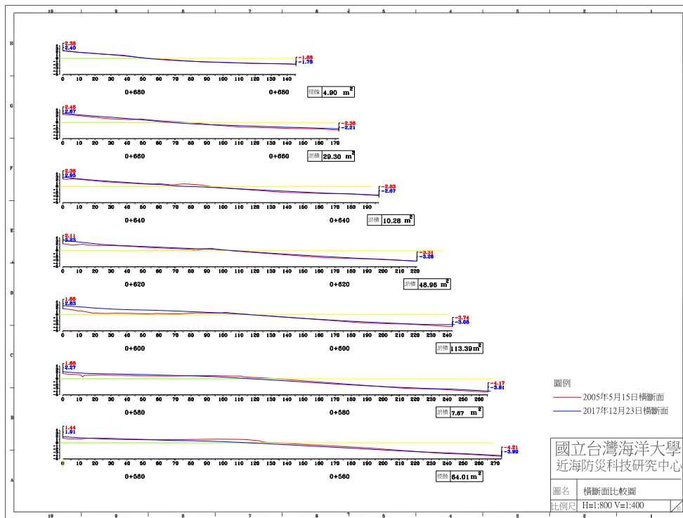
圖 4-5(b) 2017 年 12 月 23 日 B 監測區橫斷面比較圖
