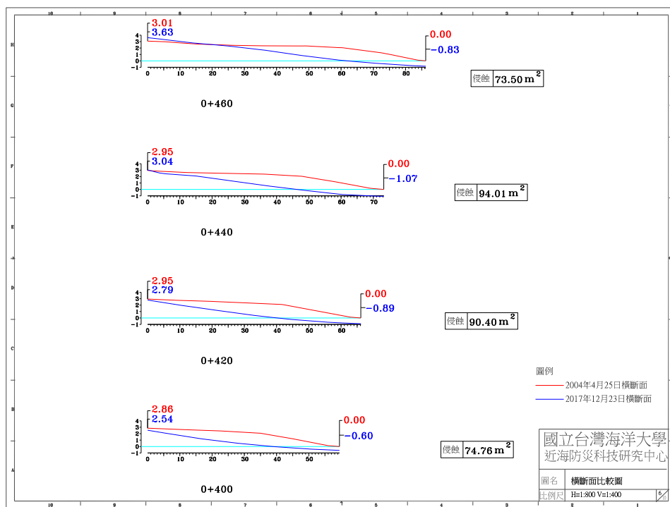
圖 4-4(e) 2017 年 12 月 23 日 A 監測區橫斷面比較圖
