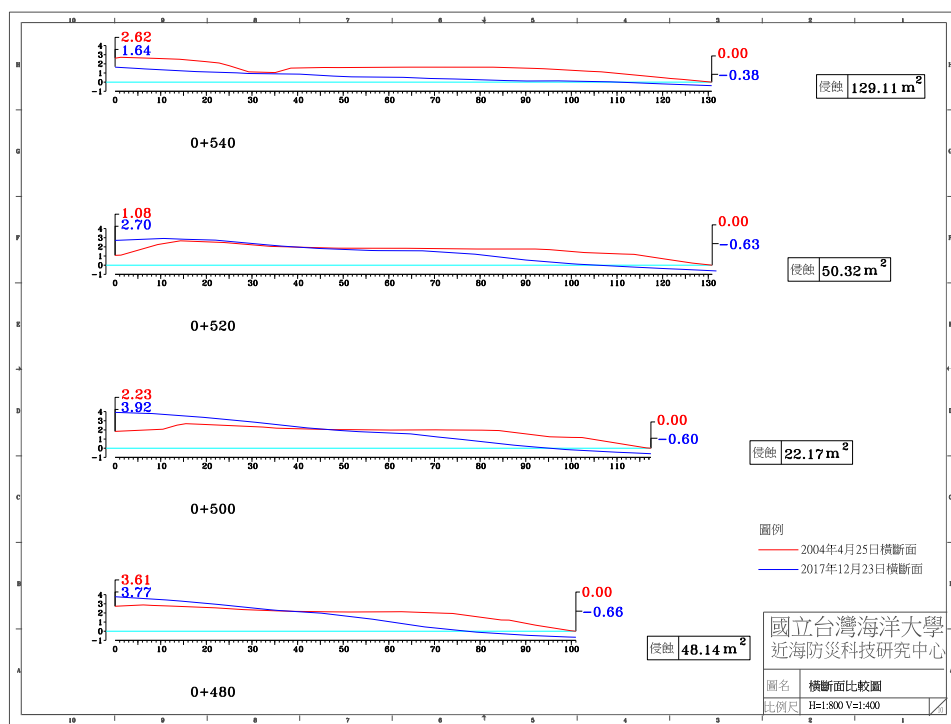
圖 4-4(d) 2017 年 12 月 23 日 A 監測區橫斷面比較圖
