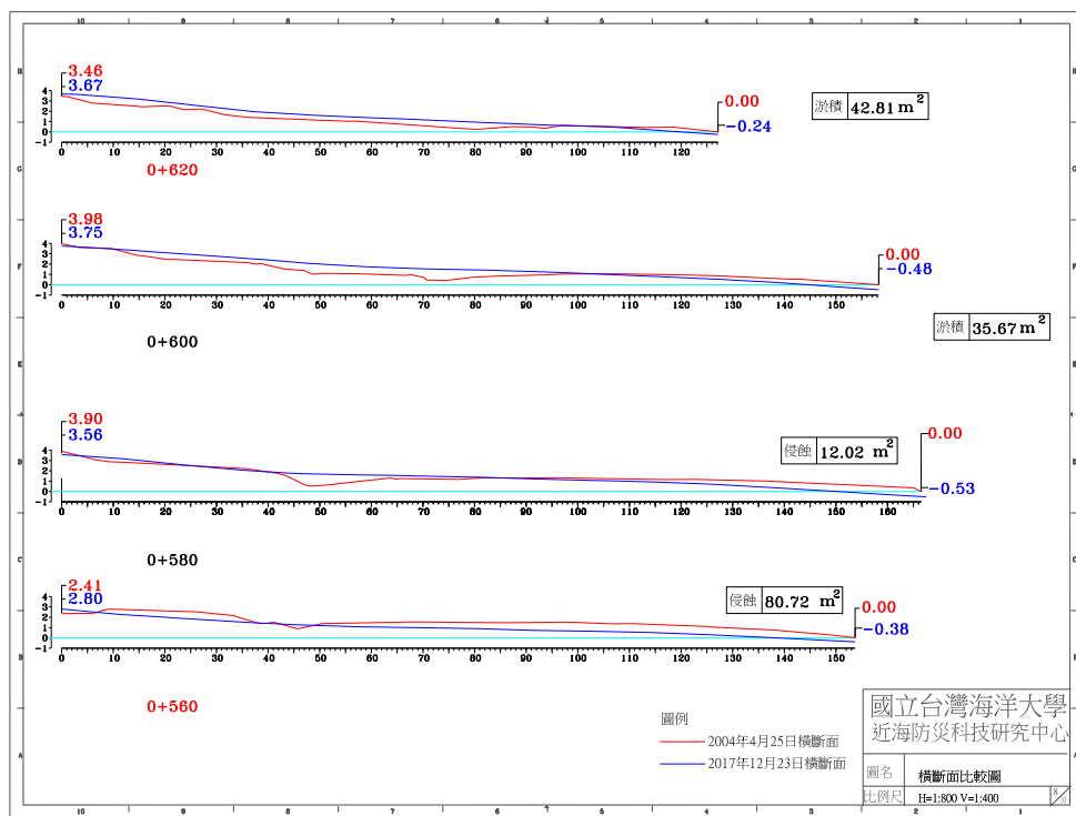
圖 4-4(c) 2017 年 12 月 23 日 A 監測區橫斷面比較圖
