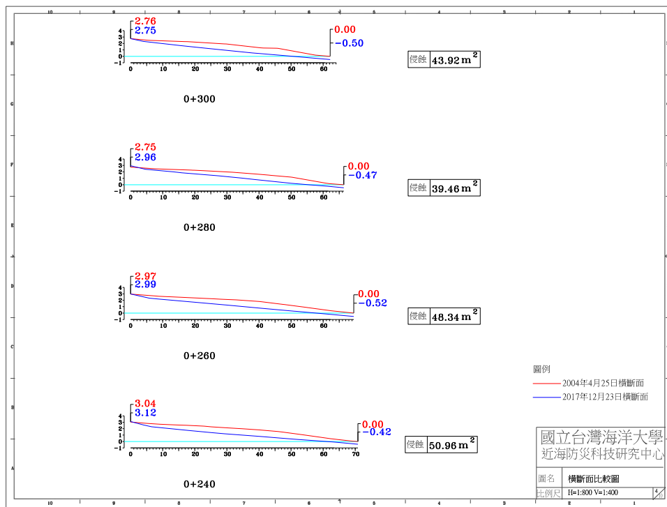
圖 4-4(g) 2017 年 12 月 23 日 A 監測區橫斷面比較圖
