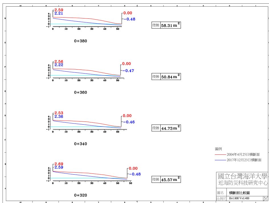
圖 4-4(f) 2017 年 12 月 23 日 A 監測區橫斷面比較圖
