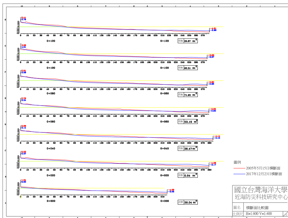
圖 4-5(f) 2017 年 12 月 23 日 B 監測區橫斷面比較圖
