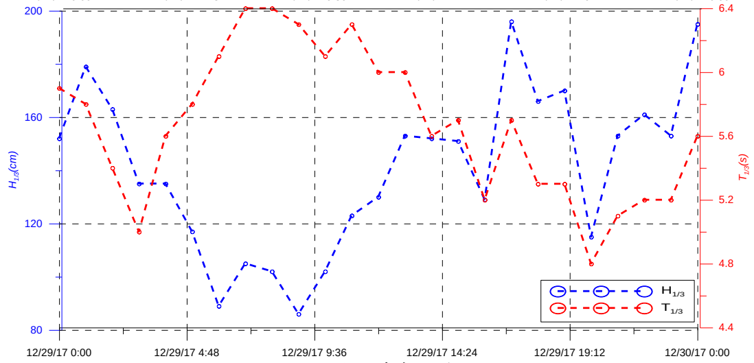
圖 2-3 波浪時序列變化圖
