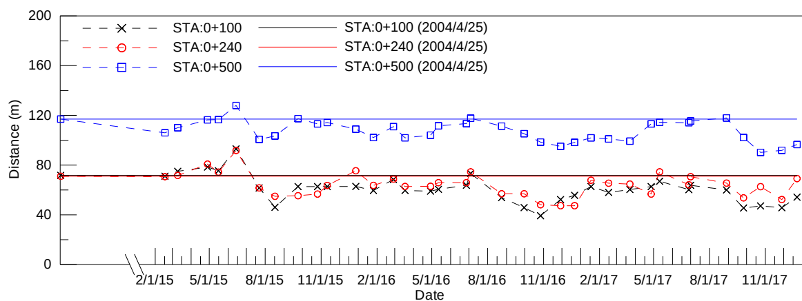
圖 4-21 岸線斷面沙灘寬度變化圖(斷面編號：0+100、0+240、0+500)
