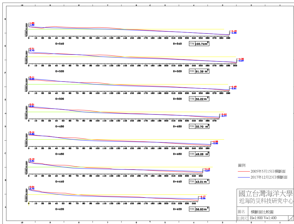
圖 4-5(c) 2017 年 12 月 23 日 B 監測區橫斷面比較圖
