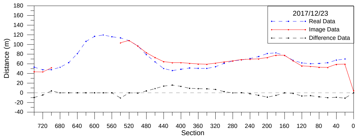
圖 3-23 海岸線分析比較圖(2017/12/23)
