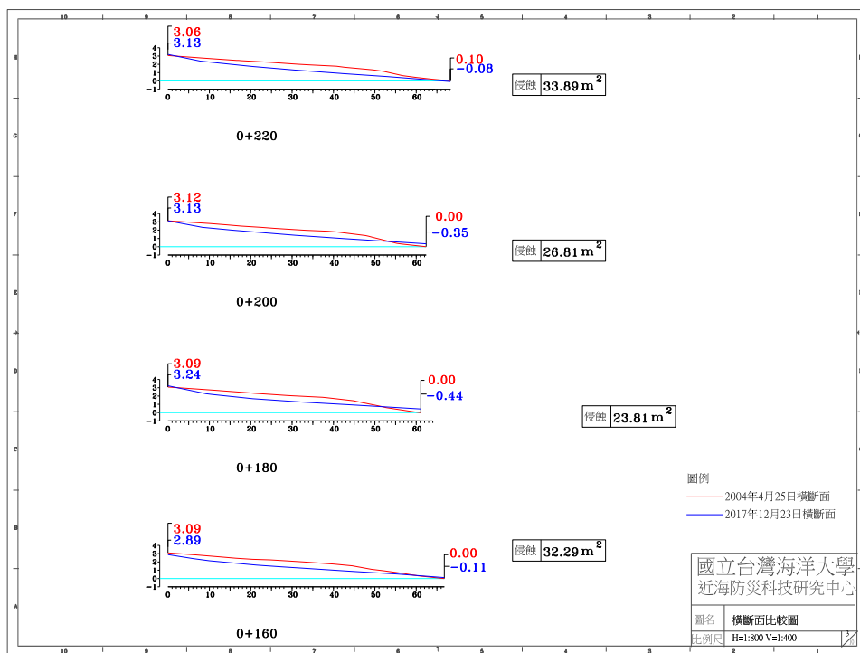
圖 4-4(h) 2017 年 12 月 23 日 A 監測區橫斷面比較圖
