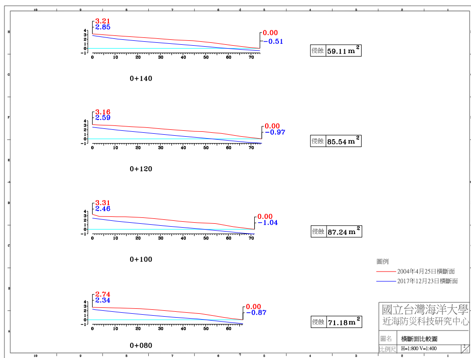
圖 4-4(i) 2017 年 12 月 23 日 A 監測區橫斷面比較圖
