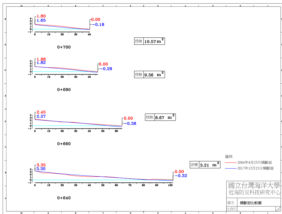
圖 4-4(b) 2017 年 12 月 23 日 A 監測區橫斷面比較圖
