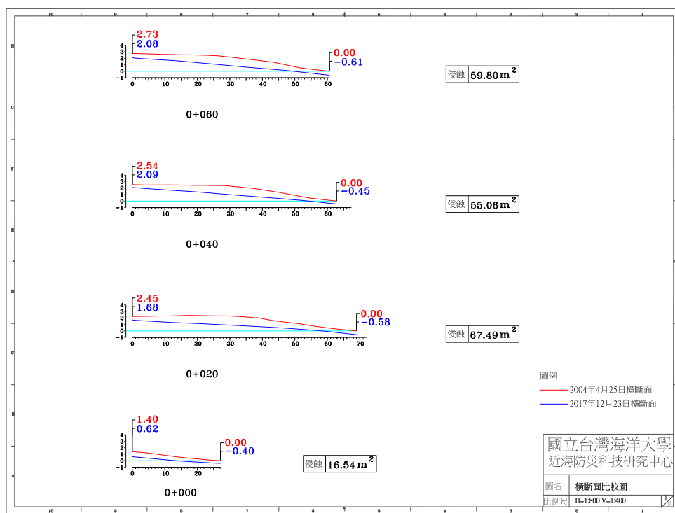
圖 4-4(j) 2017 年 12 月 23 日 A 監測區橫斷面比較圖
