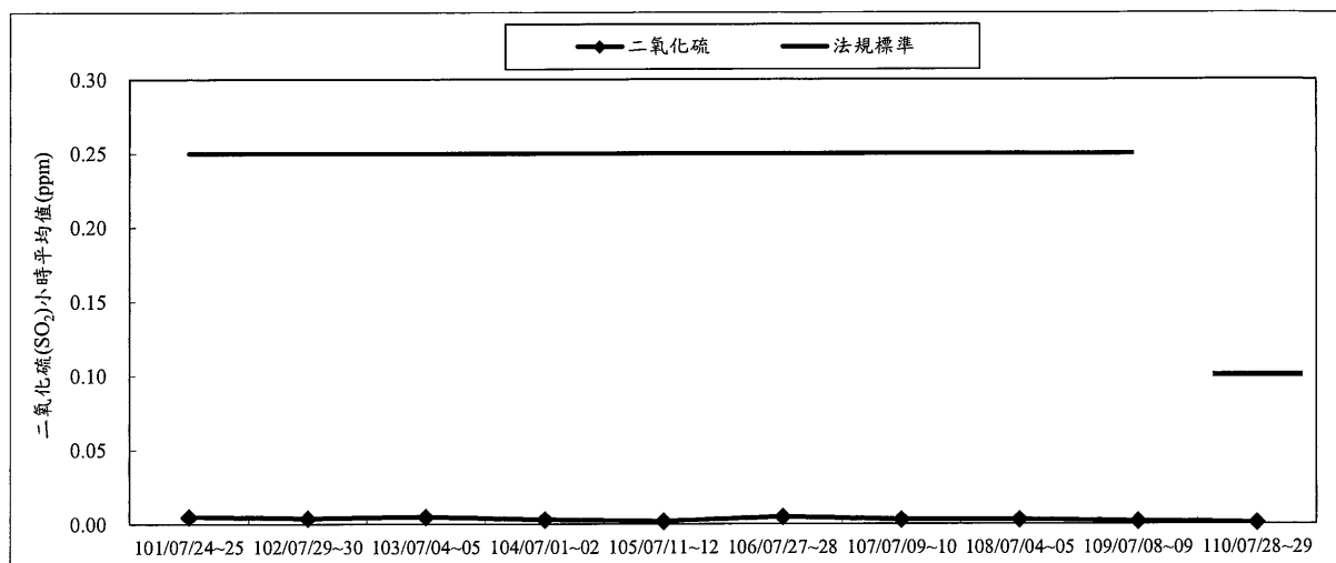
圖 3.1-6 歷年同期二氧化硫(SO 2 )小時平均值監測成果彙整
