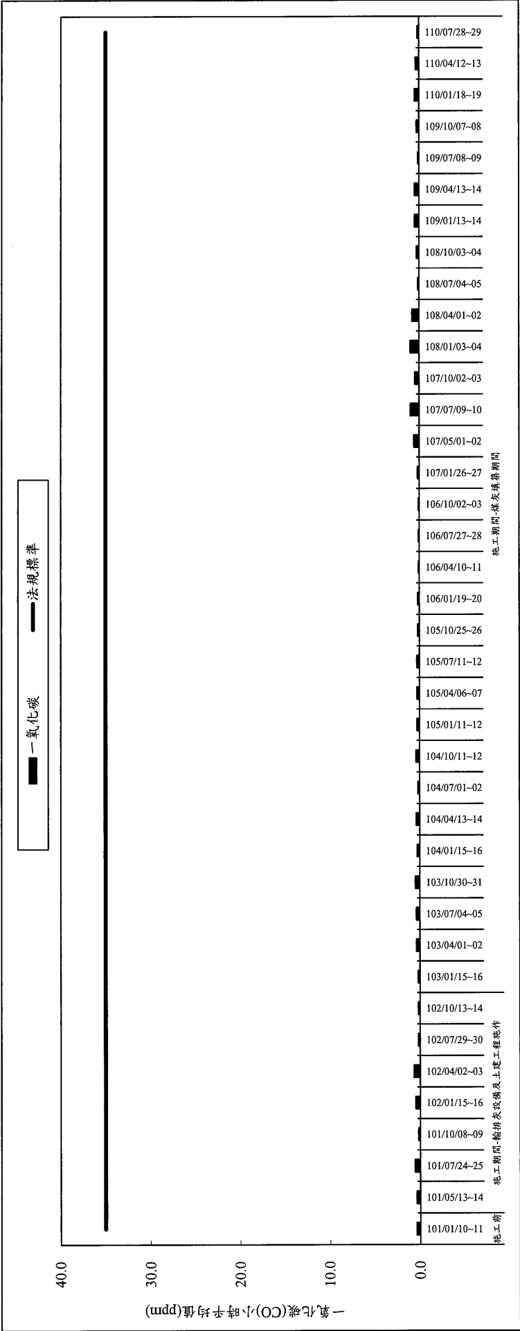
圖 2.1-6 歷季一氧化碳(CO)小時平均濃度監測成果彙整
