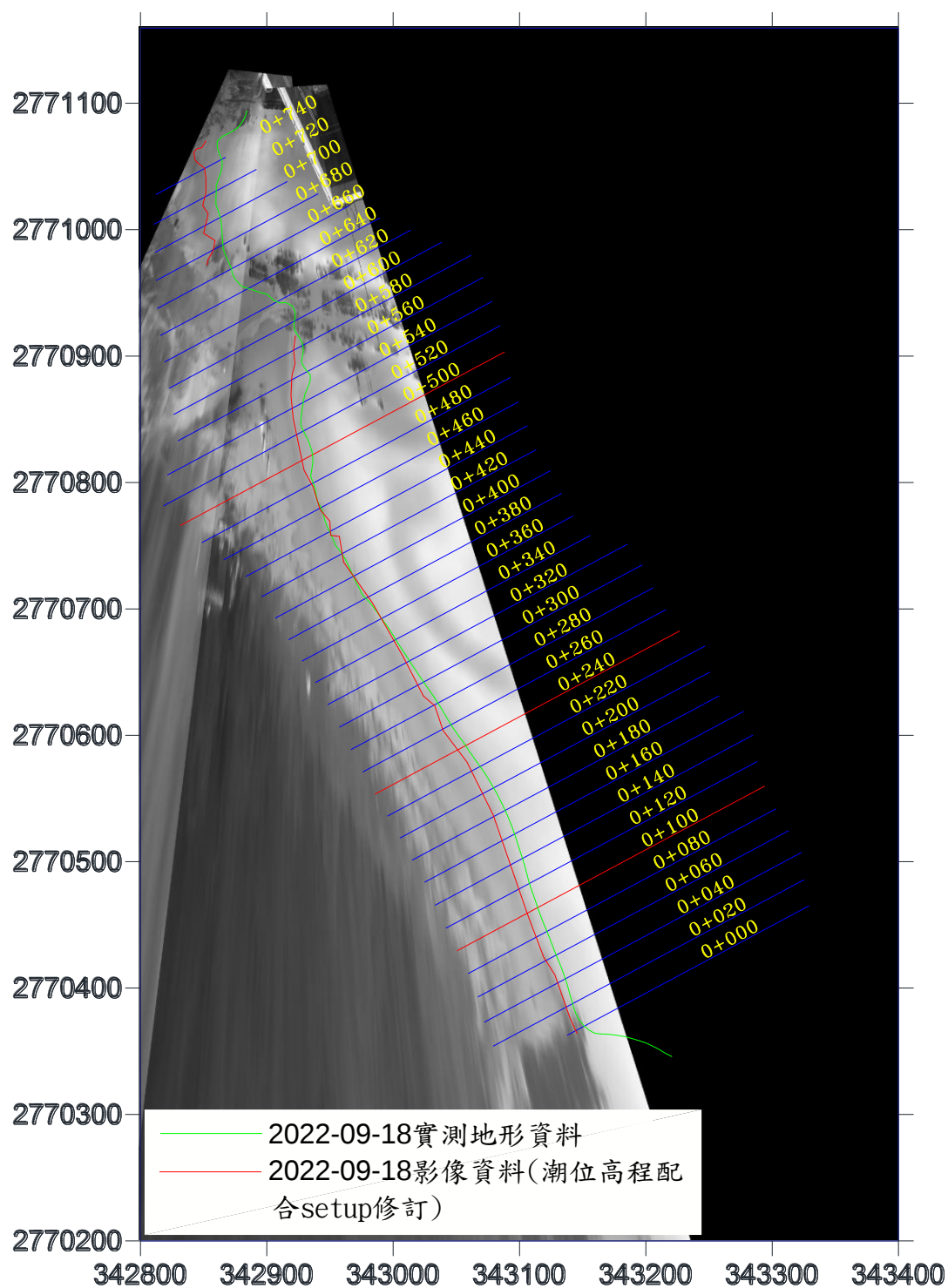
圖 3-22 水位線分析結果圖(2022/09/18)
