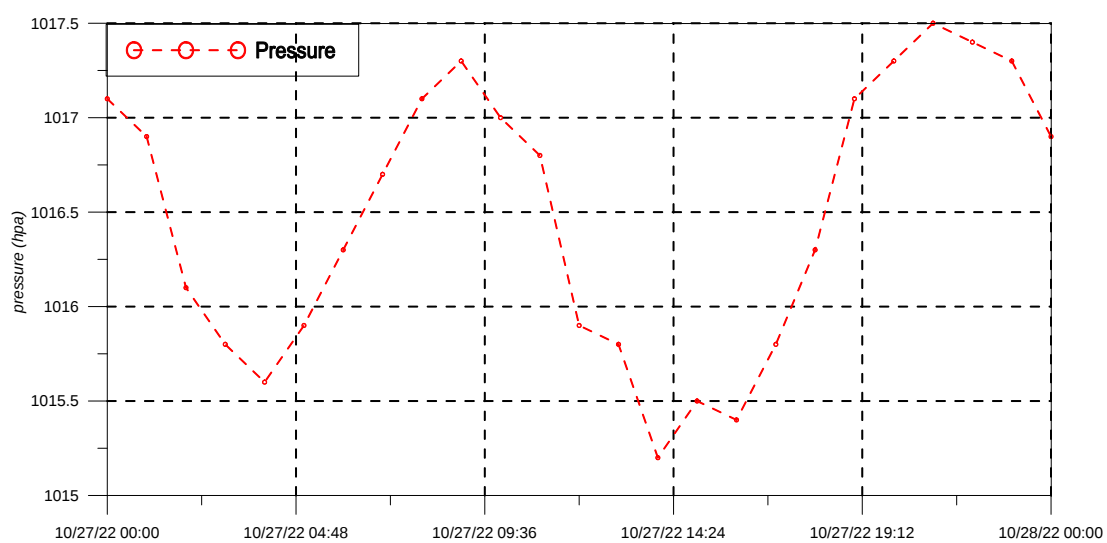
圖 2-5 壓力時序列變化圖
