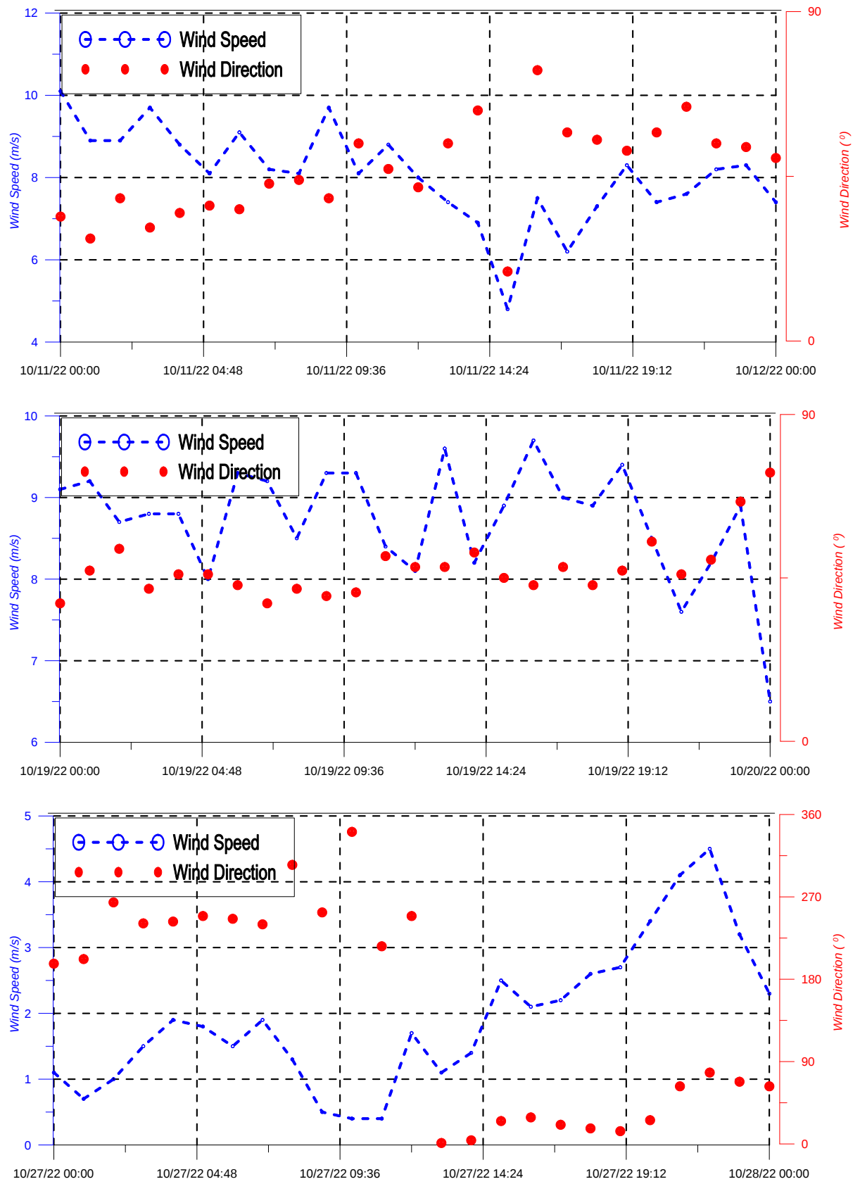
圖 2-2 風速風向時序列變化圖
