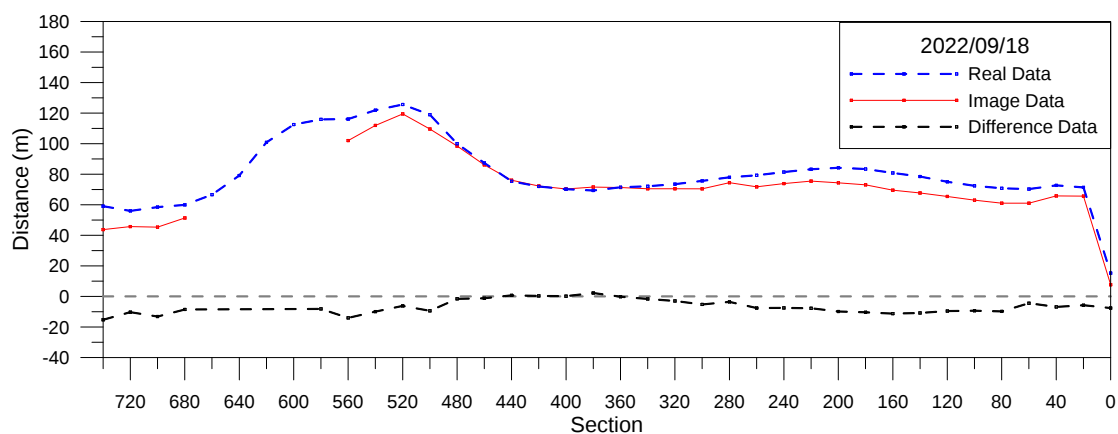
圖 3-23 海岸線分析比較圖(2022/09/18)
