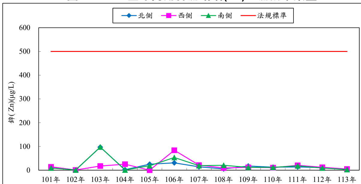
圖 3.1-17 歷年同期各測站鋅(Zn)監測成果彙整
