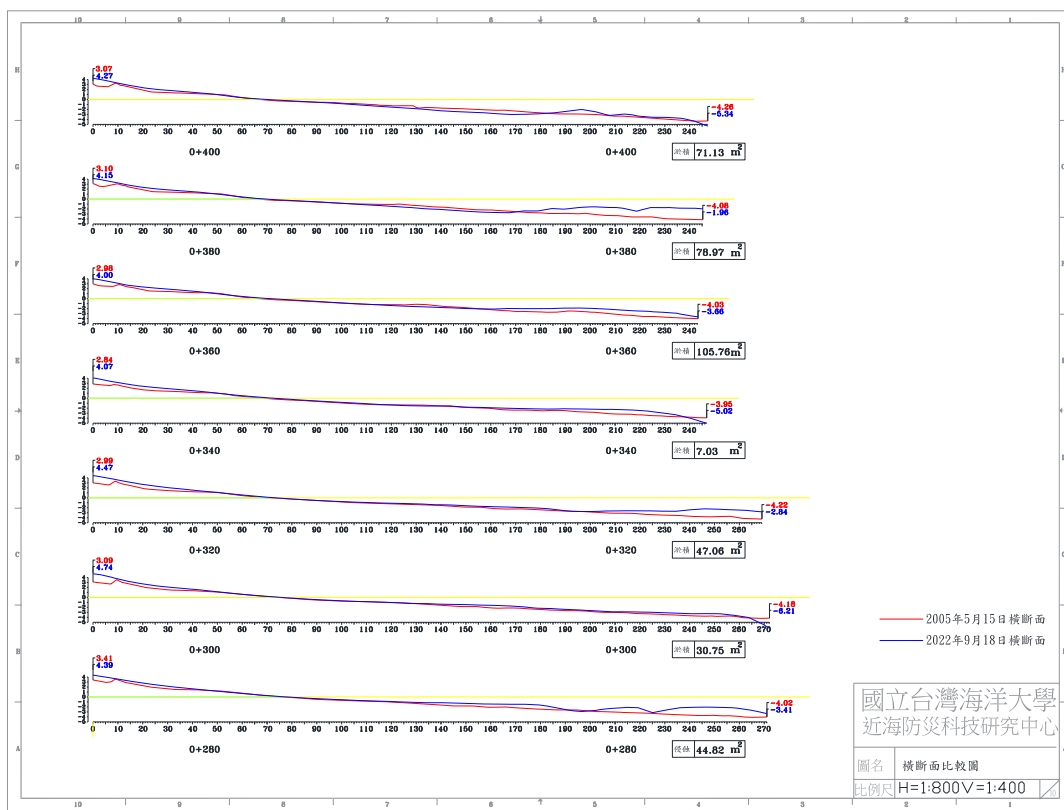
圖 4-5(d) 2022 年 9 月 18 日 B 監測區橫斷面比較圖
