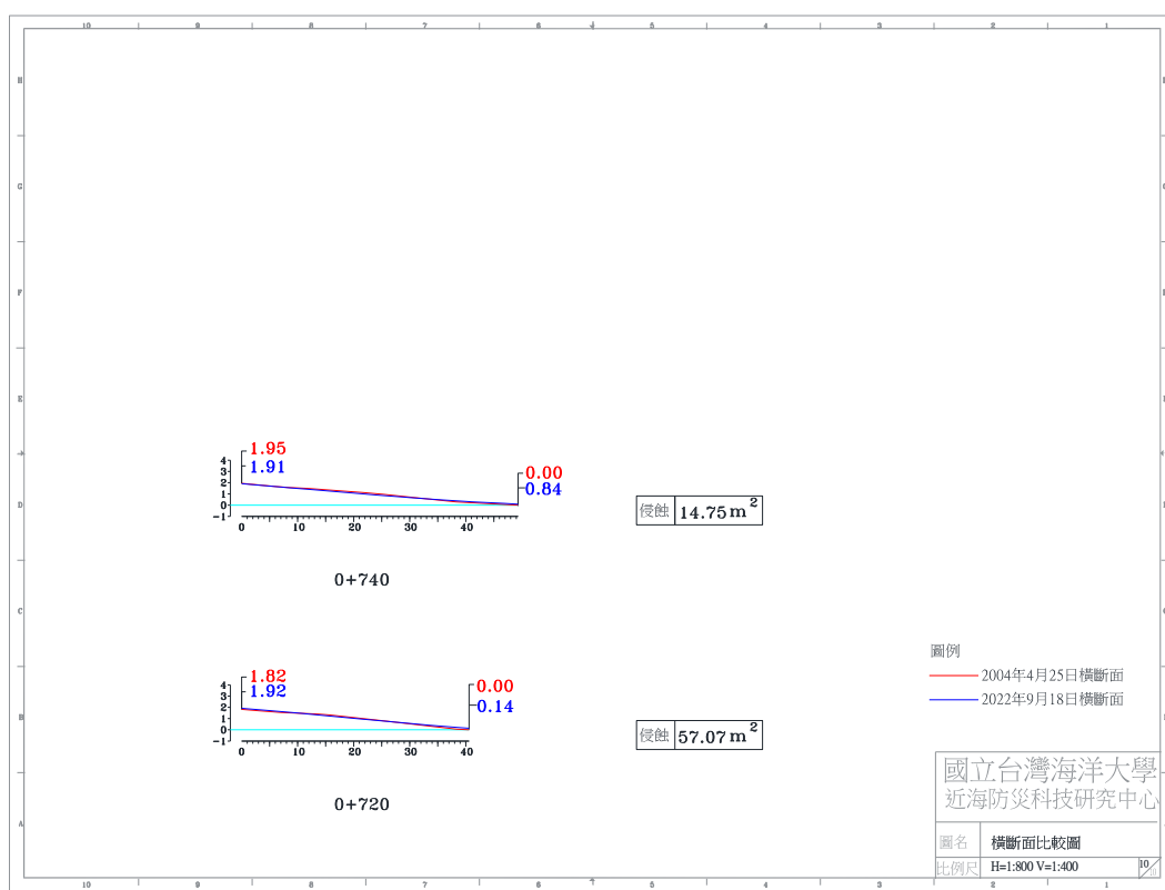
圖 4-4(a) 2022 年 9 月 18 日 A 監測區橫斷面比較圖
