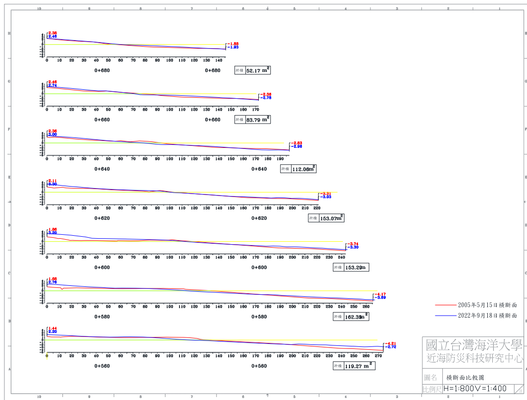
圖 4-5(b) 2022 年 9 月 18 日 B 監測區橫斷面比較圖
