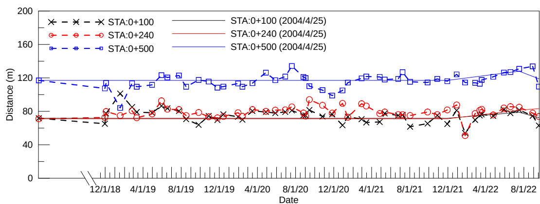
圖 4-21 岸線斷面沙灘寬度變化圖(2022/9/18)
