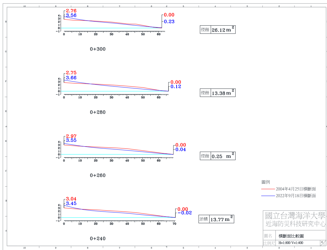
圖 4-4(g) 2022 年 9 月 18 日 A 監測區橫斷面比較圖
