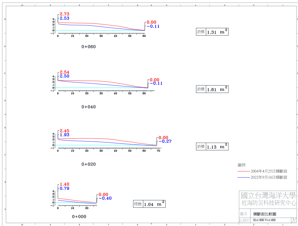
圖 4-4(j) 2022 年 9 月 18 日 A 監測區橫斷面比較圖
