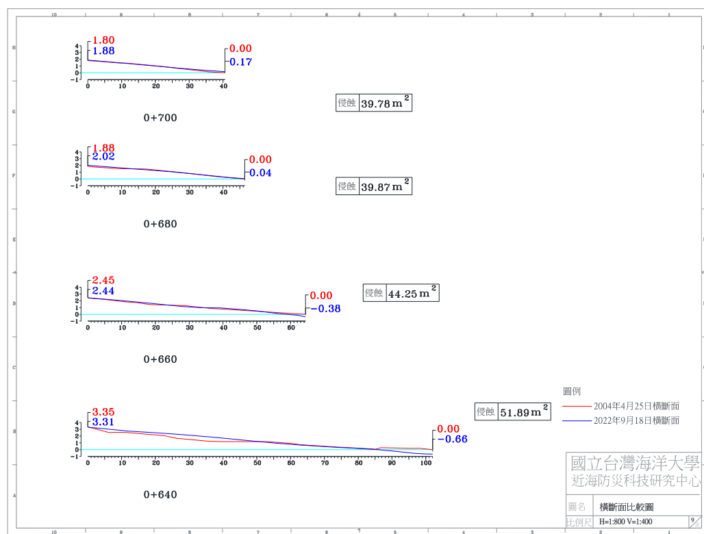
圖 4-4(b) 2022 年 9 月 18 日 A 監測區橫斷面比較圖
