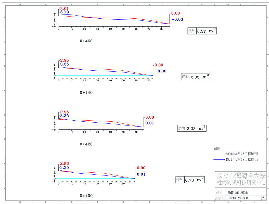
圖 4-4(e) 2022 年 9 月 18 日 A 監測區橫斷面比較圖
