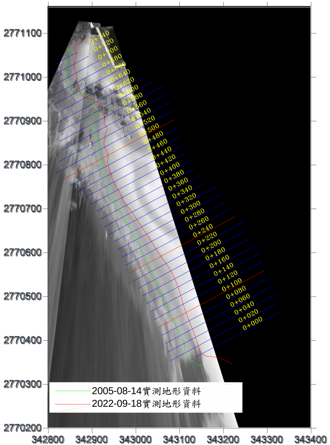
圖 4-22 長期實測 0 m 灘線比對平面示意圖(2022/09/18)
