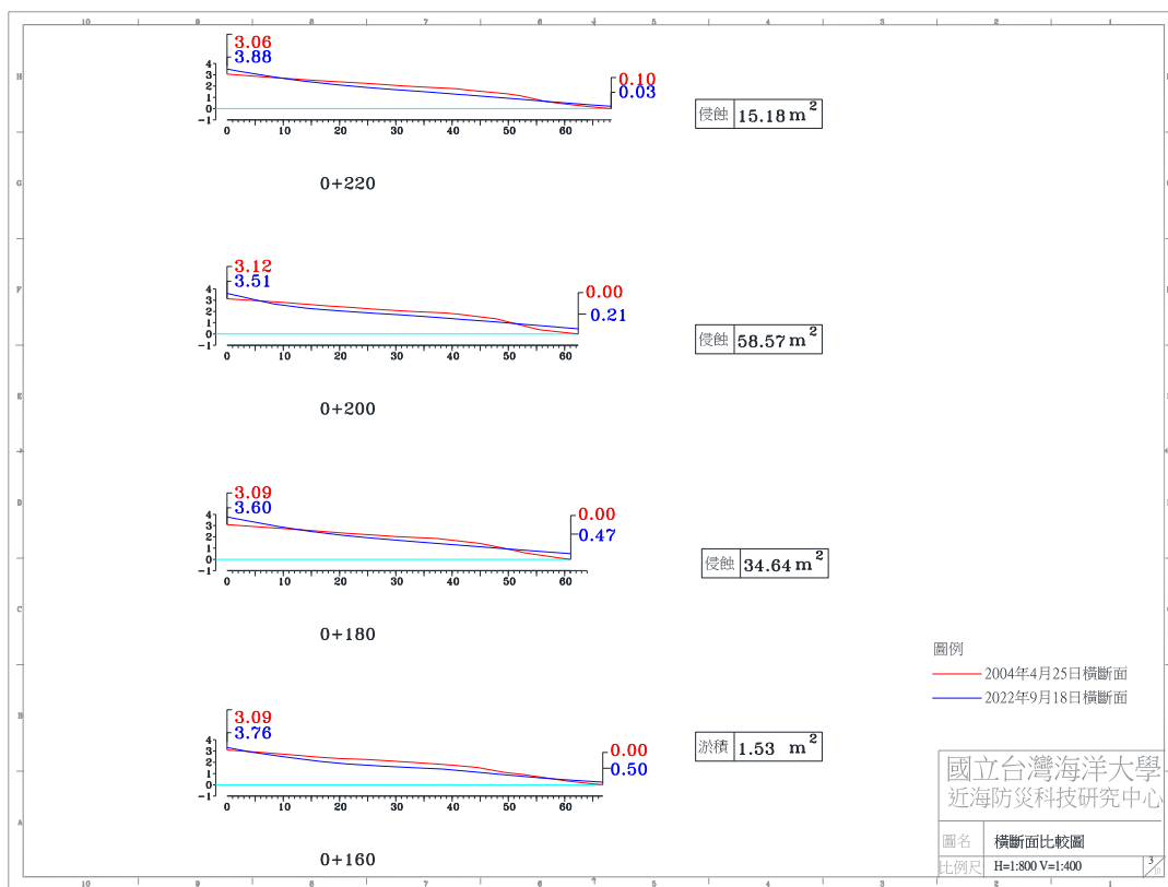
圖 4-4(h) 2022 年 9 月 18 日 A 監測區橫斷面比較圖
