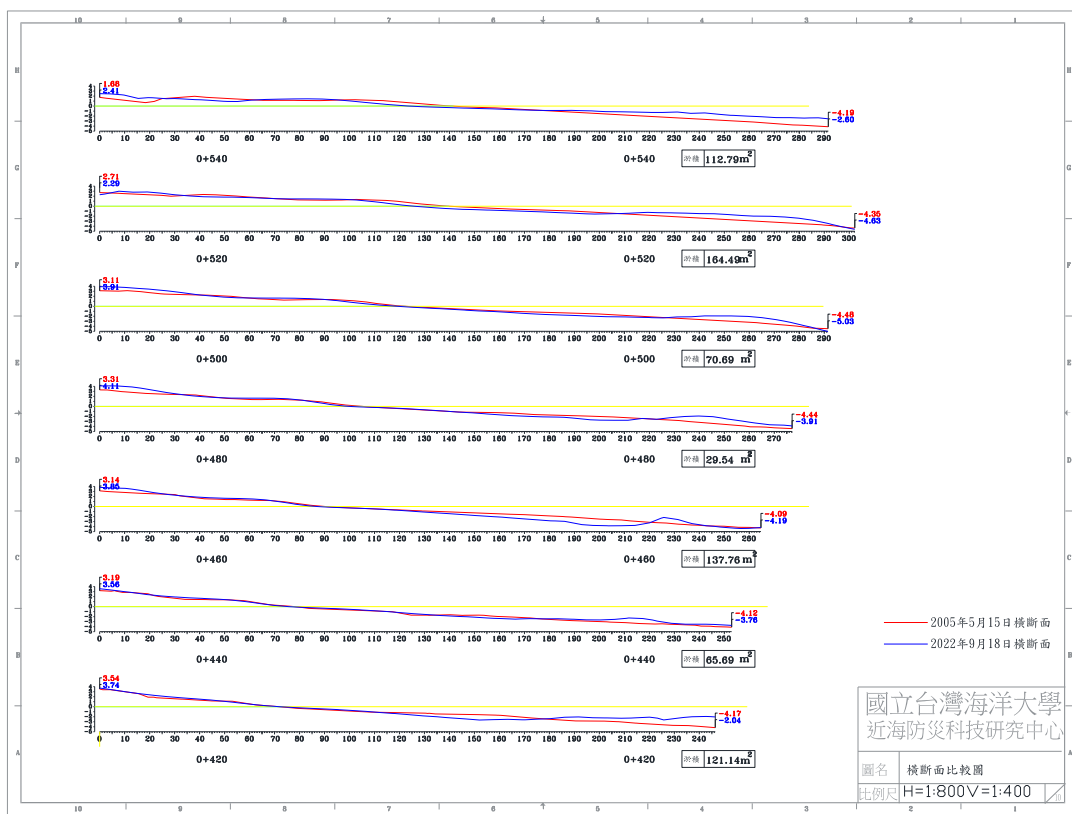
圖 4-5(c) 2022 年 9 月 18 日 B 監測區橫斷面比較圖
