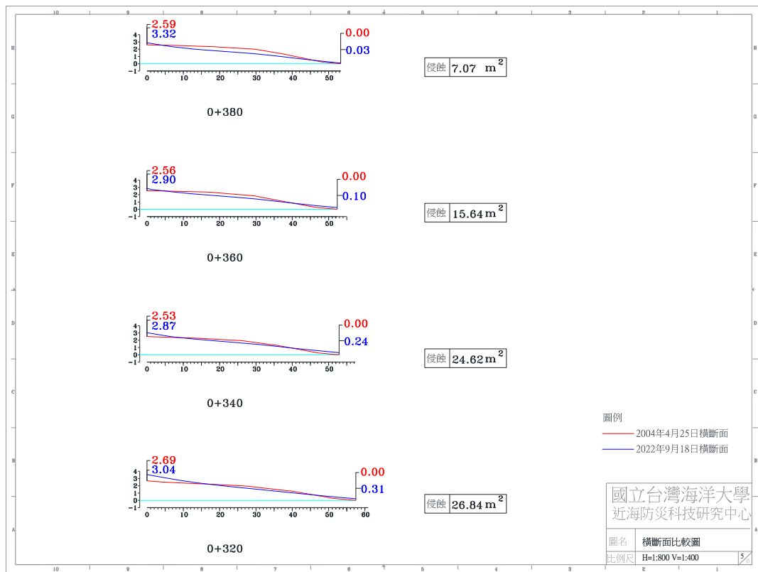
圖 4-4(f) 2022 年 9 月 18 日 A 監測區橫斷面比較圖
