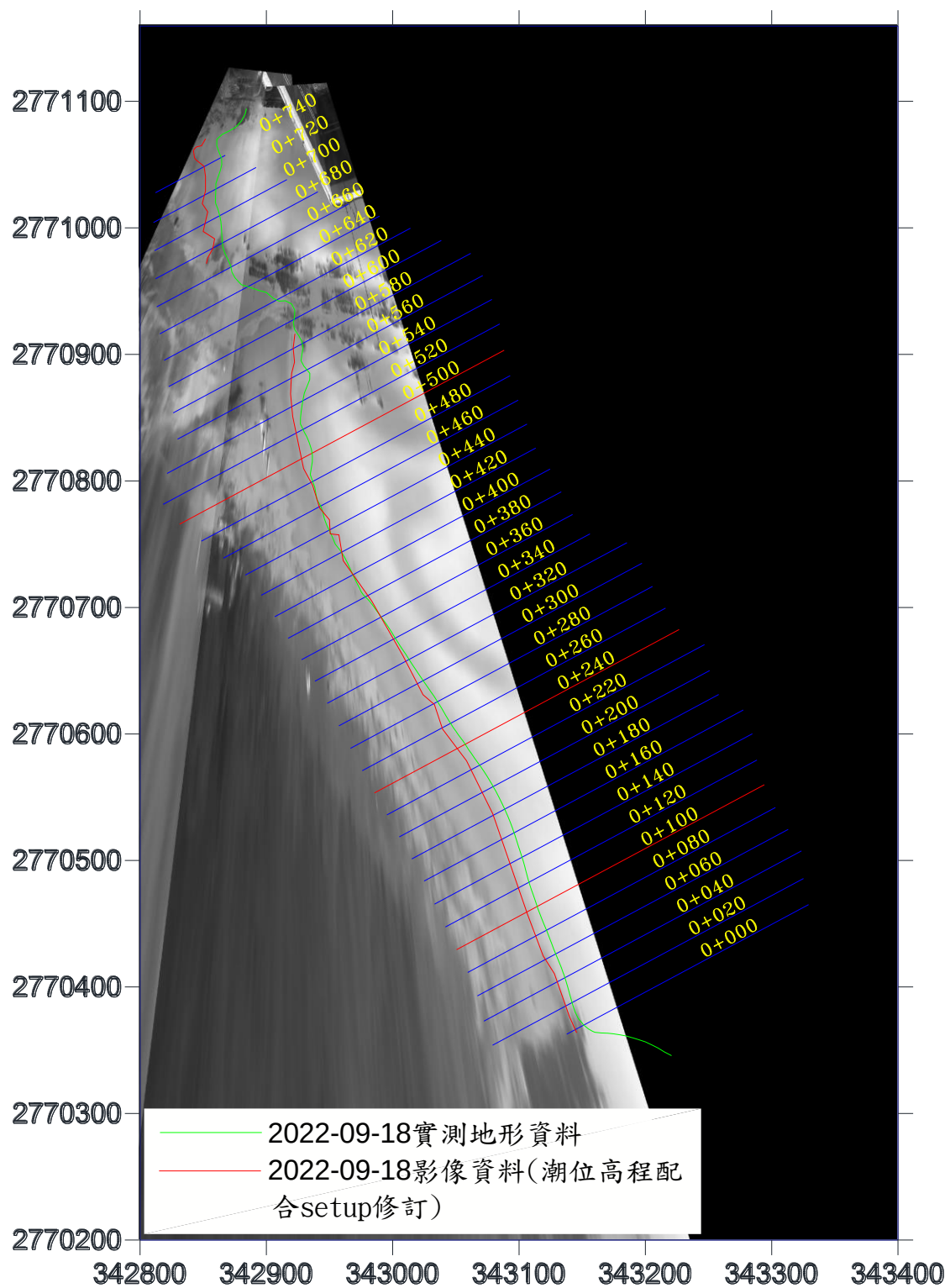
圖 3-22 水位線分析結果圖(2022/09/18)
