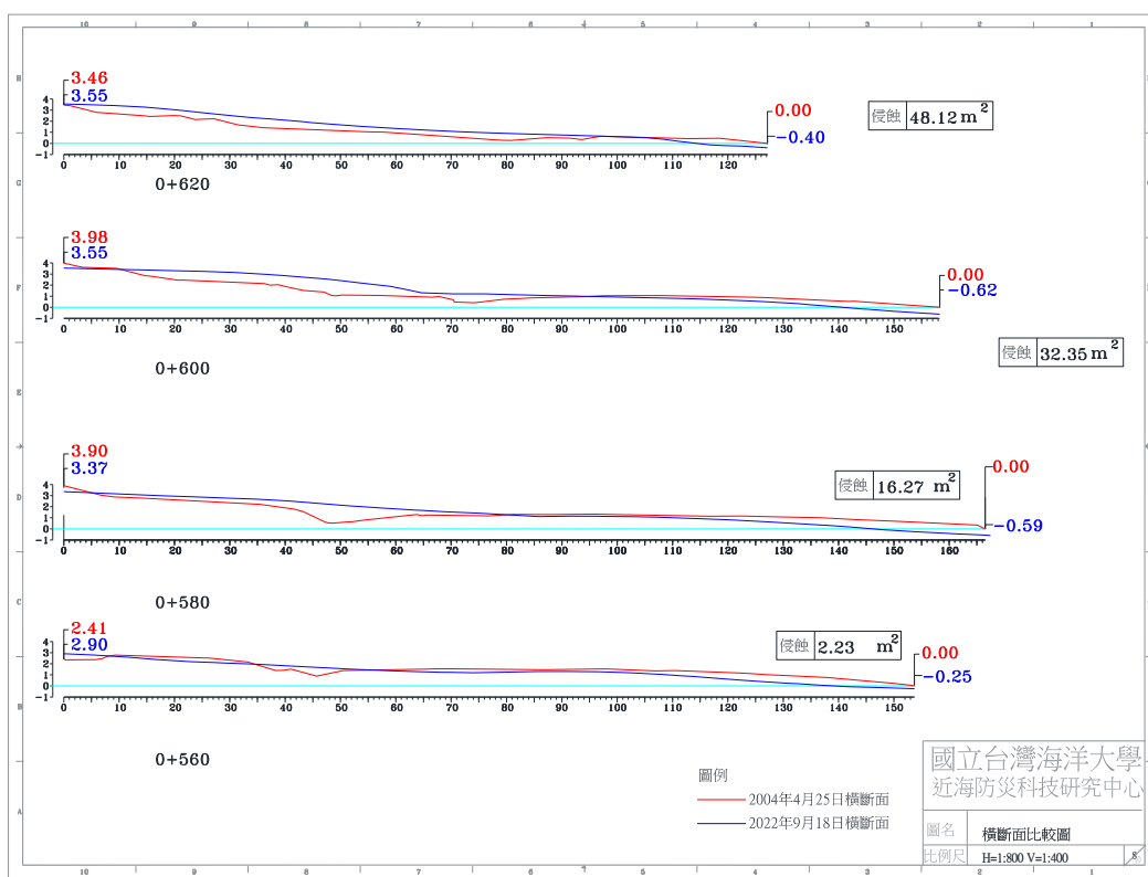
圖 4-4(c) 2022 年 9 月 18 日 A 監測區橫斷面比較圖
