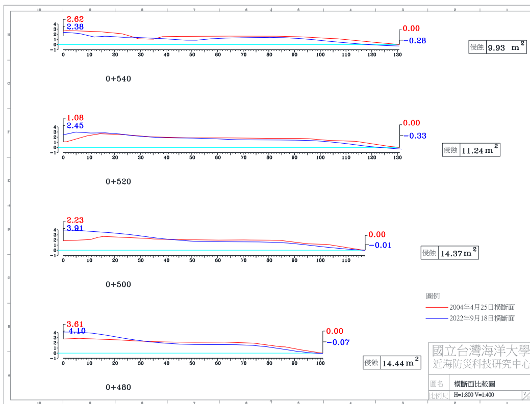
圖 4-4(d) 2022 年 9 月 18 日 A 監測區橫斷面比較圖
