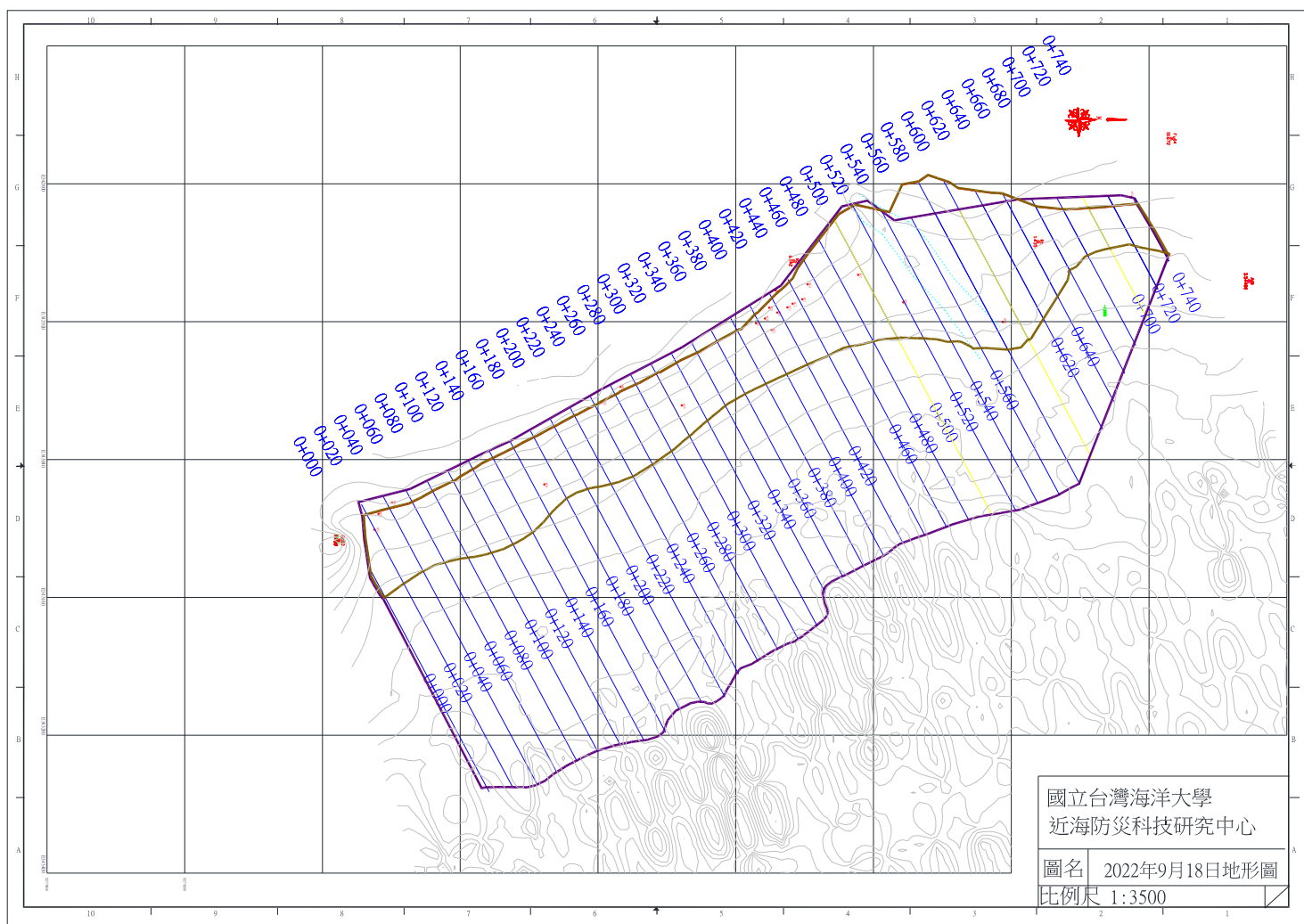
圖 4-1 2022 年 9 月 18 日監測地形
