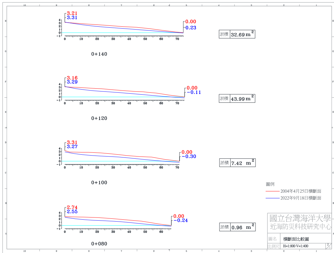
圖 4-4(i) 2022 年 9 月 18 日 A 監測區橫斷面比較圖
