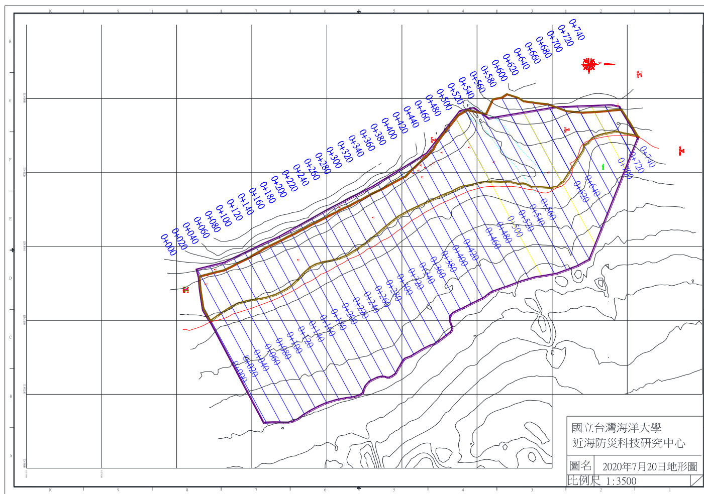
圖 4-1 2020 年 7 月 20 日監測地形圖
