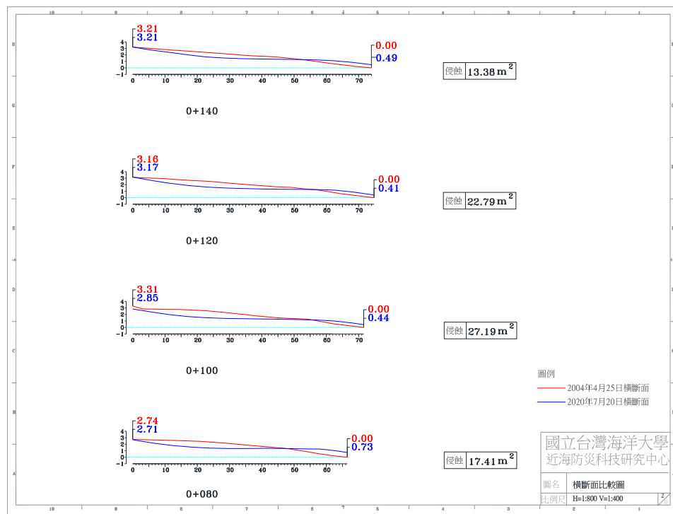
圖 4-4(i) 2020 年 7 月 20 日 A 監測區橫斷面比較圖
