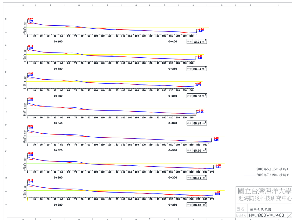
圖 4-5(d) 2020 年 7 月 20 日 B 監測區橫斷面比較圖
