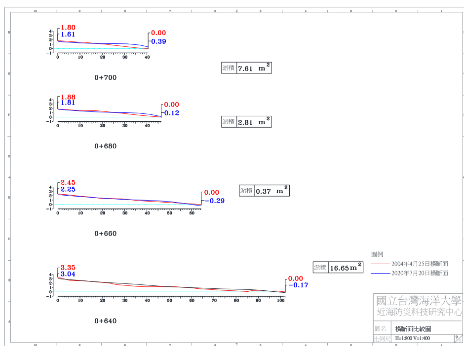
圖 4-4(b) 2020 年 7 月 20 日 A 監測區橫斷面比較圖
