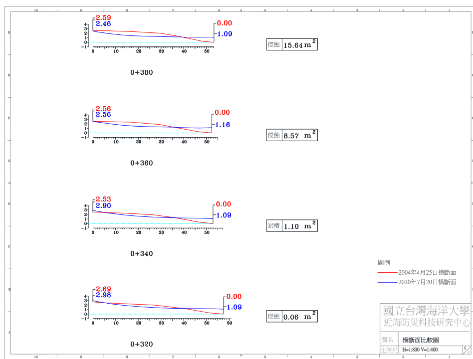
圖 4-4(f) 2020 年 7 月 20 日 A 監測區橫斷面比較圖
