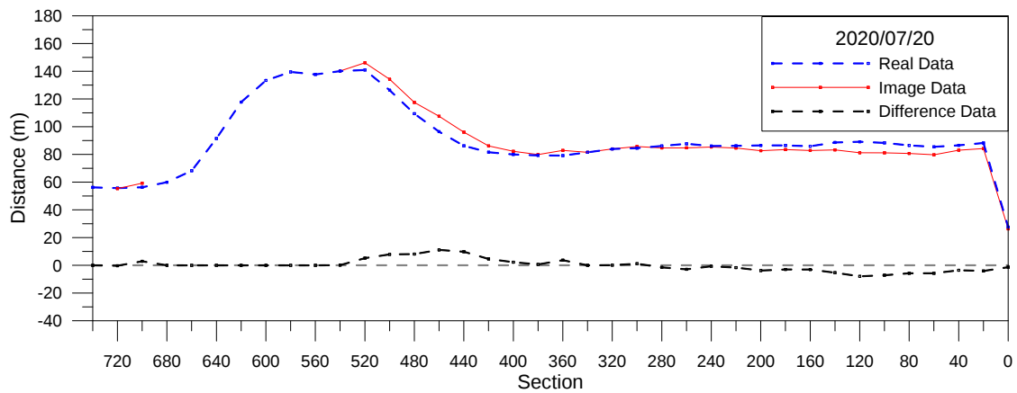
圖 3-23 海岸線分析比較圖(2020/7/20)
