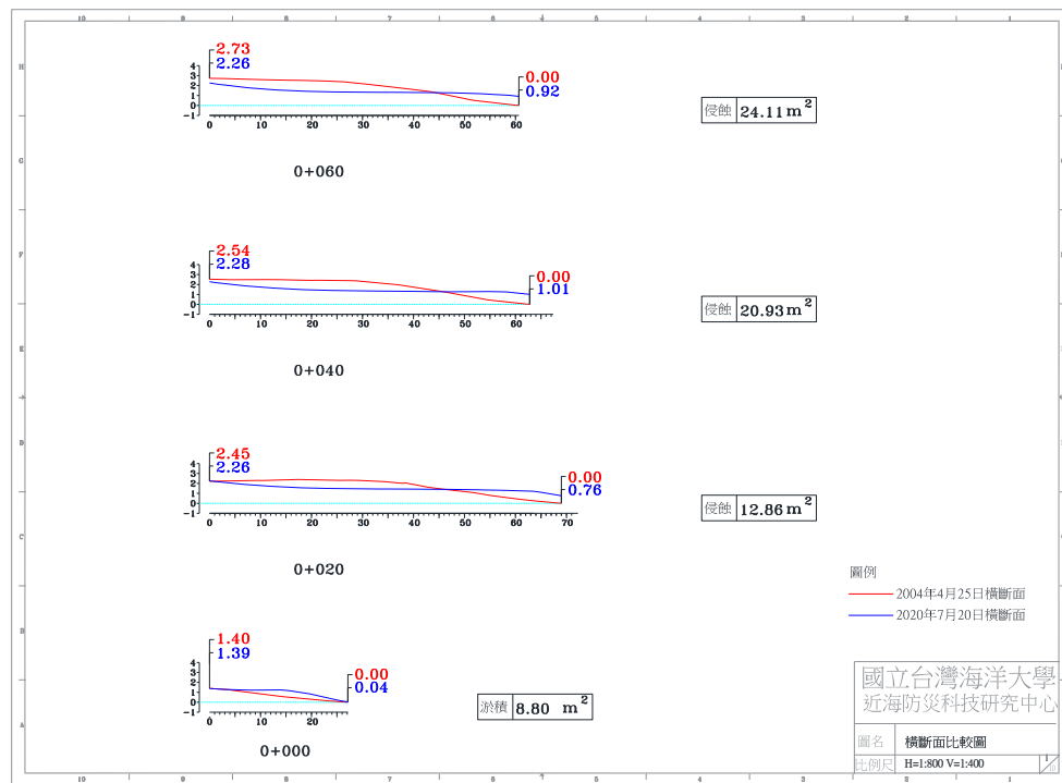
圖 4-4(j) 2020 年 7 月 20 日 A 監測區橫斷面比較圖
