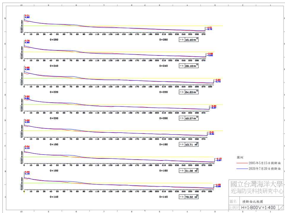
圖 4-5(e) 2020 年 7 月 20 日 B 監測區橫断面比較圖
