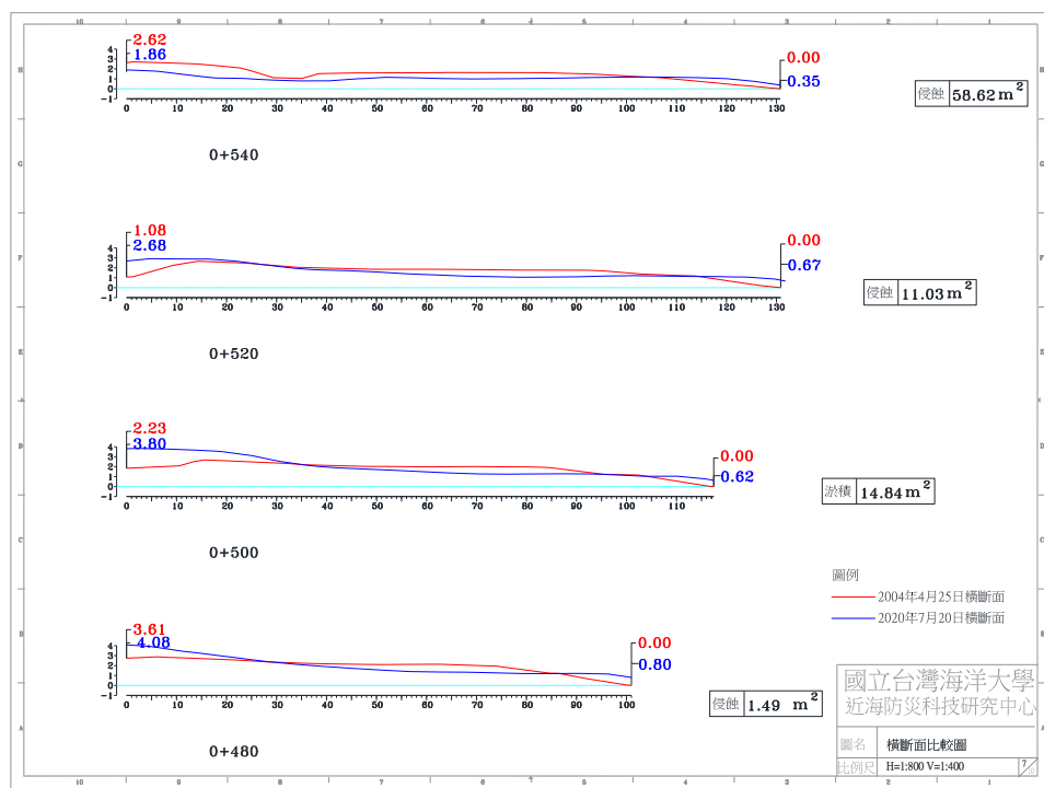
圖 4-4(d) 2020 年 7 月 20 日 A 監測區橫斷面比較圖
