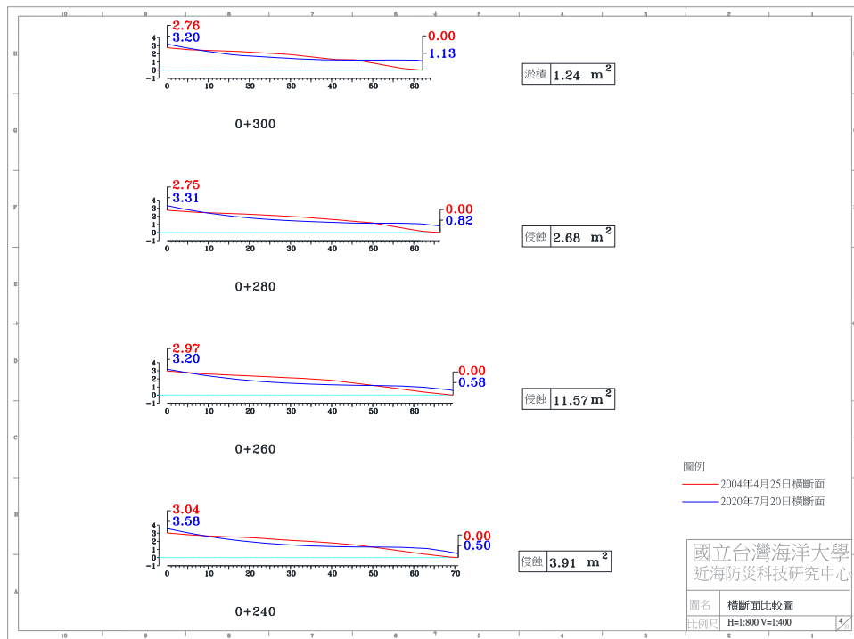
圖 4-4(g) 2020 年 7 月 20 日 A 監測區橫斷面比較圖
