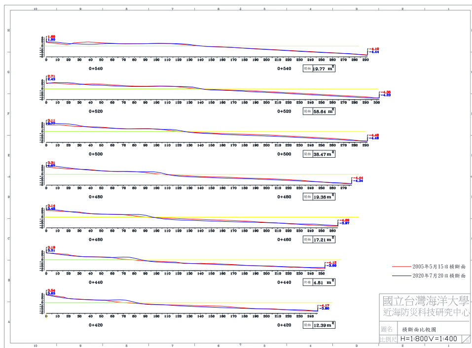
圖 4-5(c) 2020 年 7 月 20 日 B 監測區橫斷面比較圖
