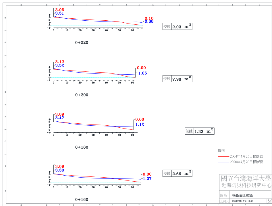
圖 4-4(h) 2020 年 7 月 20 日 A 監測區橫斷面比較圖
