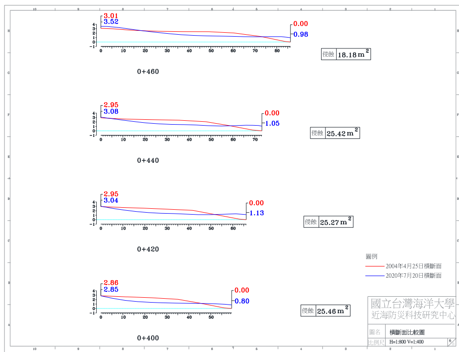
圖 4-4(e) 2020 年 7 月 20 日 A 監測區橫斷面比較圖
