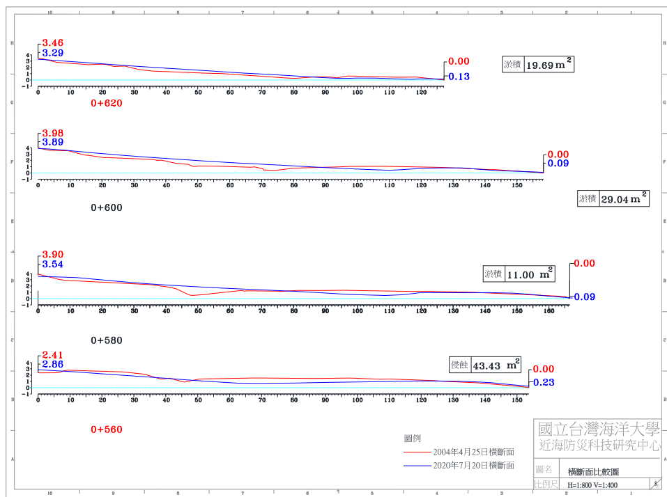
圖 4-4(c) 2020 年 7 月 20 日 A 監測區橫斷面比較圖
