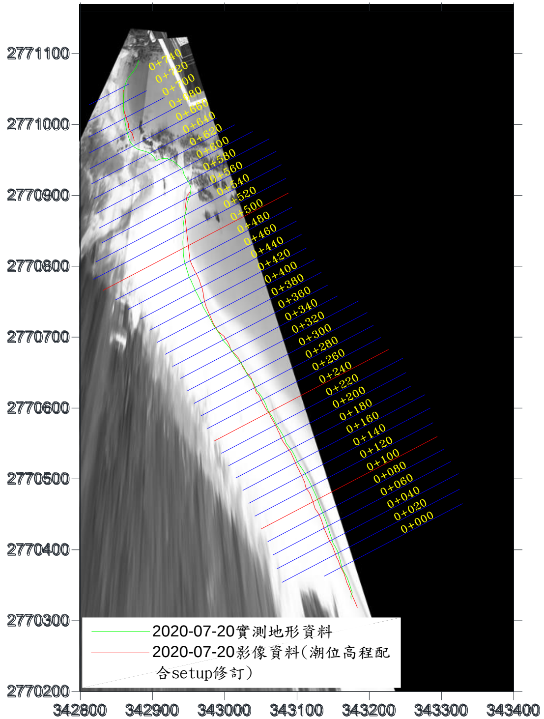
圖 3-22 水位線分析結果圖(2020/7/20)
