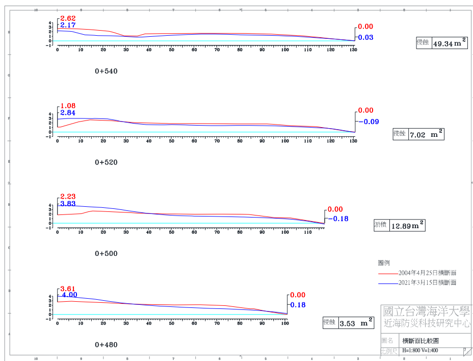
圖 4-4(d) 2021 年 3 月 15 日 A 監測區橫斷面比較圖
