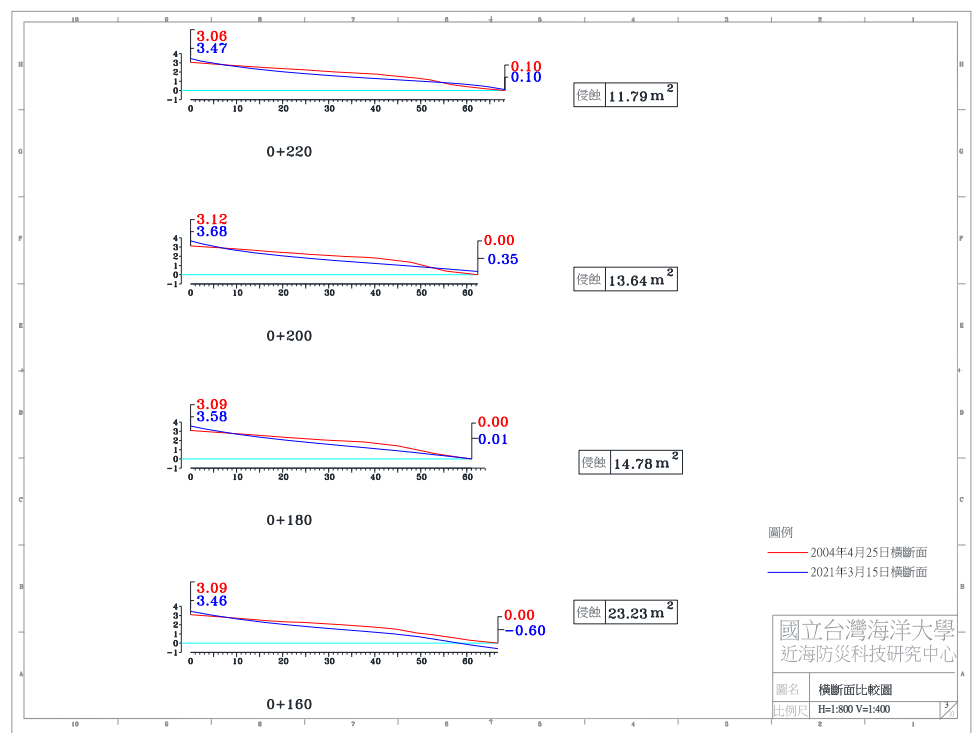
圖 4-4(h) 2021 年 3 月 15 日 A 監測區橫斷面比較圖
