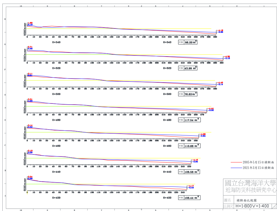
圖 4-5(c) 2021 年 3 月 15 日 B 監測區橫斷面比較圖
