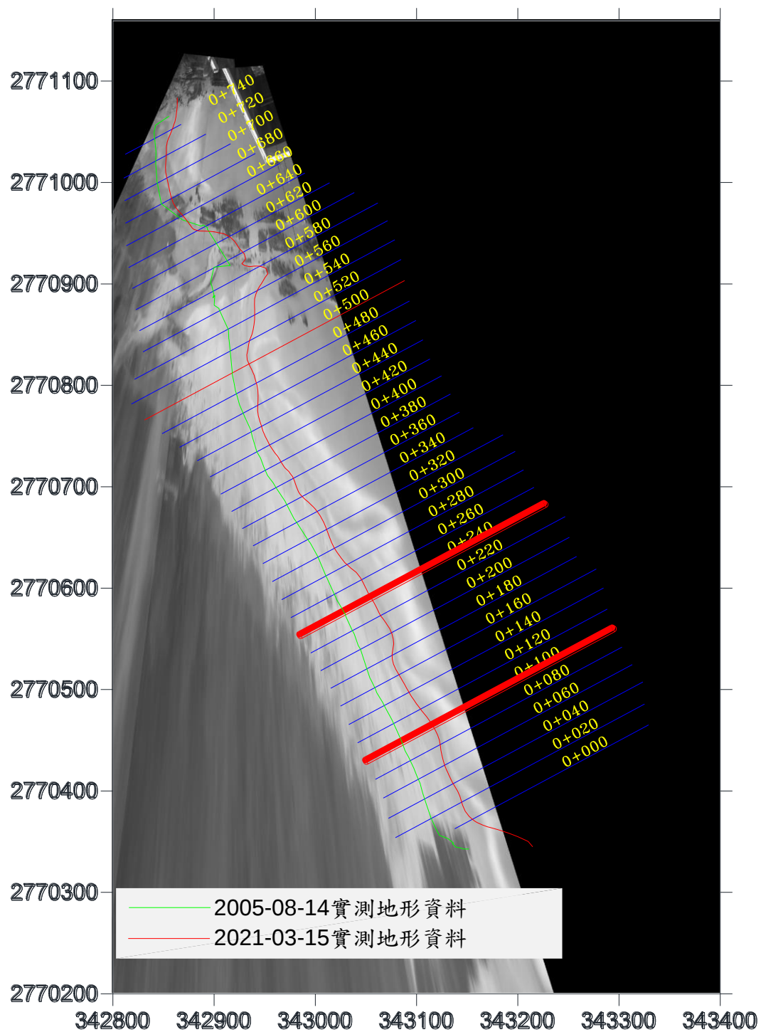
圖 4-22 實測地形水位線分析結果圖(2021/03/15)
