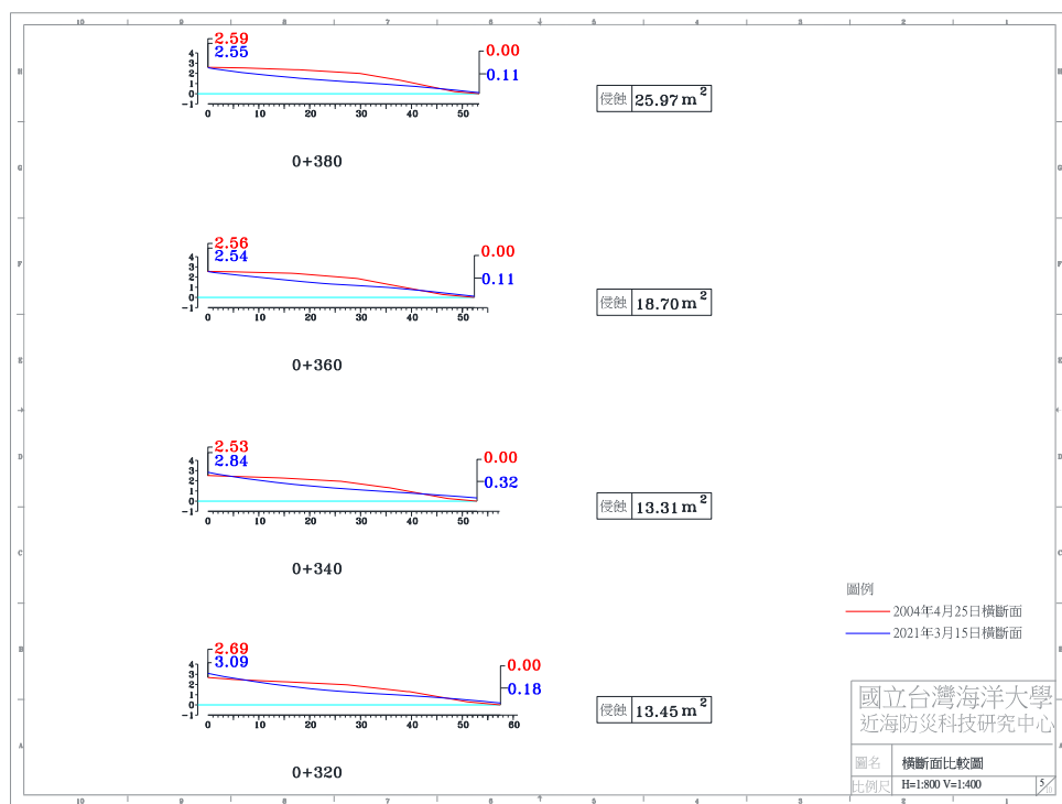
圖 4-4(f) 2021 年 3 月 15 日 A 監測區橫斷面比較圖
