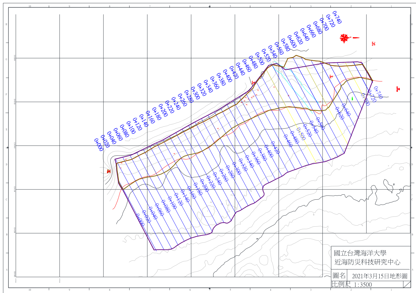
圖 4-1 2021 年 3 月 15 日監測地形圖
