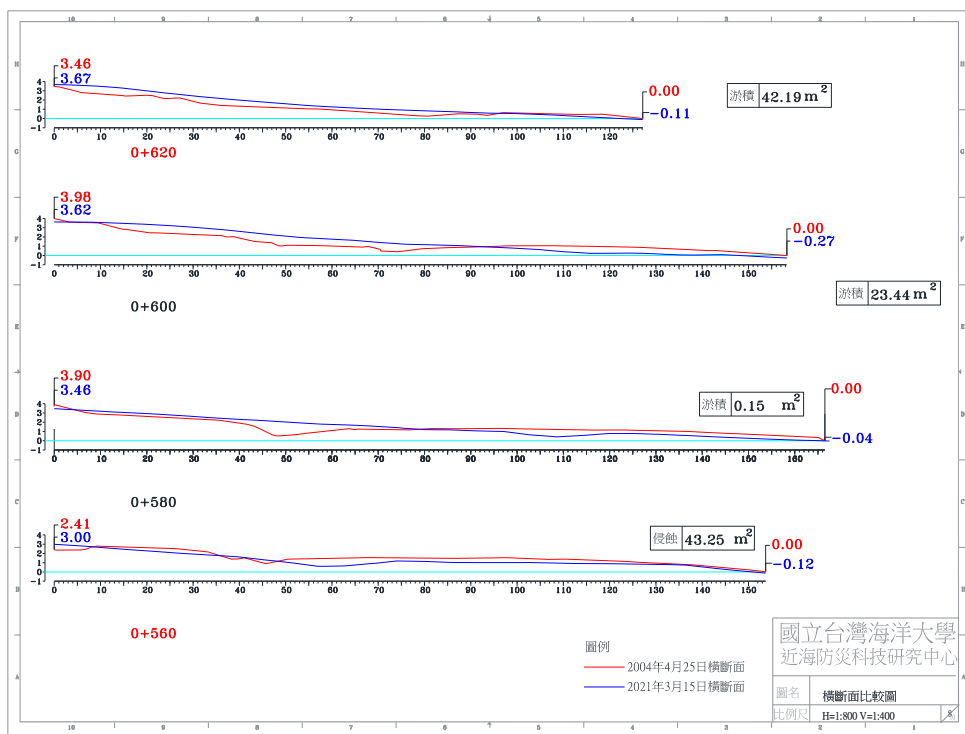
圖 4-4(c) 2021 年 3 月 15 日 A 監測區橫斷面比較圖
