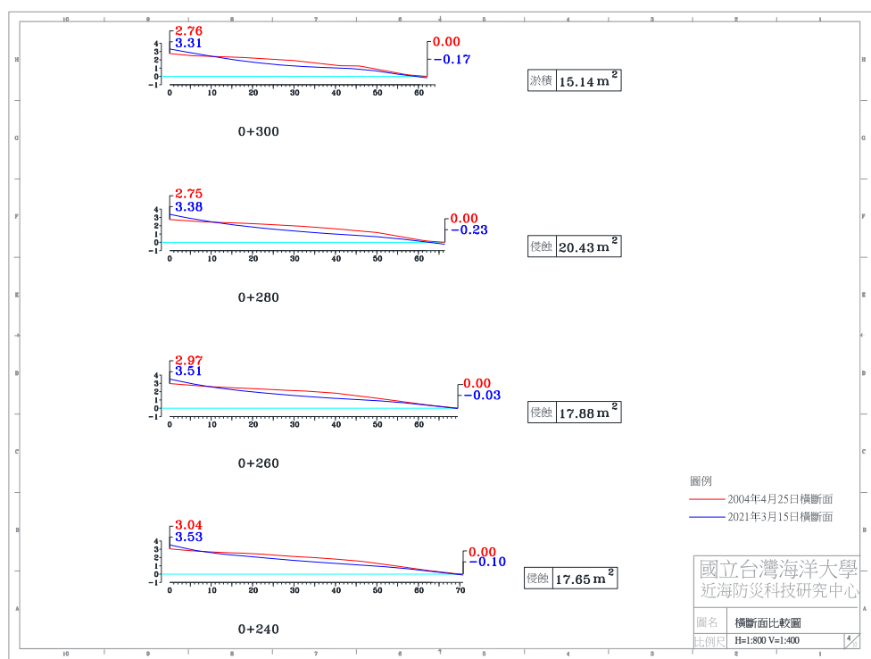
圖 4-4(g) 2021 年 3 月 15 日 A 監測區橫斷面比較圖
