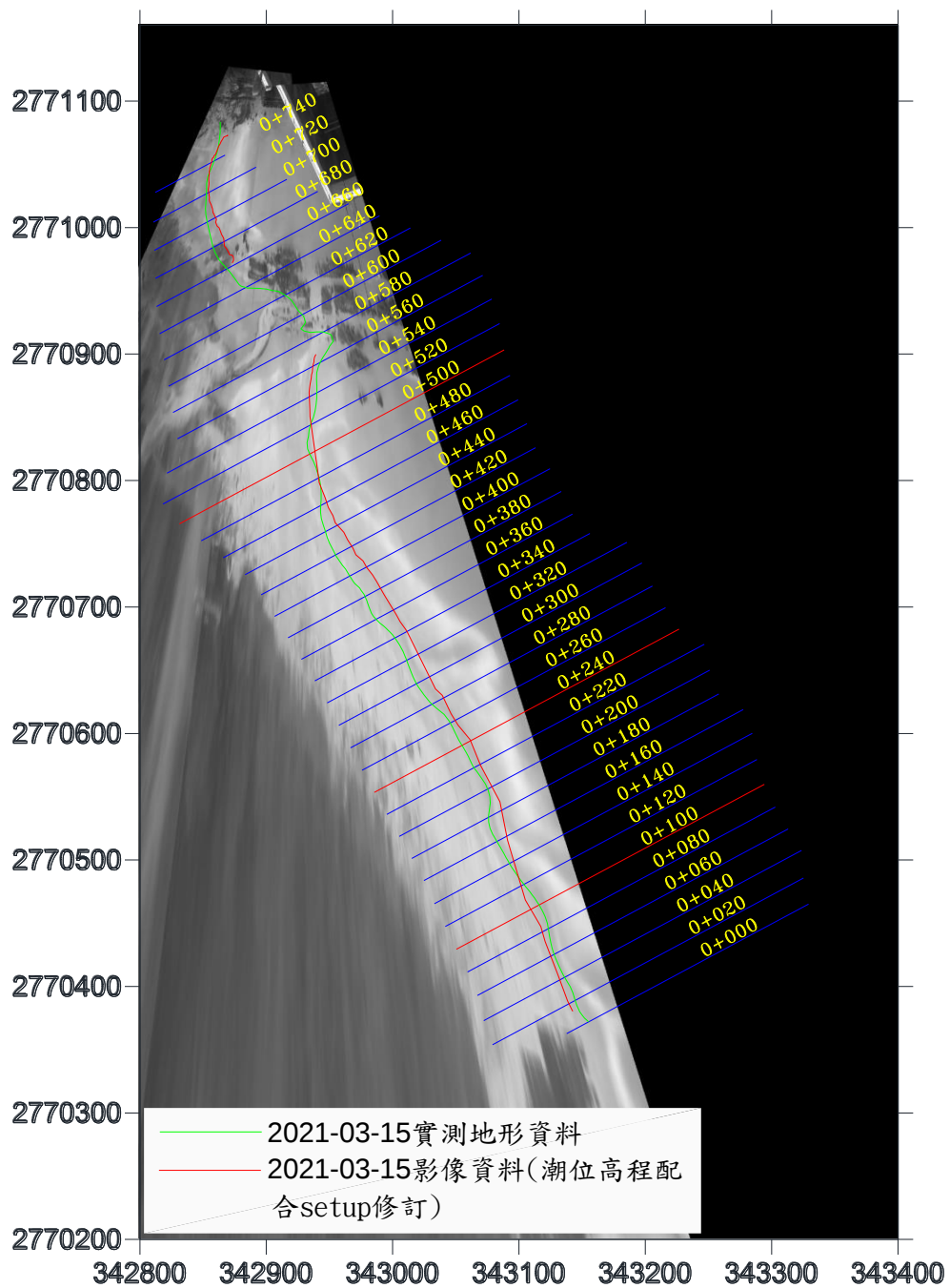
圖 3-22 水位線分析結果圖(2021/03/15)
