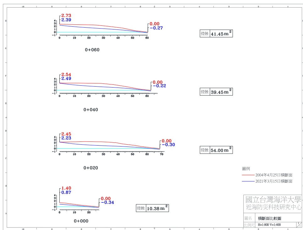
圖 4-4(j) 2021 年 3 月 15 日 A 監測區橫斷面比較圖
