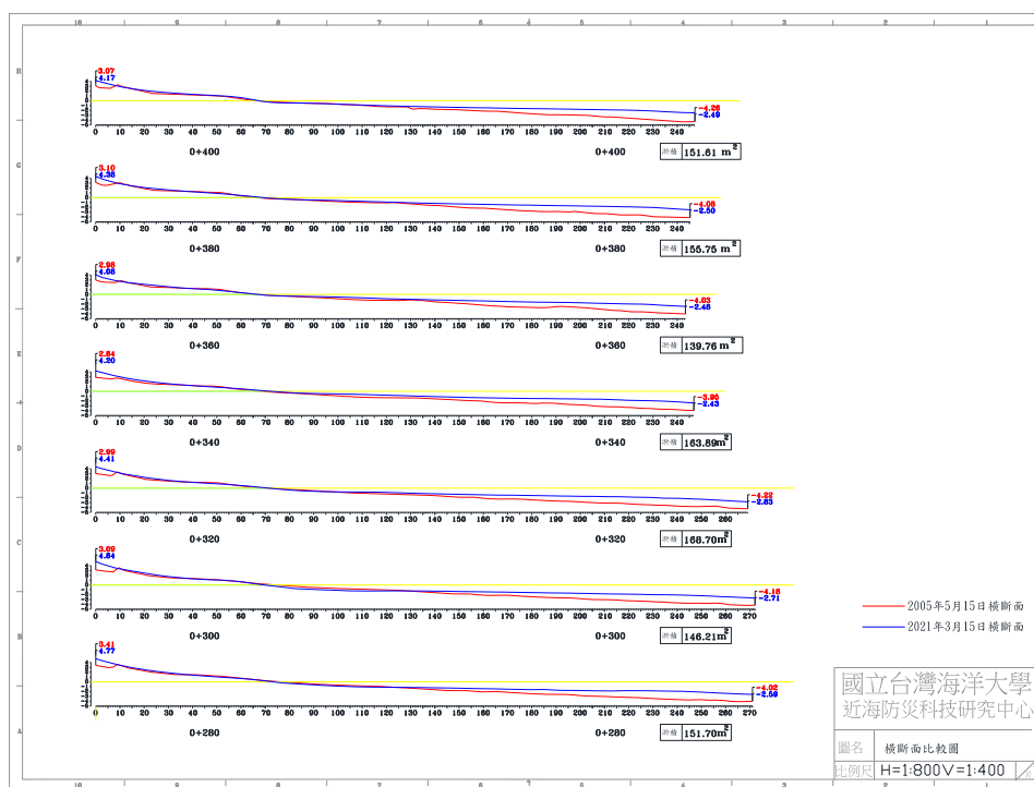
圖 4-5(d) 2021 年 3 月 15 日 B 監測區橫斷面比較圖
