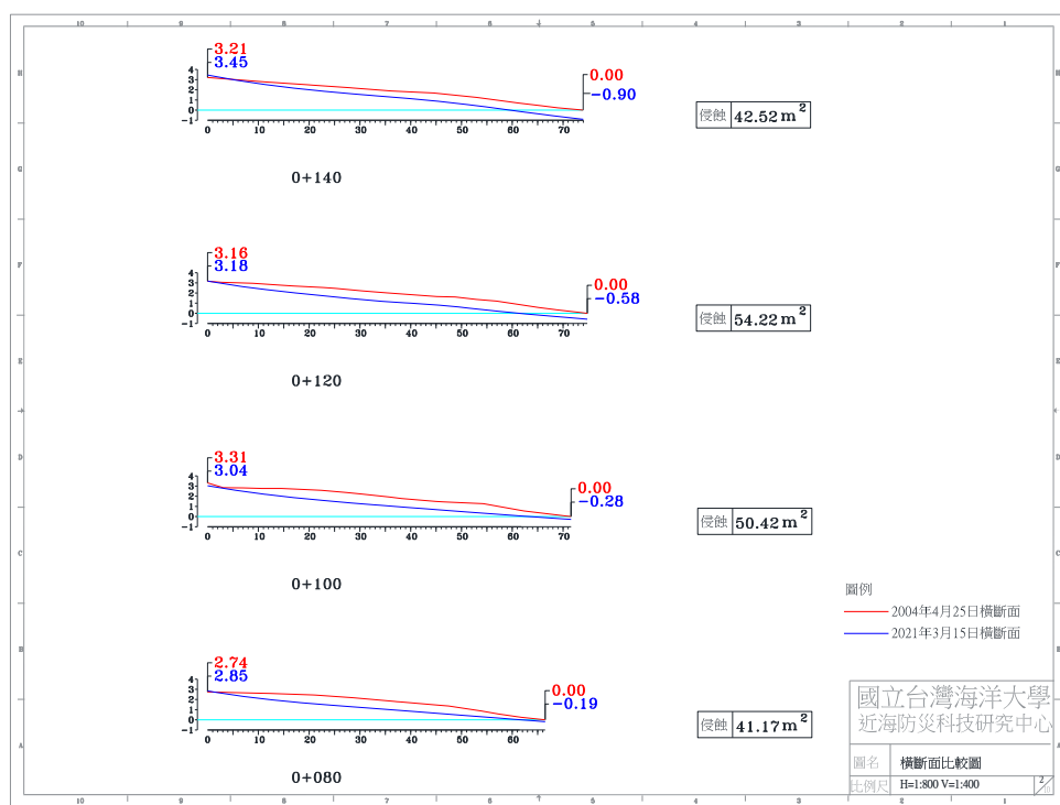
圖 4-4(i) 2021 年 3 月 15 日 A 監測區橫斷面比較圖
