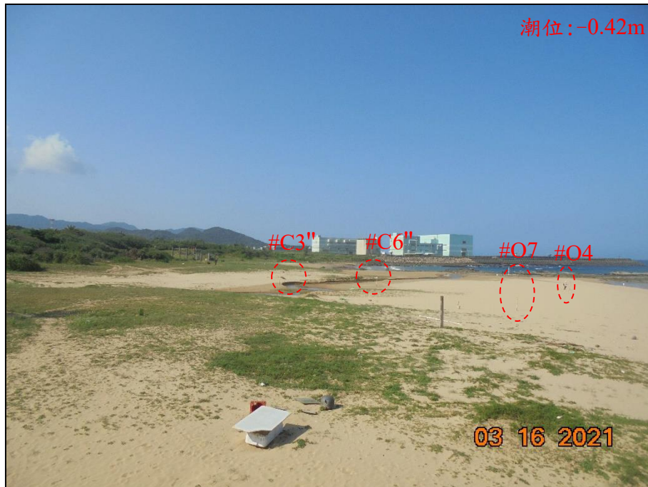
附圖 2-3 小舞台前輔助觀測樁位置圖(2021/03/16)
