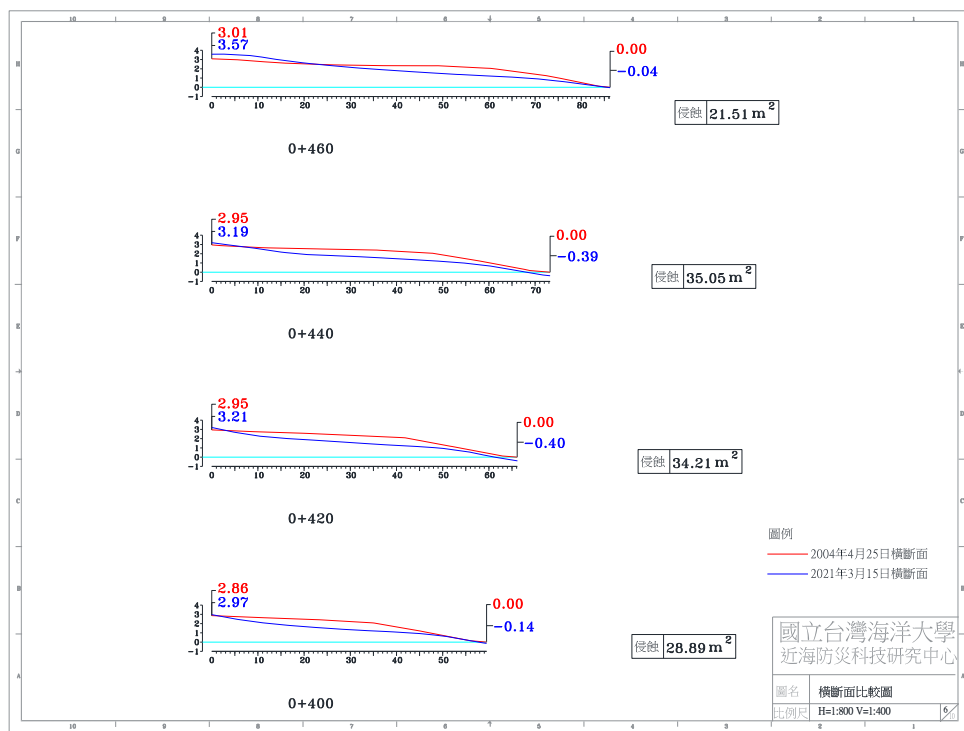
圖 4-4(e) 2021 年 3 月 15 日 A 監測區橫斷面比較圖
