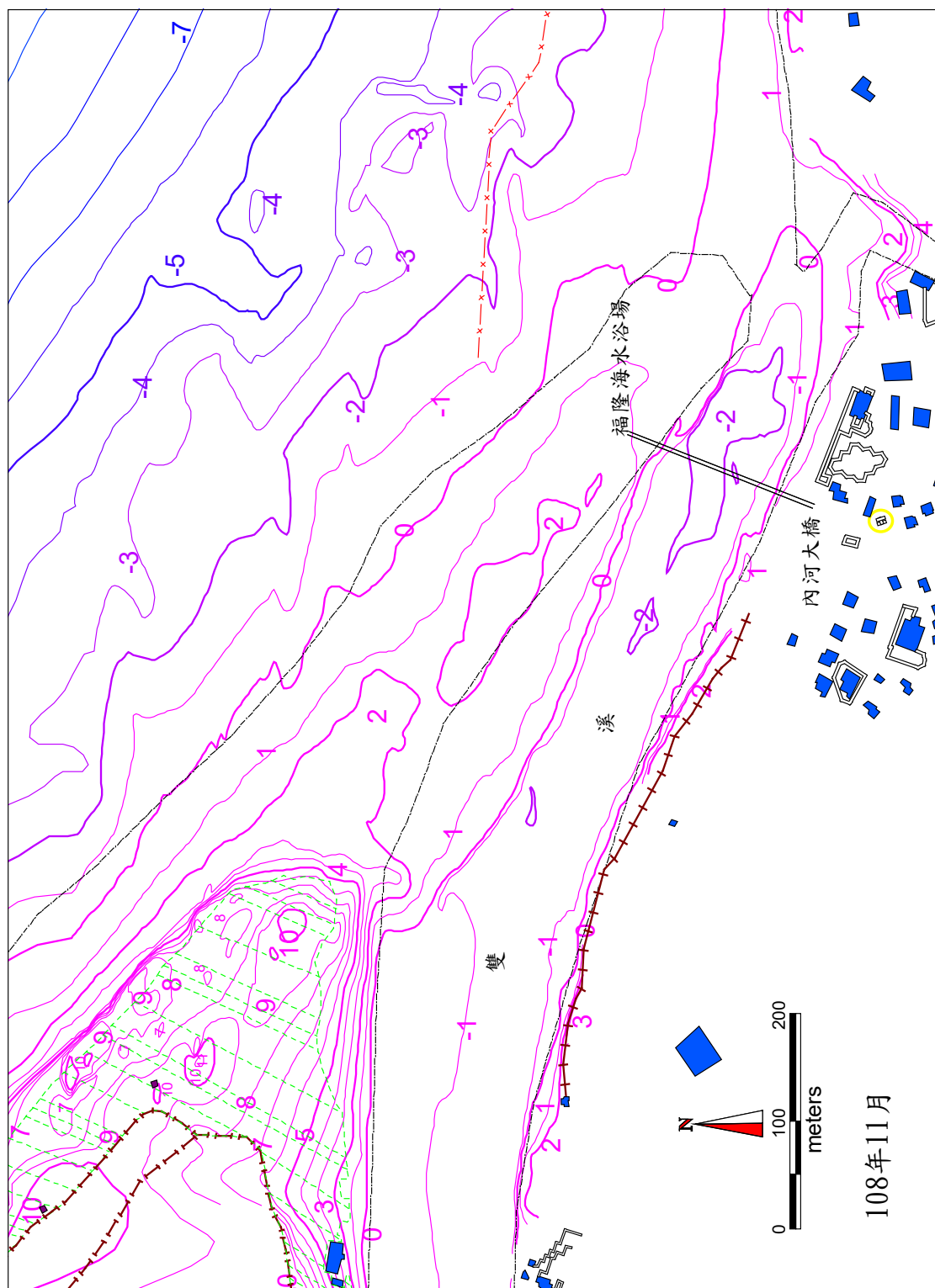
圖 2.5-4 核四封存期間福隆附近 108 年第 4 季海岸地形監測結果
