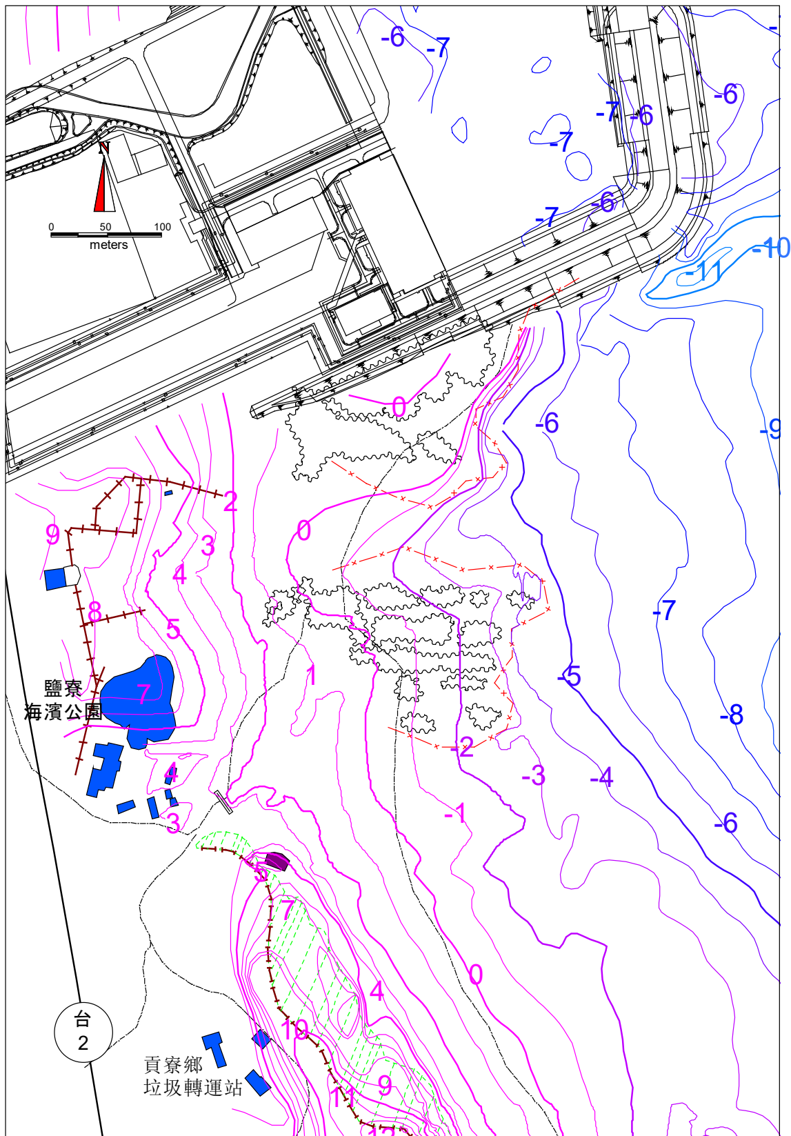
圖 2.5-3 核四封存期間鹽寮公園附近 108 年第 4 季 海岸地形監測結果
