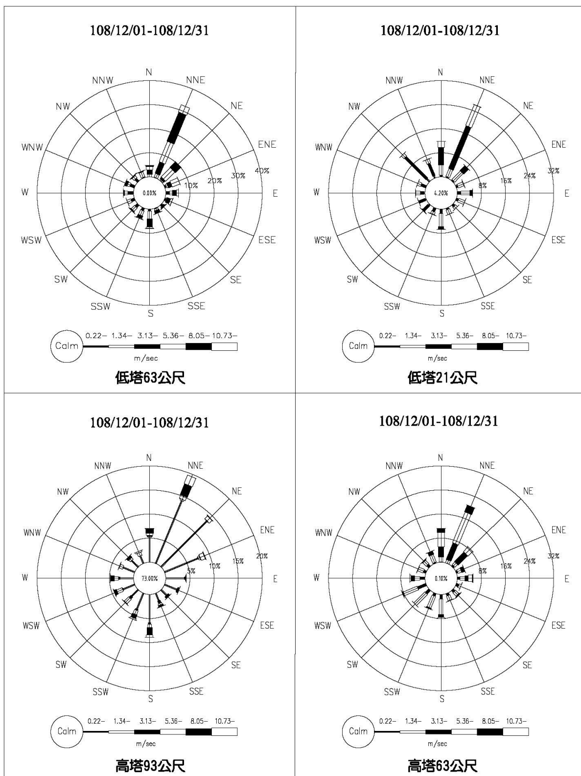
圖 2.1-2 核四封存期間環境監測氣象塔 108 年 12 月風花圖
