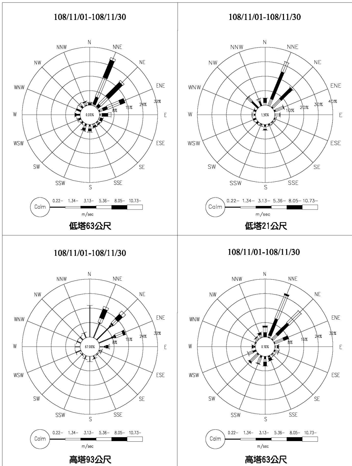
圖 2.1-2 核四封存期間環境監測氣象塔 108 年 11 月風花圖
