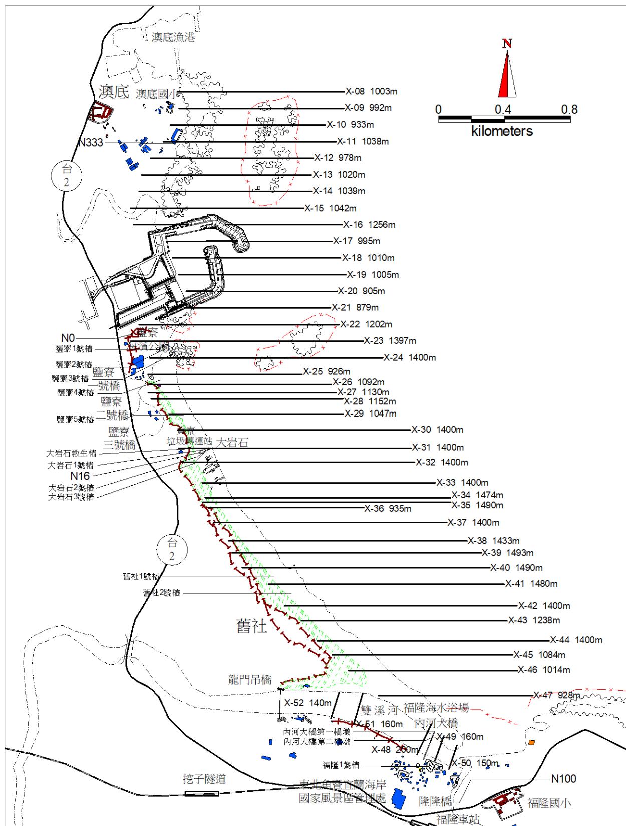
圖 2.5-1 核四封存期間附近海岸地形測量斷面位置圖
