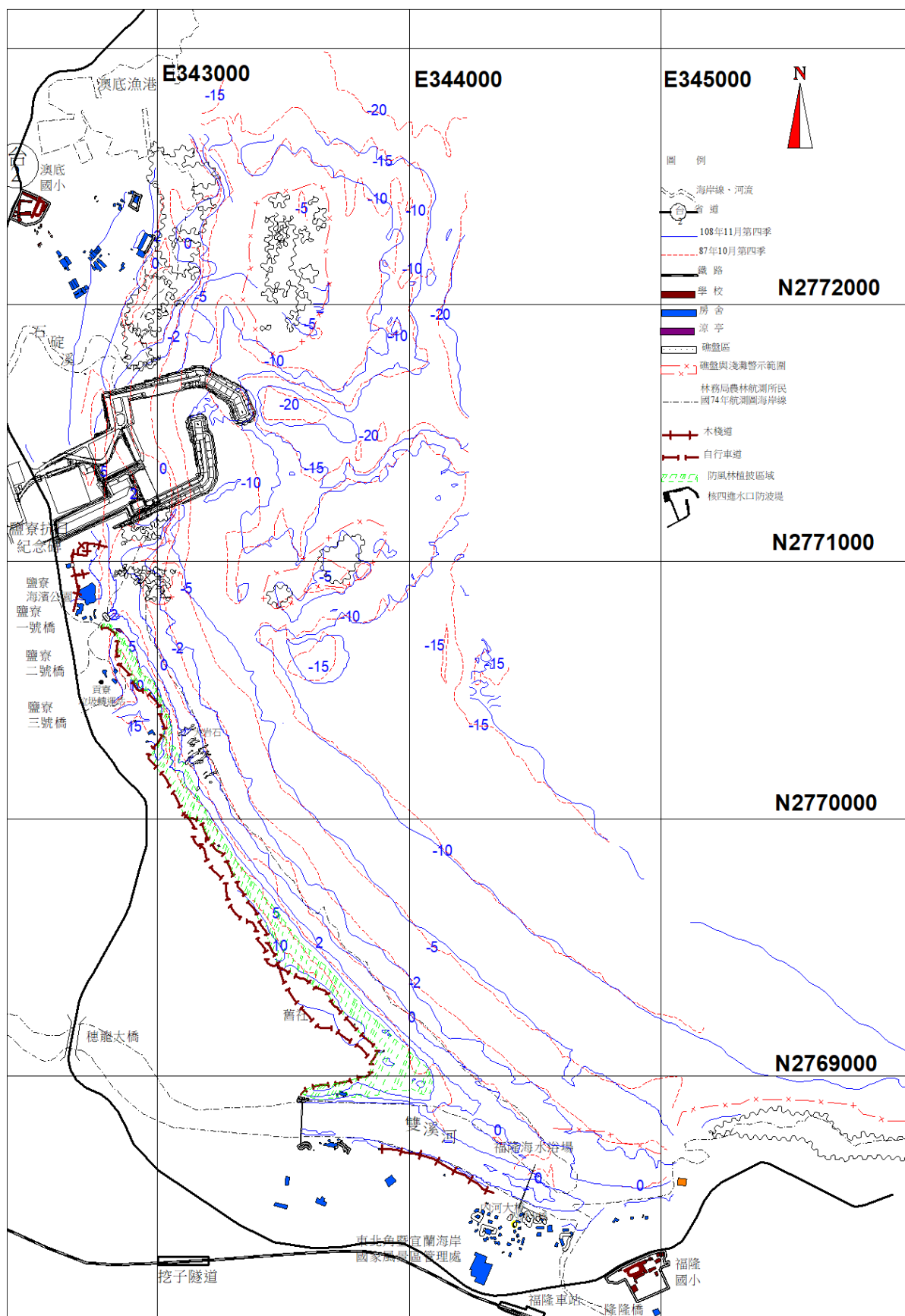
圖 3.1-13 核四環境監測海岸地形 108 年 10 月與 87 年 10 月（海事工程施工前）監測結果比較
