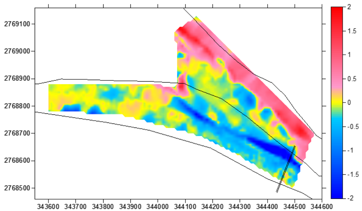
(B)108 年 11 月與 107 年 10 月福隆海水浴場侵淤比較圖
