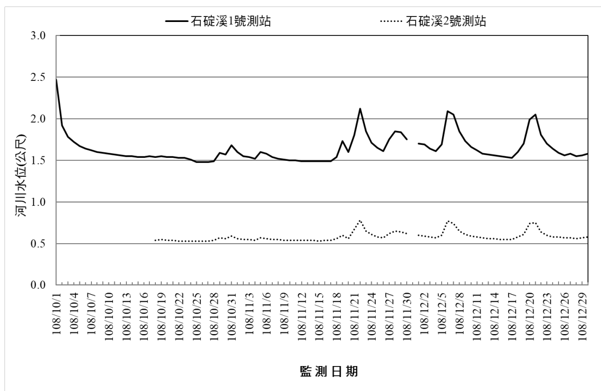
圖 2.2-1 核四封存期間河川水文 108 年 10~12 月水位變化圖
