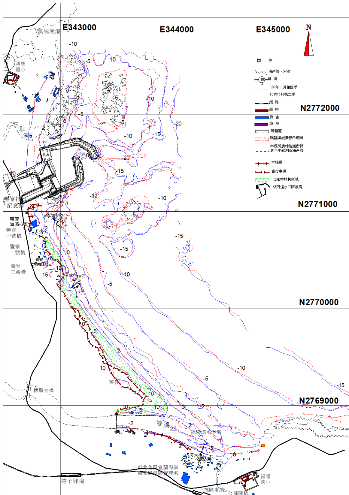
圖 2.5-5 核四封存期間海岸地形 108 年第 4 季與 108 年第 2 季監測結果比較
