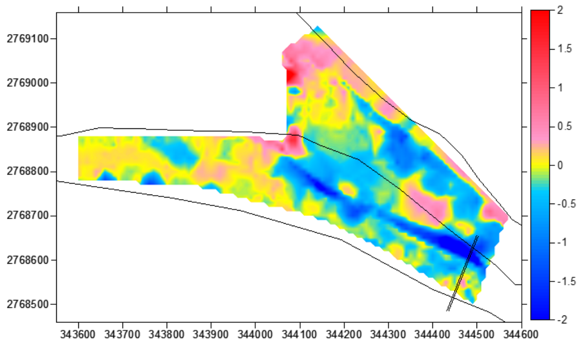
(A)108 年 11 月與 108 年 5 月福隆海水浴場侵淤比較圖
