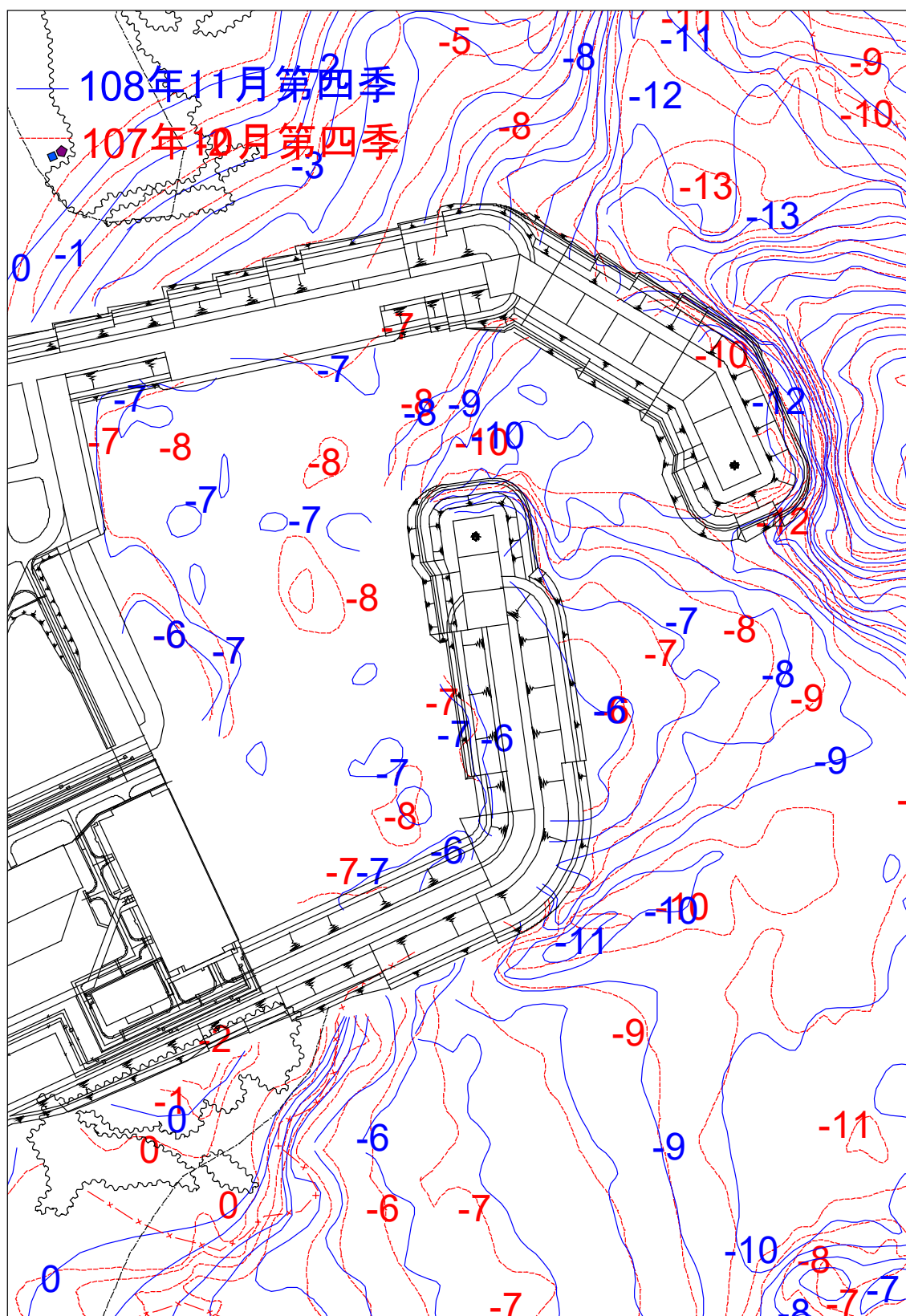
圖 3.1-11 核四環境監測海岸地形進水口防坡堤 108 年 11 月與 107 年 10 月監測結果比較
