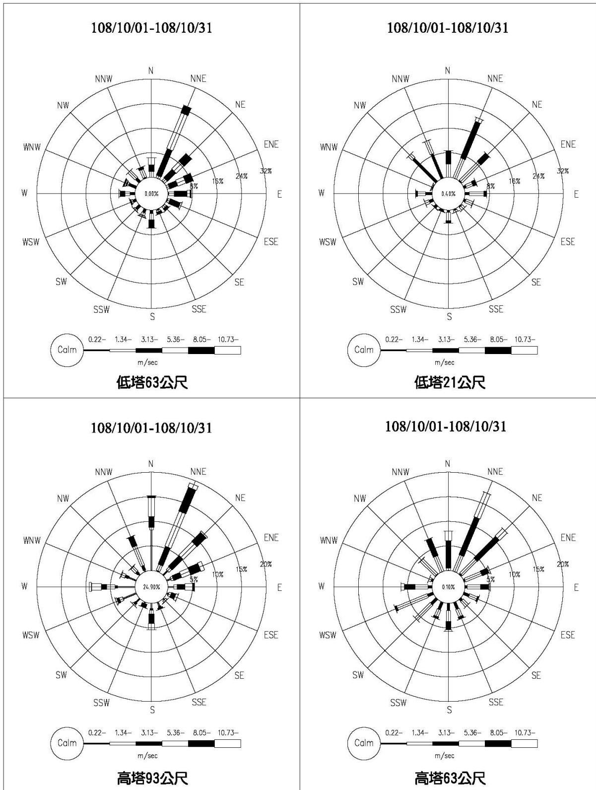
圖 2.1-1 核四封存期間環境監測氣象塔 108 年 10 月風花圖
