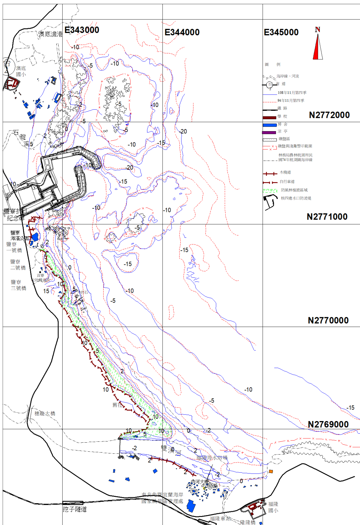
圖 3.1-14 核四施工環境監測海岸地形 108 年 11 月與 94 年 11 月監測結果比較
