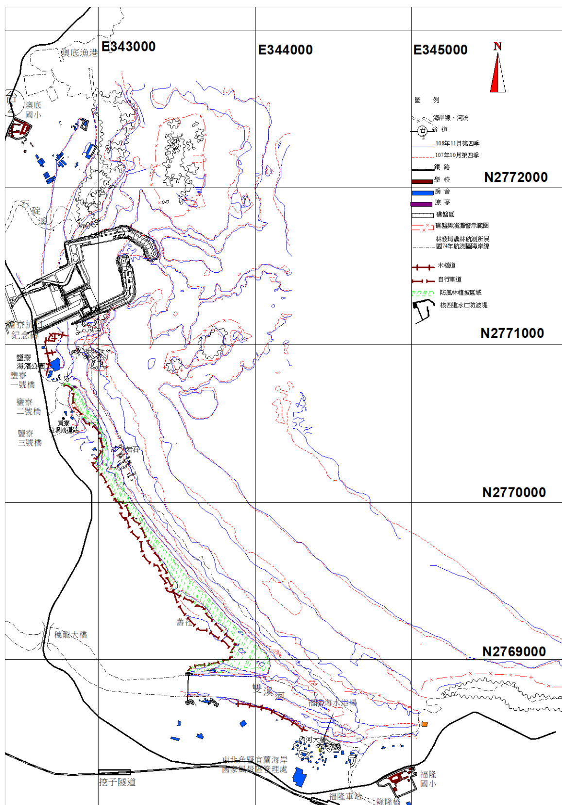
圖 3.1-10 核四環境監測海岸地形 108 年 11 月與 107 年 10 月 監測結果比較
