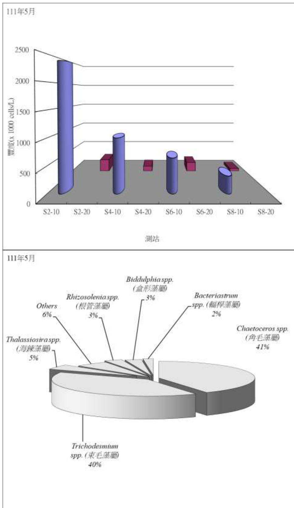
圖 2.10.1-1 民國 111 年 5 月於彰化濱海工業區附近海域各測站之浮游植物豐度分析圖
