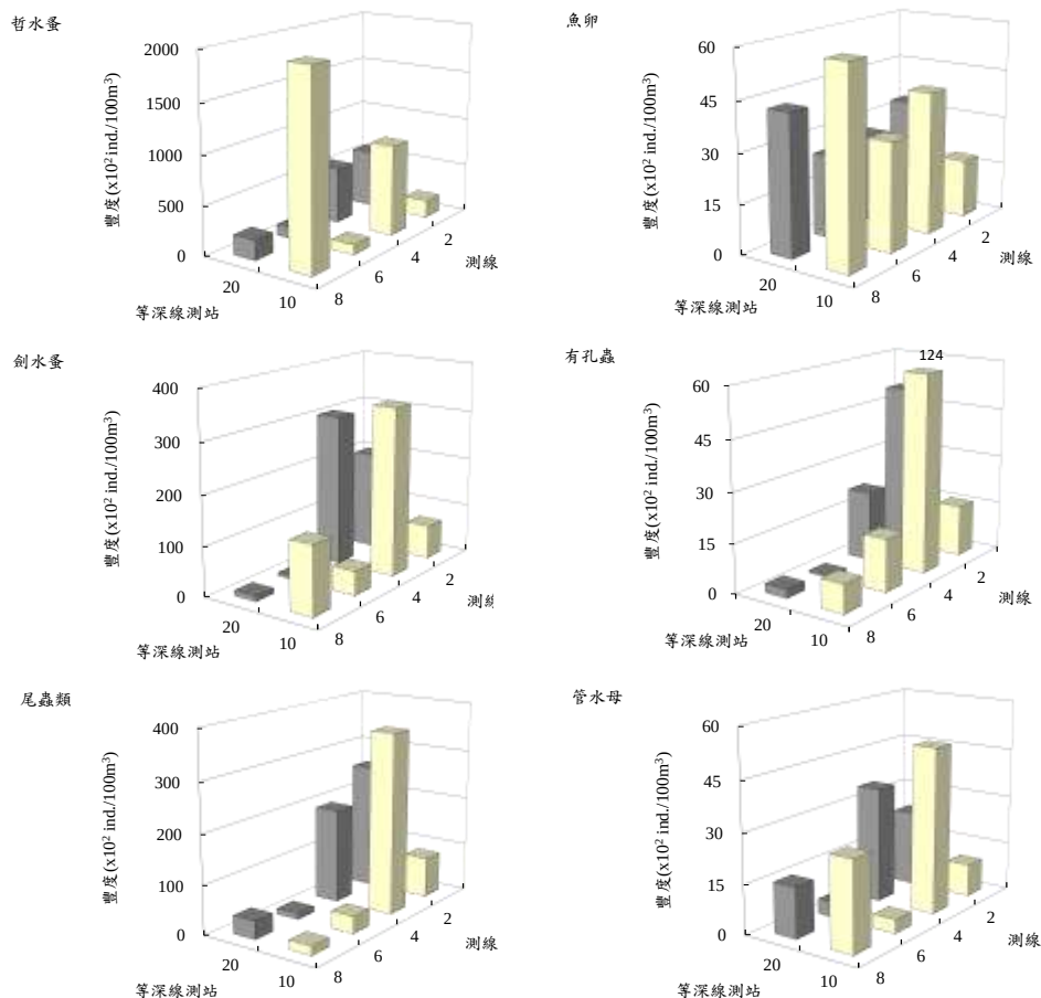
圖 2.10.2-2 民國 111 年 5 月彰化濱海工業區附近海域浮游動物主要優勢類群之豐度分布圖
