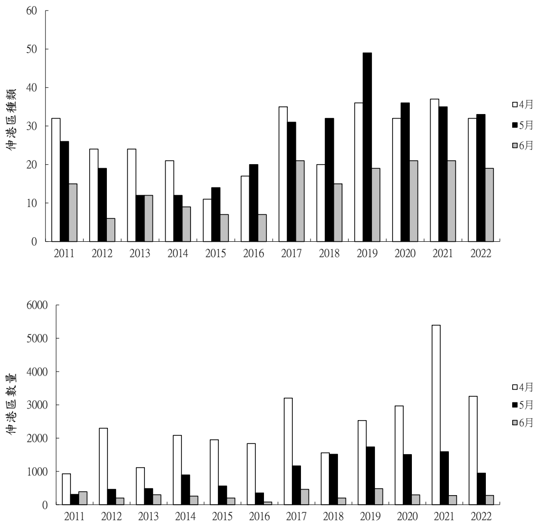
圖 3.1.5-1 仲港區歷年同期鳥類調查結果比較
