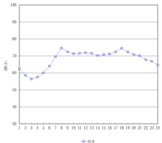
圖 2.2-6 海埔國小本季噪音測值逐時變 化圖
