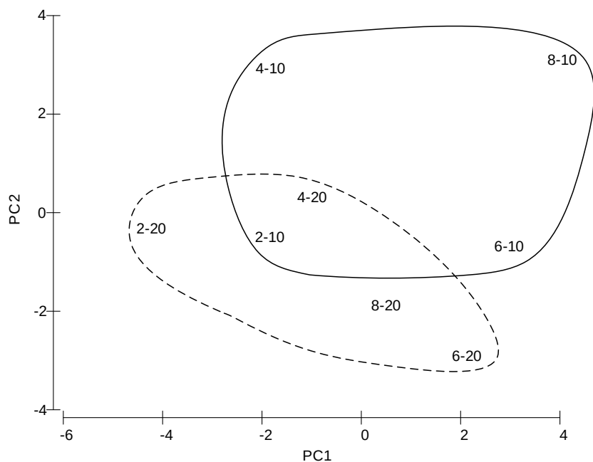
圖 2.10.2-3 民國 111 年 5 月彰濱工業區附近海域各測站浮游動物群聚分析圖(圖中第一個數字代表測站，第二個數字代表深度)
