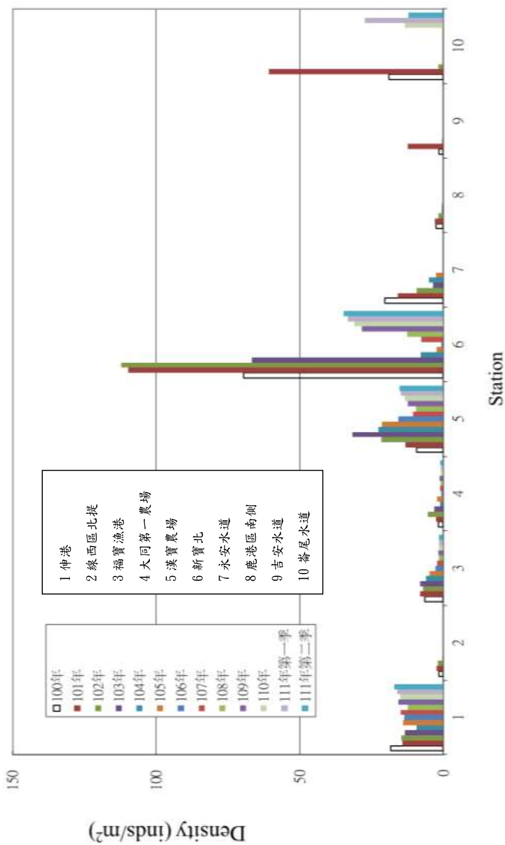
圖 3.1.6-1 各測站螞蛄蝦平均密度(個體數/m 2 )分布圖
