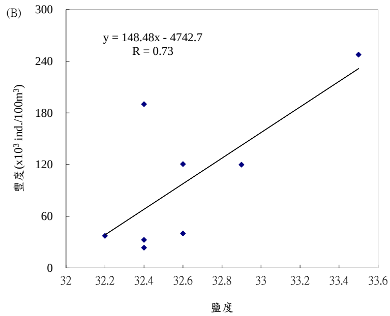
圖 2.10.2-4 民國 111 年 5 月彰濱工業區之浮游動物豐度與(A)溫度 (B)鹽度之相關係數圖
