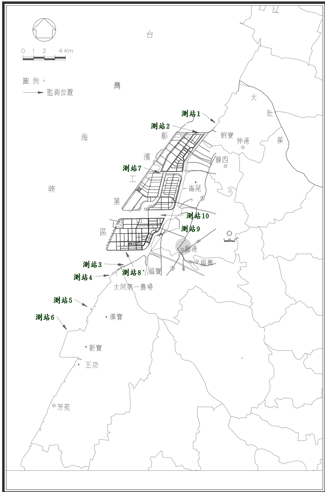
圖 1.4-10 施工及營運期間螞蟧蝦監測站位置
