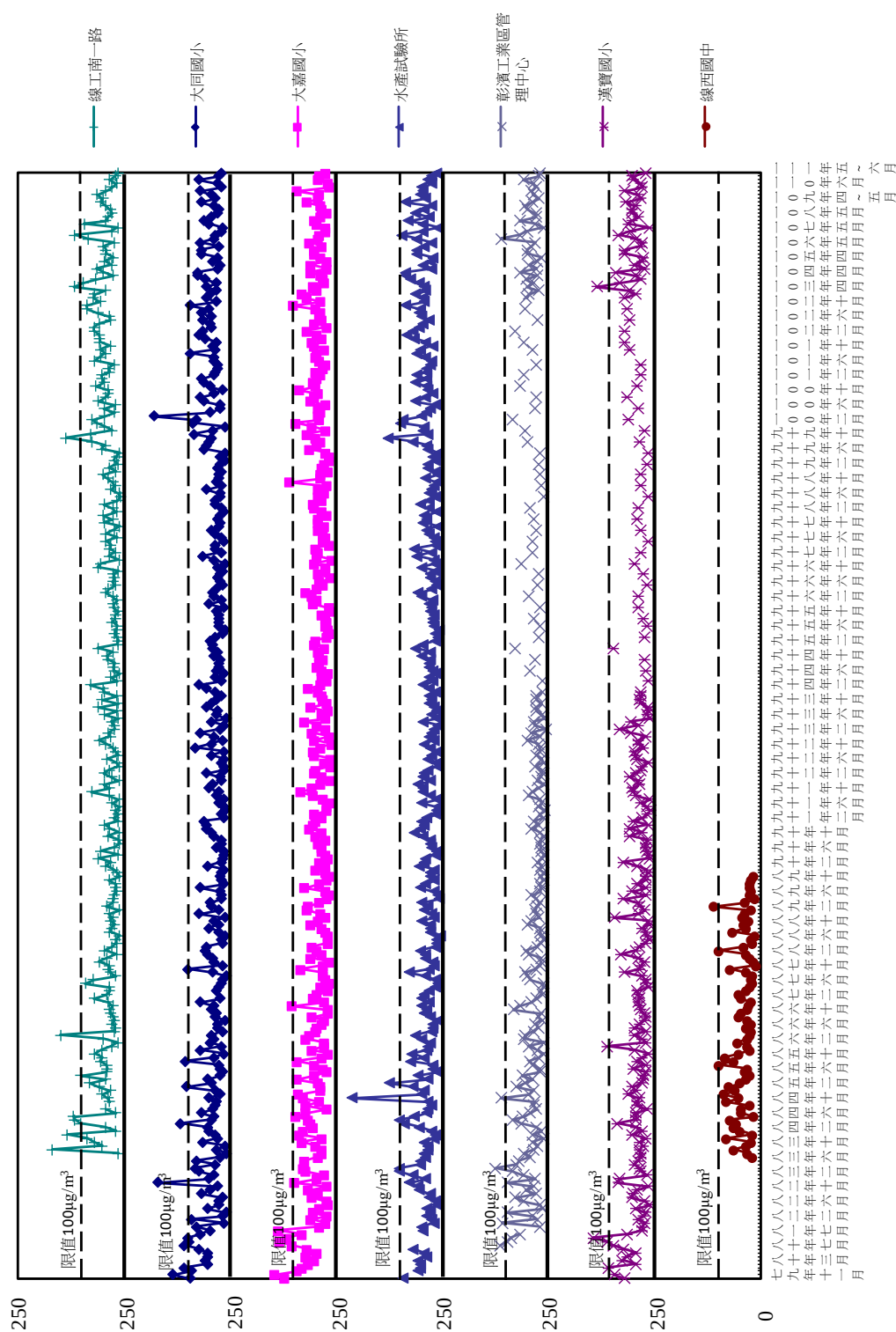
圖 3.1.1-7 彰濱地區歷年粒徑小於 10\mu\text{m} 之懸浮微粒( \text{PM}_{10} )日平均值監測結果分析圖
