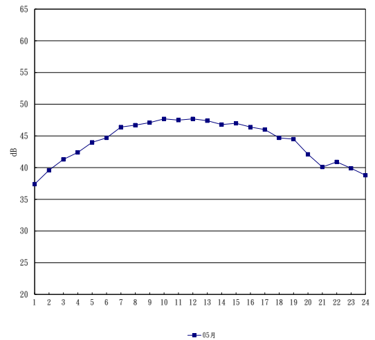
圖 2.3-2 西濱快與 2 號連絡道交叉日本季振動測值逐時變化圖
