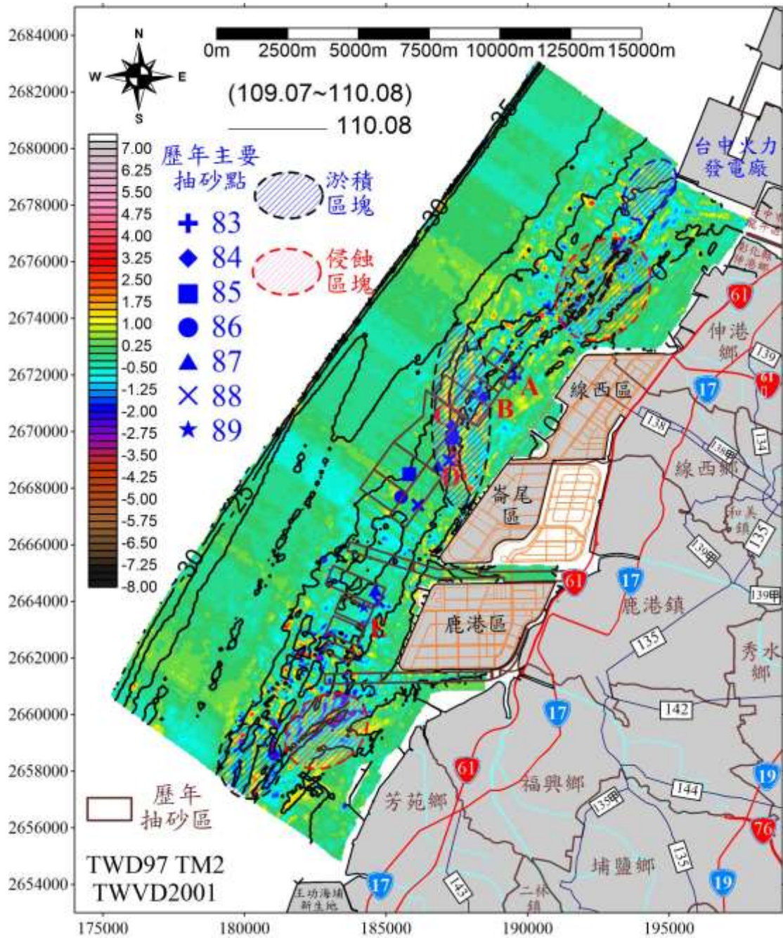
圖 2.11-4 109 年 7 月與 110 年 8 月海底地形侵淤圖
