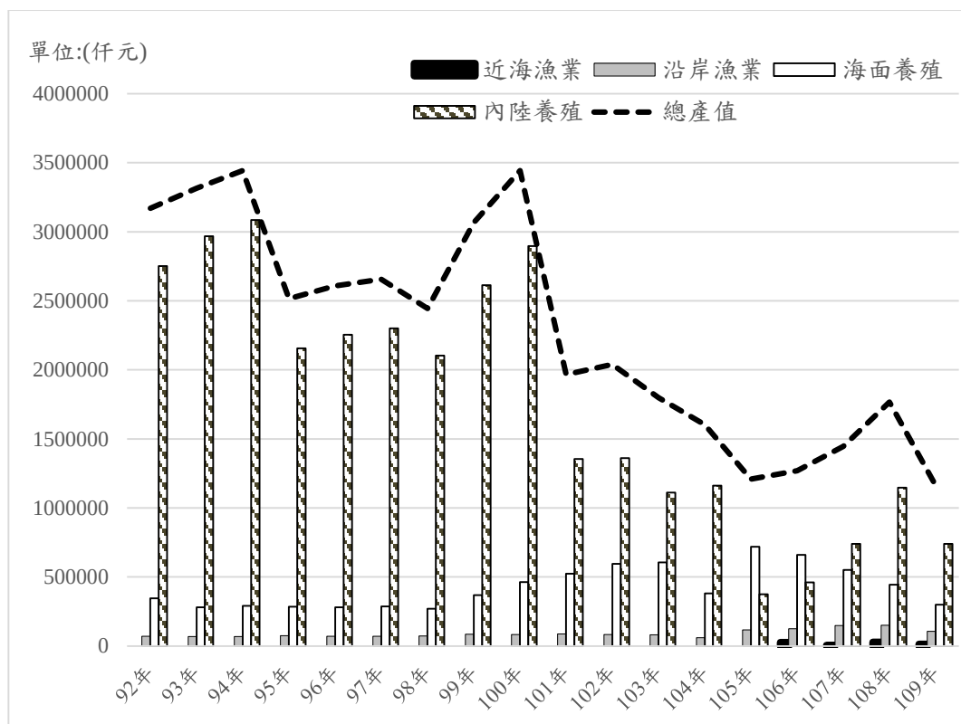
圖 2.13-2 各項漁業類別產值年間變化圖
