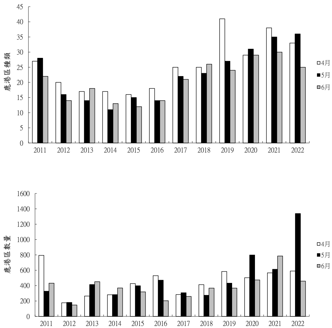
圖 3.1.5-5 鹿港區北測海堤歷年同期鳥類調查結果比較
