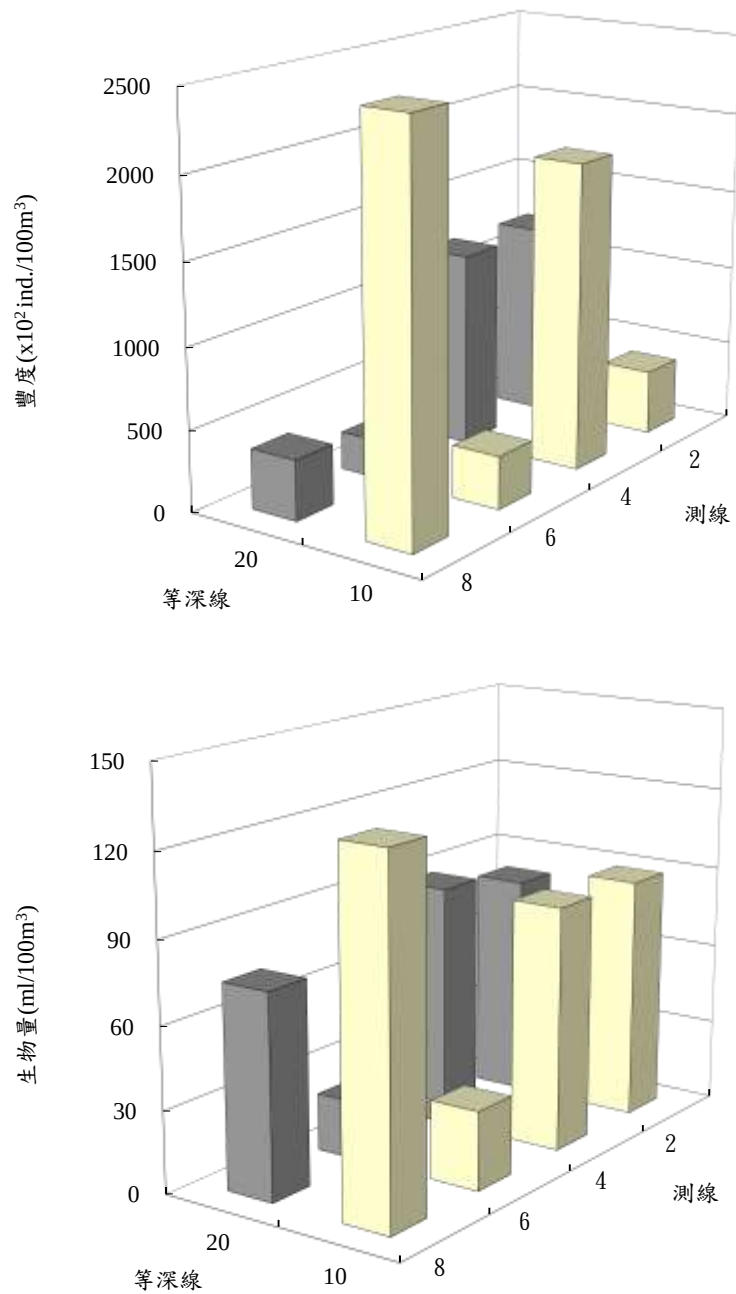
圖 2.10.2-1 民國 111 年 5 月彰化濱海工業區附近海域浮游動物之豐度及生物量分布圖
