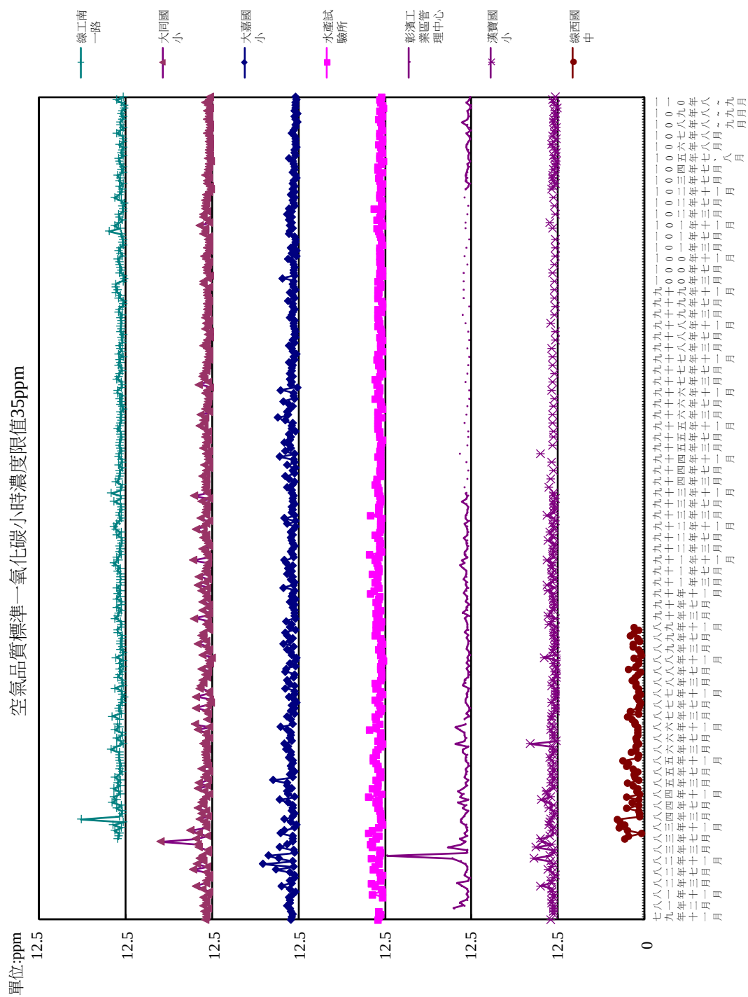
圖 3.1.1-1 彰濱地區歷年一氧化碳(CO)最高小時值監測結果分析圖
