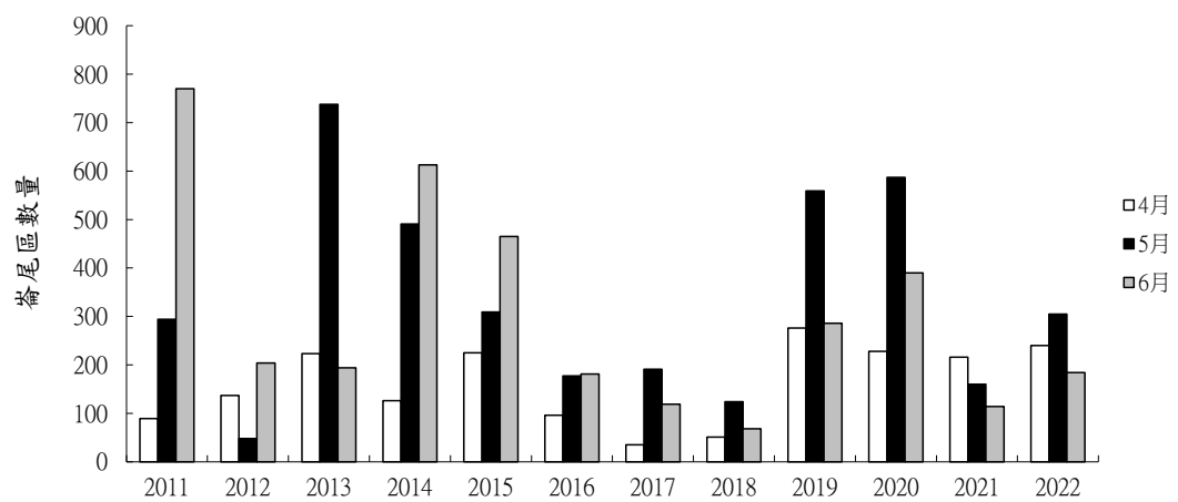
圖 3.1.5-4 嵛尾西側海堤歷年同期鳥類調查結果比較
