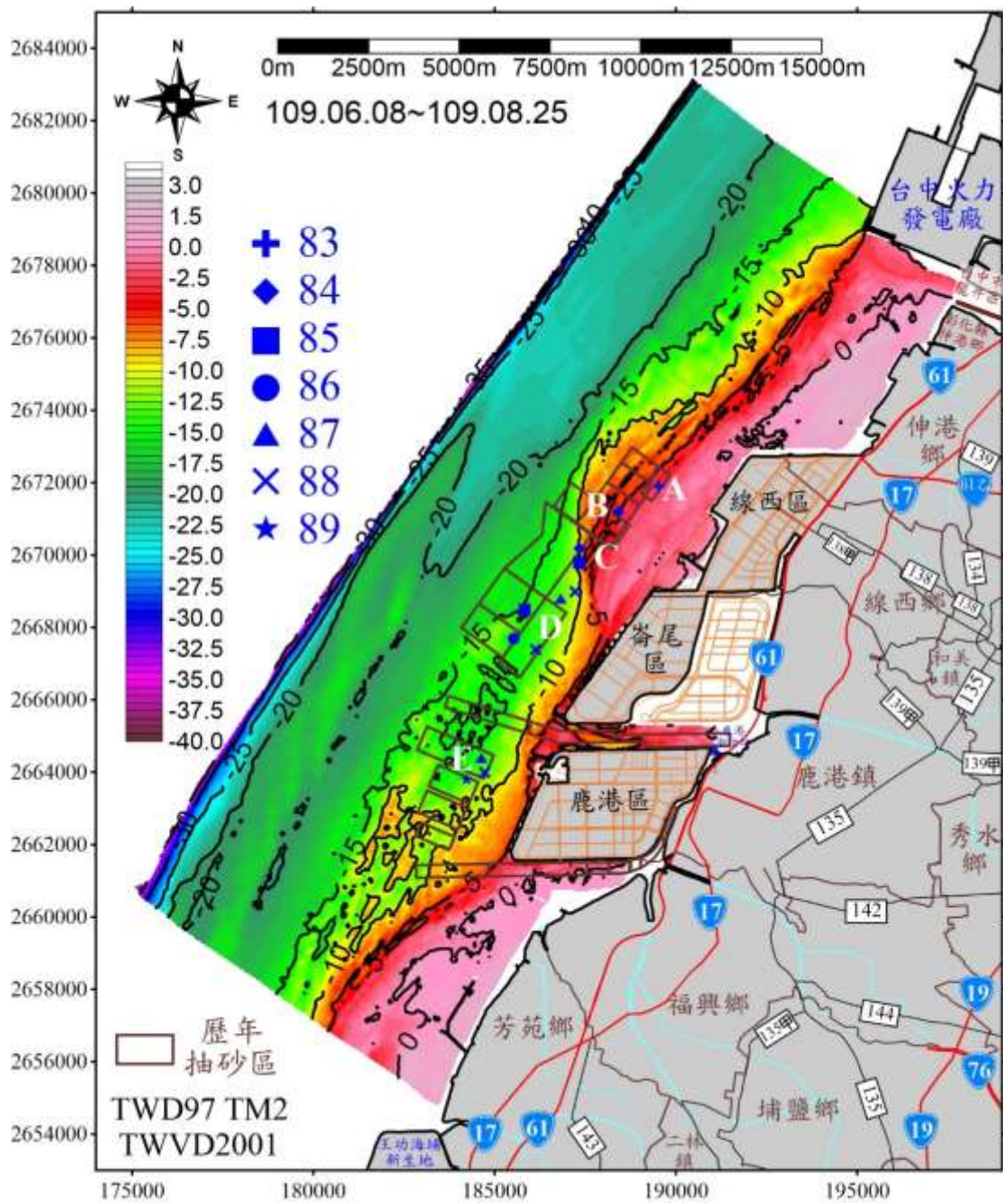
圖 2.11-1 109 年 6 月~8 月海底地形影像圖
