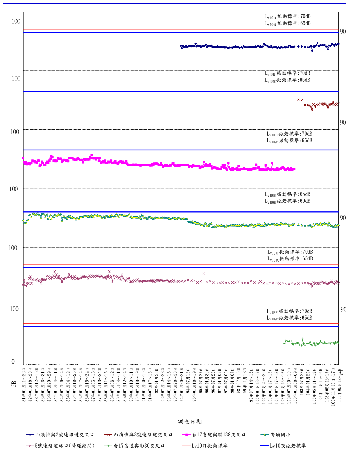
圖 3.1.3-1 彰濱地區歷次振動 L_{v10}(24\text{ 小時}) 監測結果
