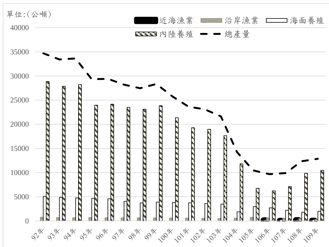
圖 2.13-1 各項漁業類別產量年間變化圖
