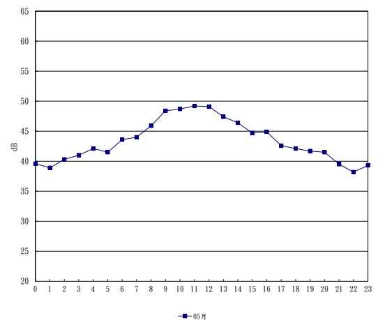
圖 2.3-4 西濱快與 3 號連絡道交叉日本季振動測值逐時變化圖
