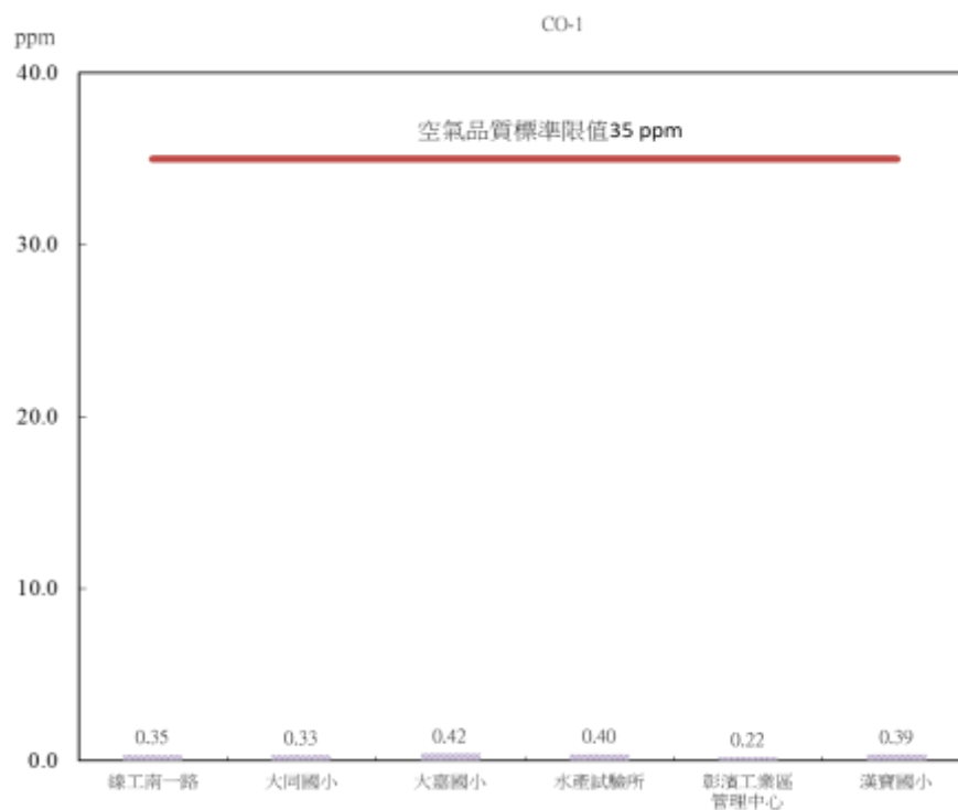
圖 2.1-2 本季各測站 CO 最高小時值監測結果比較分析圖
