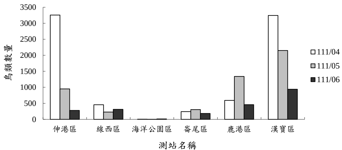
圖 2.5-2 本季各測站鳥類數量分布圖
