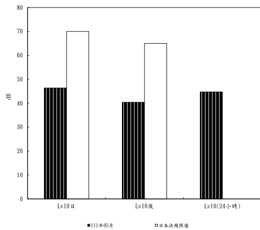
圖 2.3-3 西濱快與 3 號連絡道交叉日本季振動調查結果分析圖
