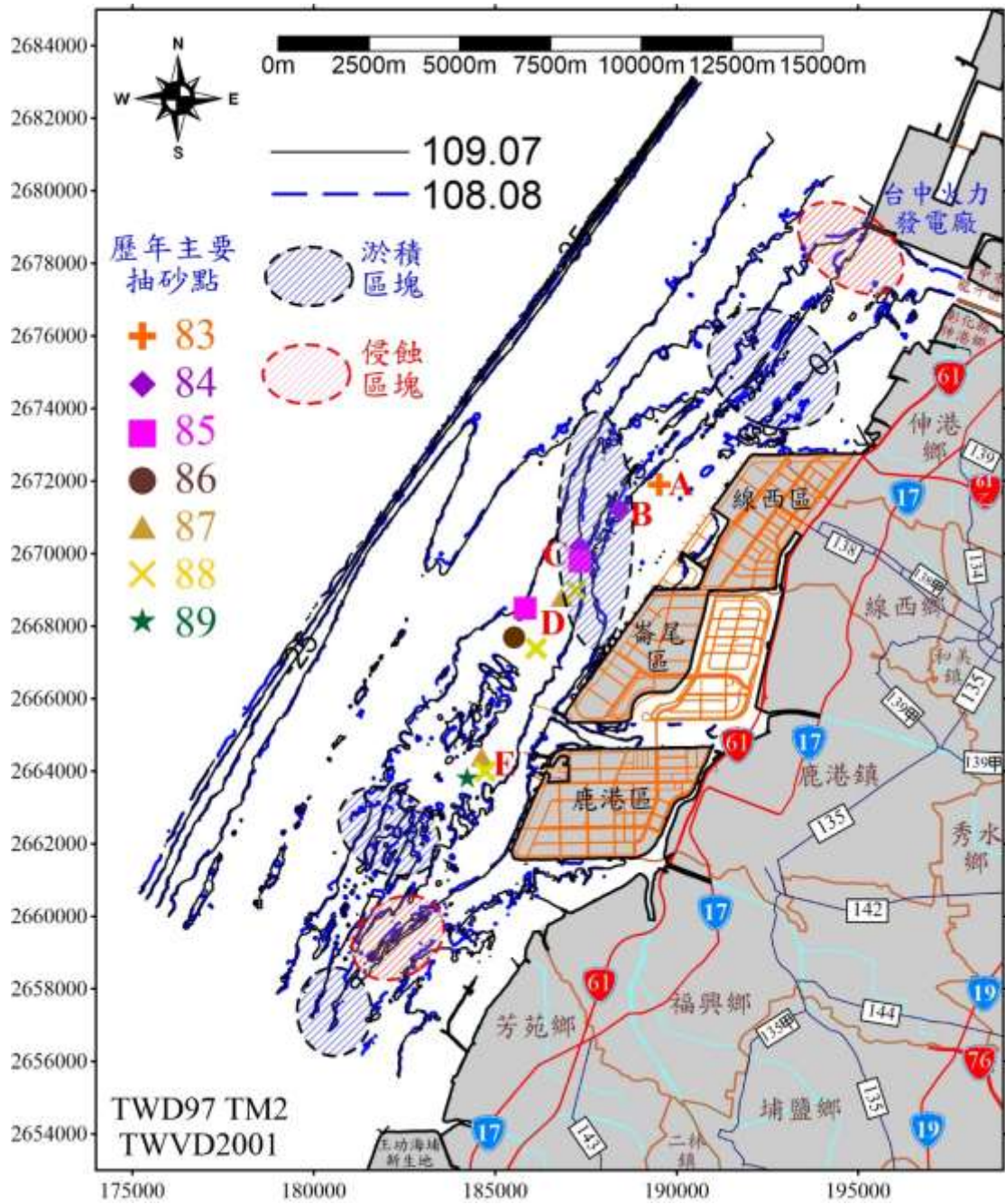
圖 2.11-3 108 年 8 月與 109 年 7 月兩次施測地形等深線比較圖
