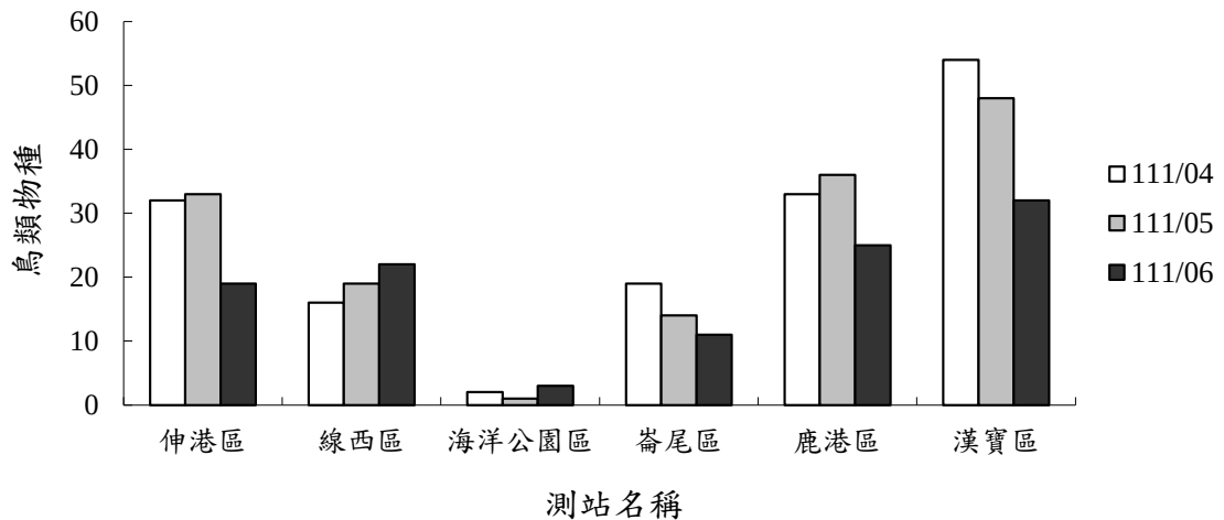
圖 2.5-1 本季各測站鳥類種數分布圖
