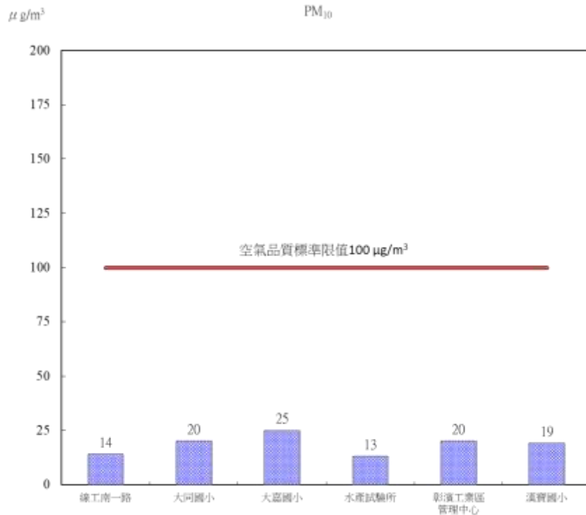
圖 2.1-9 本季各測站 PM 10 日平均值監測結果比較分析圖
