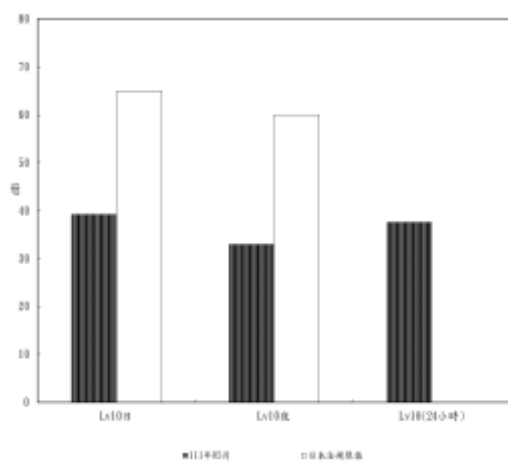
圖 2.3-5 海埔國小本季振動調查結果分析圖
