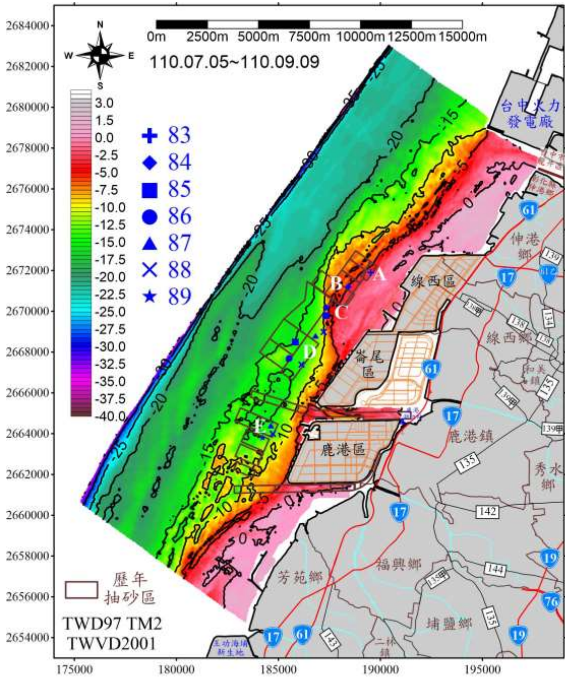
圖 2.11-2 110 年 7 月~9 月海底地形影像圖
