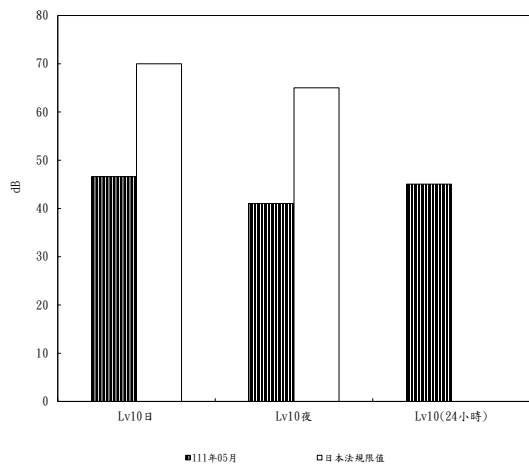
圖 2.3-1 西濱快與 2 號連絡道交叉日本季振動調查結果分析圖
