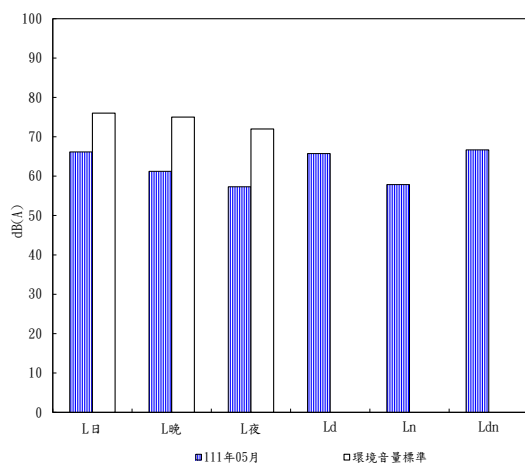
圖 2.2-9 台 17 省道與彰 30 交叉口本季噪音調查結果分析圖
