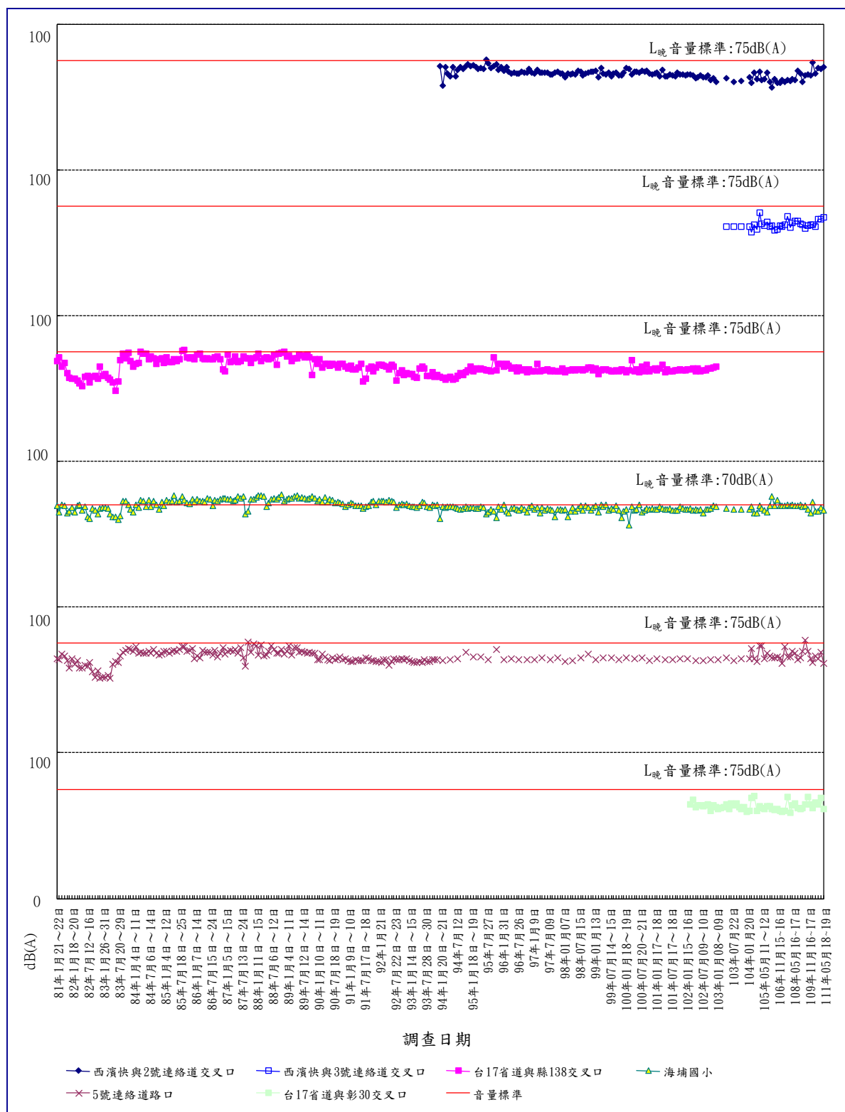
圖 3.1.2-2 彰濱地區歷次噪音 L_{\text{晚}} 監測結果
