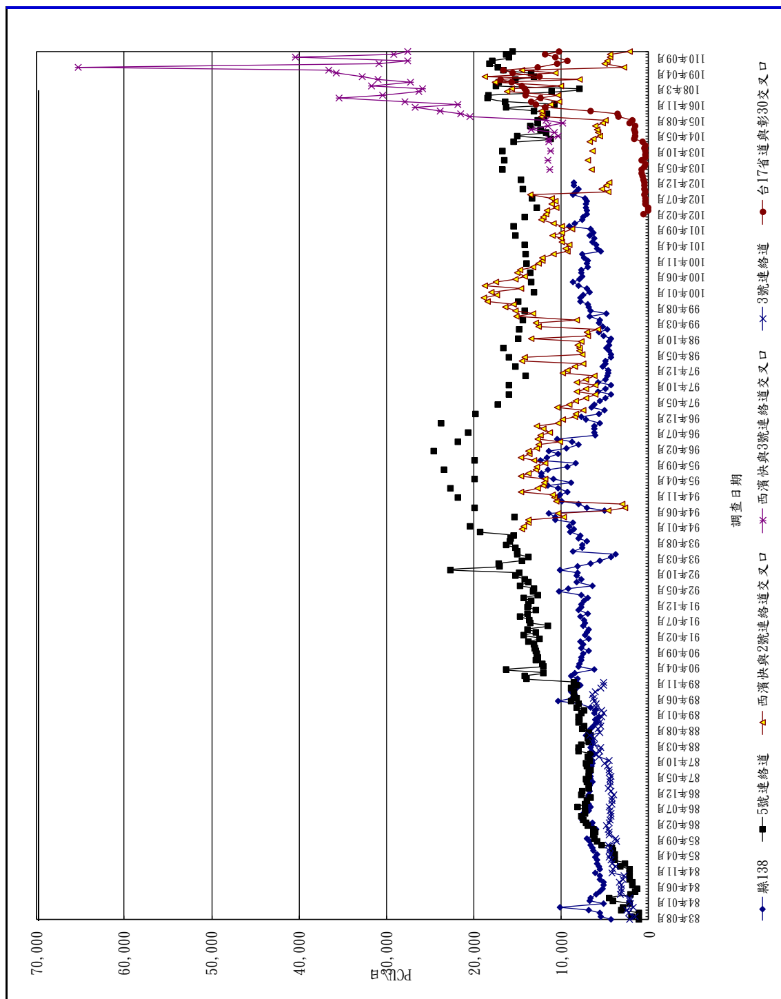
圖 3.1.4-1 彰濱地區歷次交通流量監測結果(2/2)
