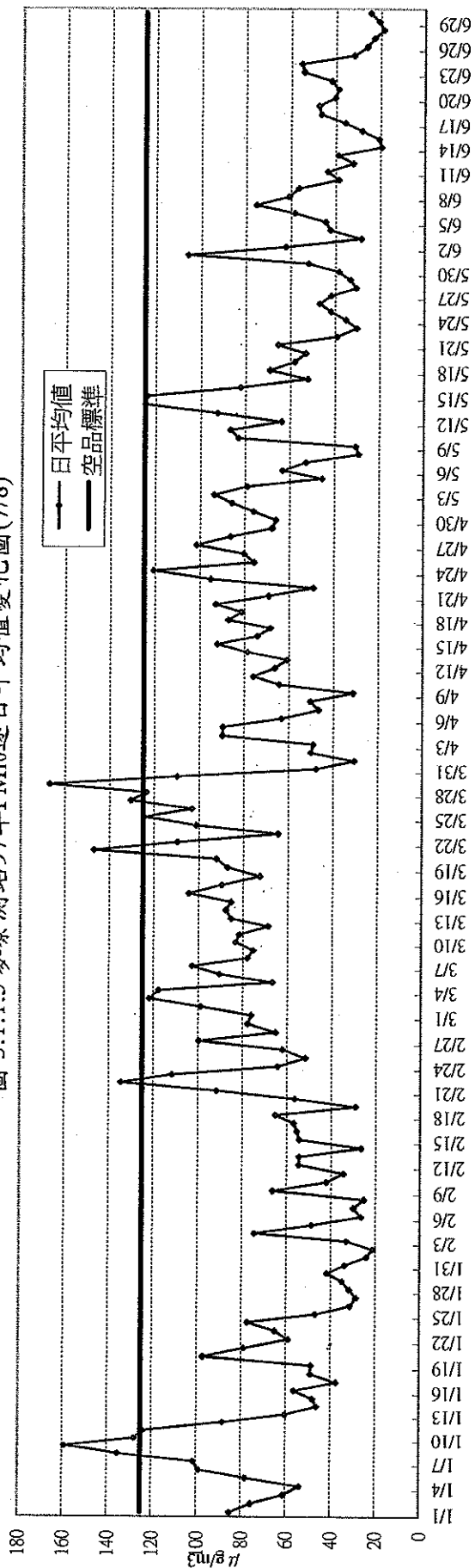
圖 3.1.1.3 麥寮測站97年TSP逐日平均值變化圖(8/8)
