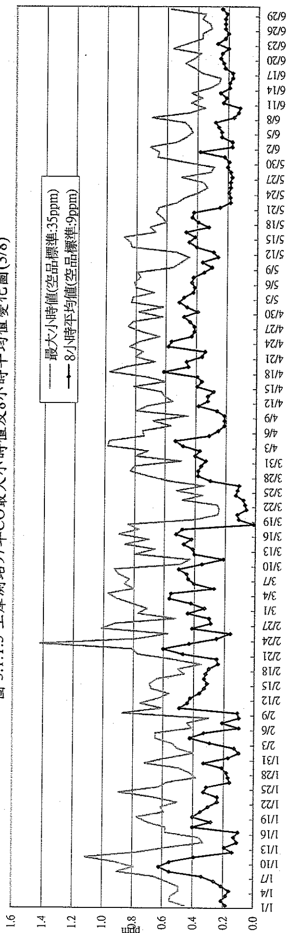
圖 3.1.1.5 參寮測站97年O3最大小時值及8小時平均值變化圖(4/8)
