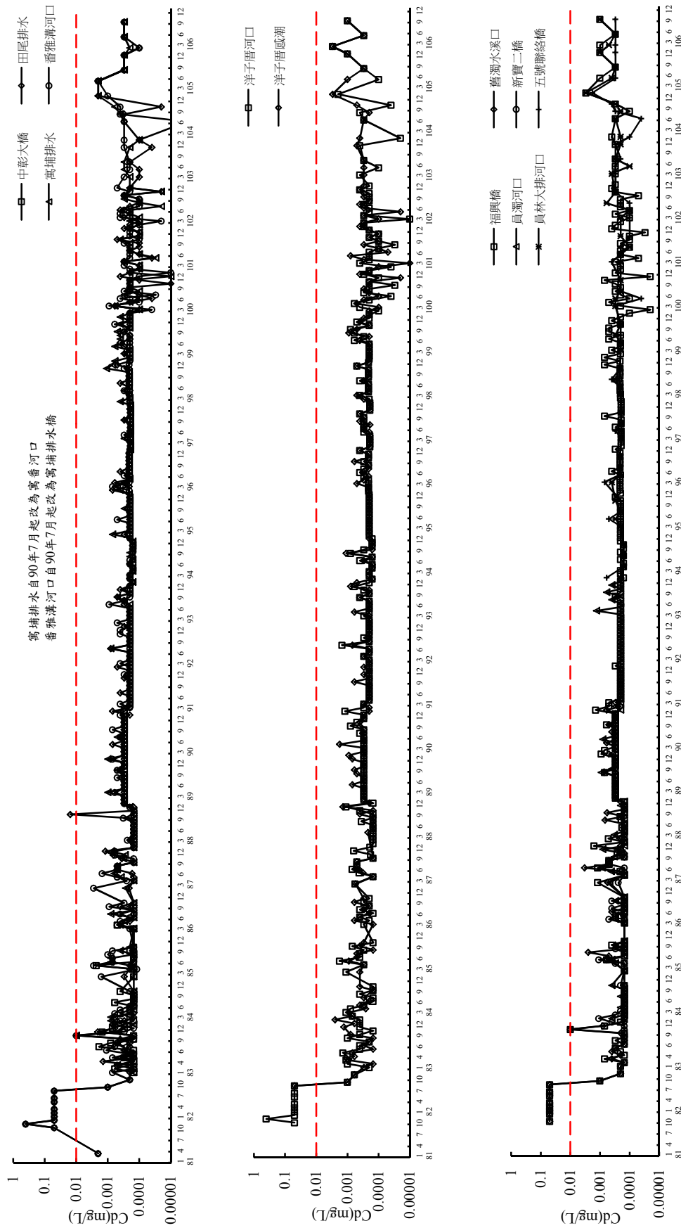
時間(民國年), 對數圖 附圖III.7-26(b) 歷次彰濱河口退潮鎘調查結果
