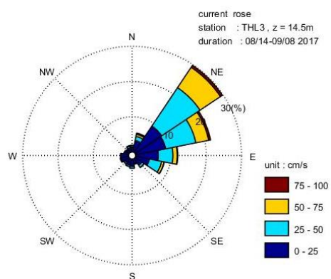
附錄III.11圖-6 THL3流速流向玫瑰圖
