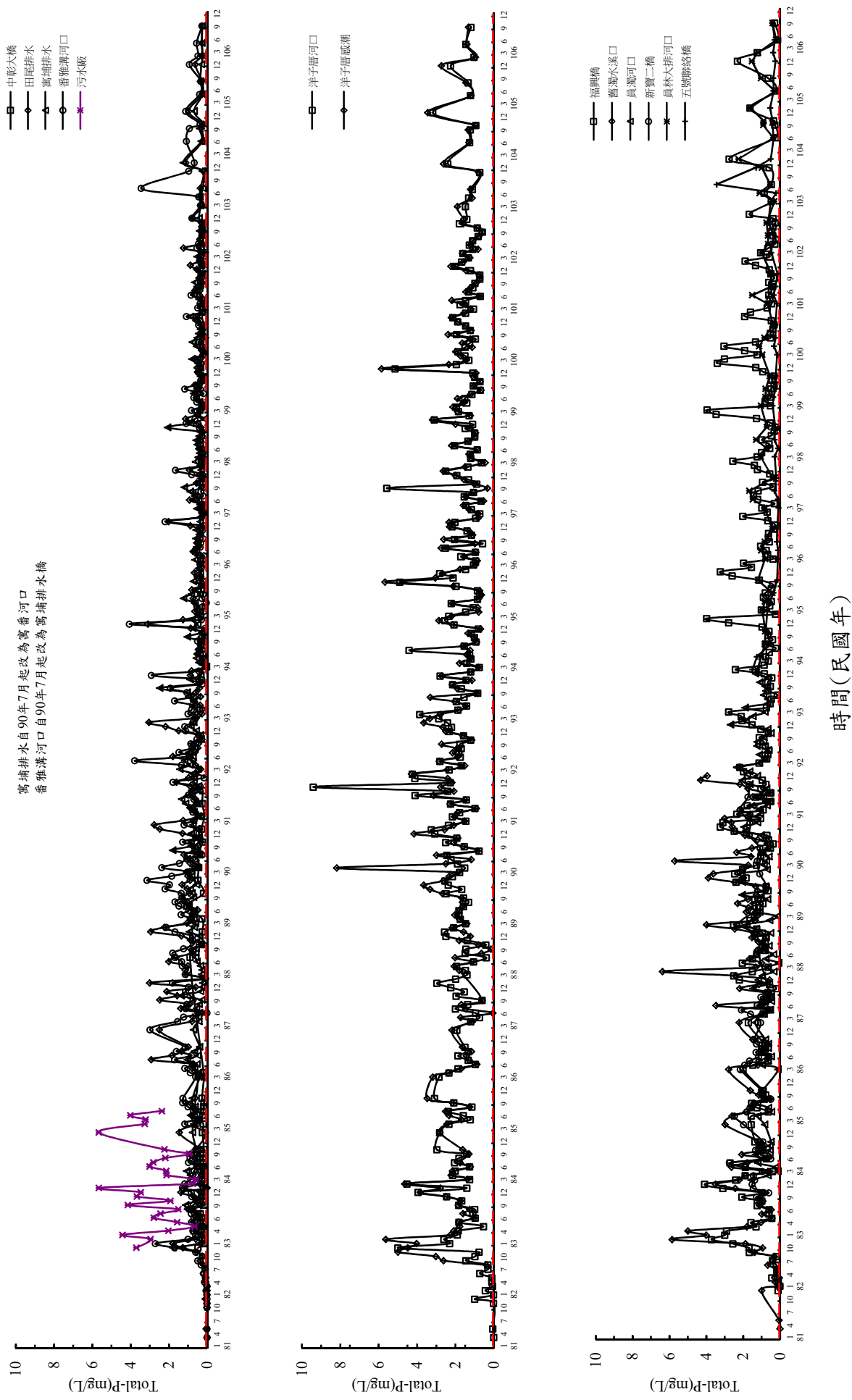
附圖III.7-14 歷次彰濱河口退潮總磷調查結果
