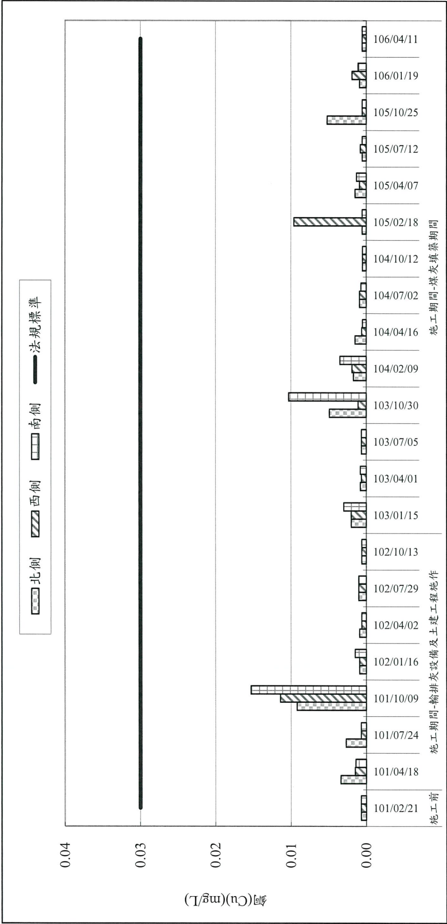
圖 2.2-7 歷季各測站銅(Cu)監測成果彙整
