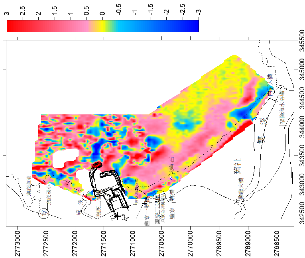
圖3.1-17 核四環境監測海岸地形109年6月與 87年6月侵淤比較圖
