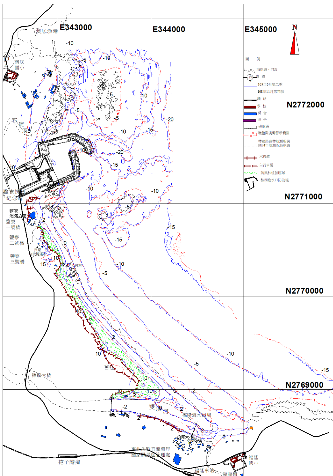
圖 2.5-5 核四封存期間海岸地形 109 年第 2 季與 108 年第 4 季監測結果比較
