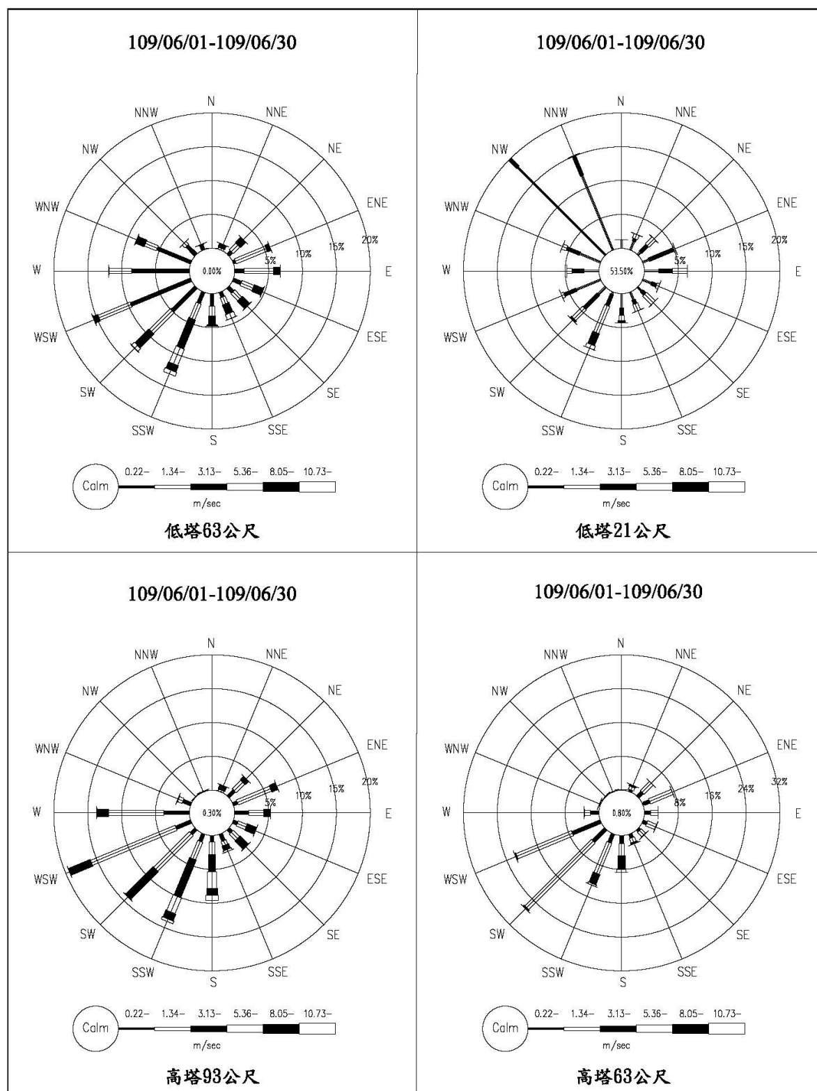
圖 2.1-2 核四封存期間環境監測氣象塔 109 年 6 月風花圖
