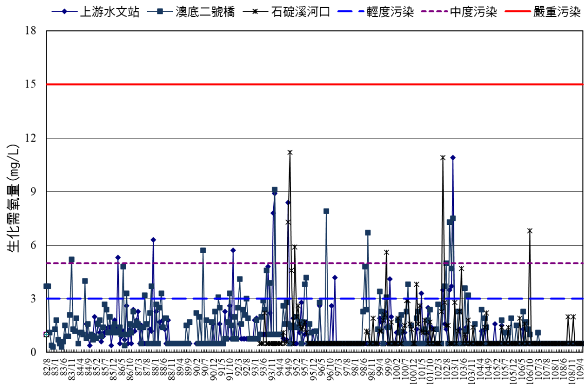
圖 3.1-3 核四環境監測河川水質歷年調查生化需氧量變化圖
