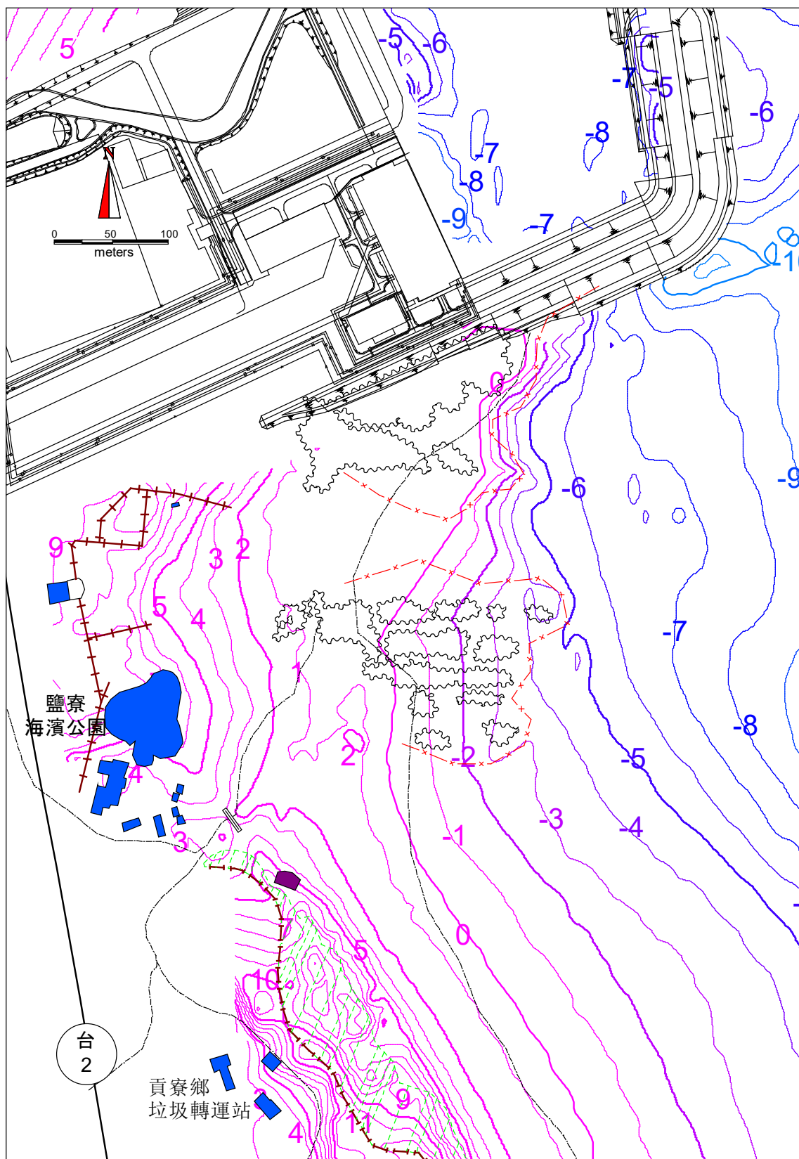
圖 2.5-3 核四封存期間鹽寮公園附近 109 年第 2 季 海岸地形監測結果
