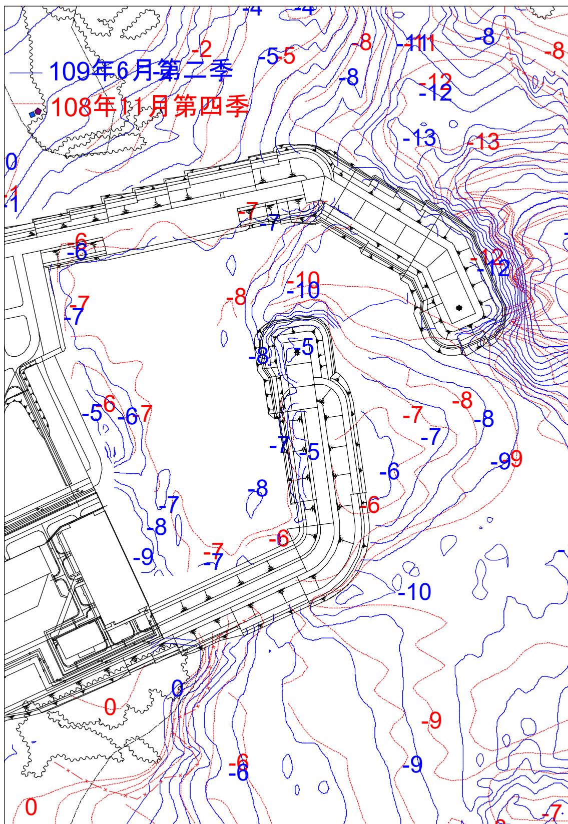
圖 3.1-11 核四環境監測海岸地形進水口防坡堤 109 年第 2 季與 108 年第 4 季監測結果比較
