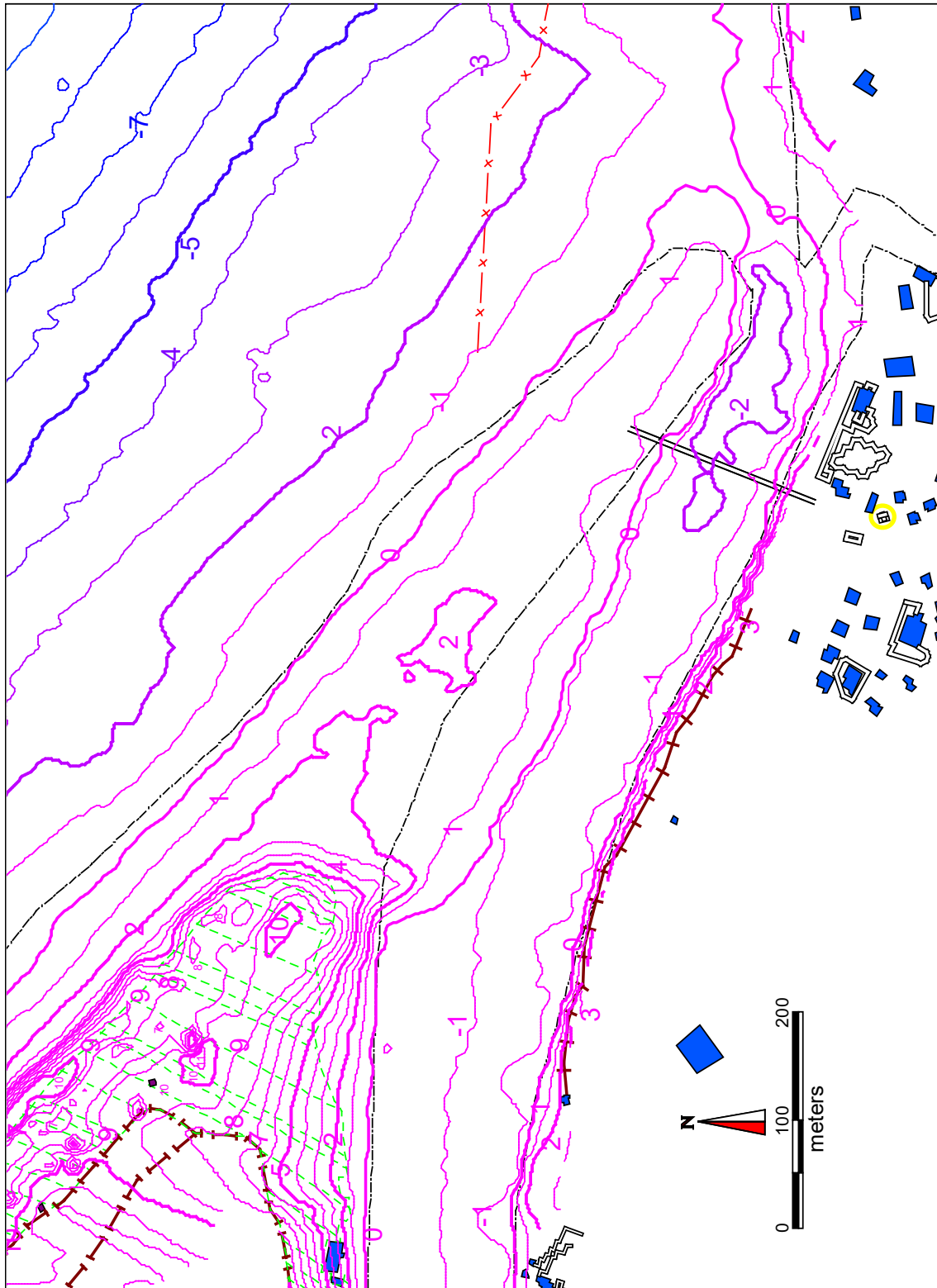
圖 2.5-4 核四封存期間福隆附近 109 年第 2 季海岸地形監測結果
