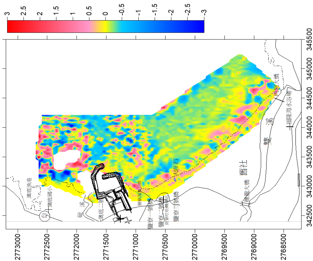
圖3.1-15 核四環境監測海岸地形109年6月與 108年11月鹽寮侵淤比較圖
