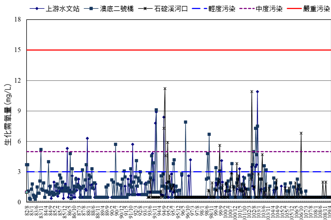
核四封存期間環境監測歷年河川水質之生化需氧量監測結果變化圖
