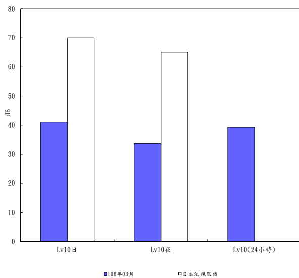
圖 2.3-5 海埔國小日本季振動調查結果分析圖
