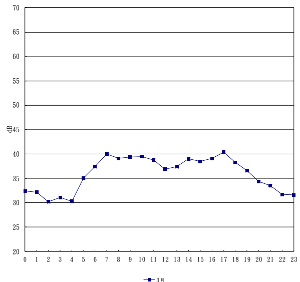
圖 2.3-6 海埔國小日本季振動測值逐時變化圖
