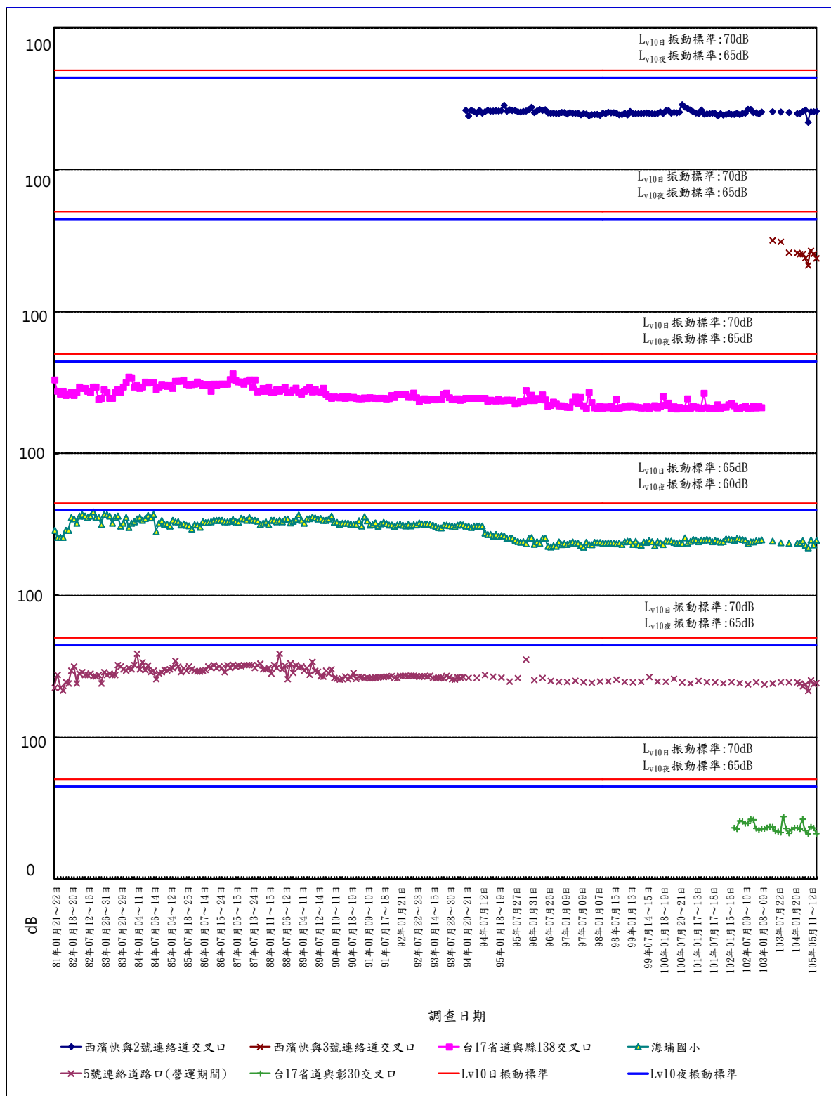
圖 3.1.3-1 彰濱地區歷次振動 L_{v10}(24 \text{ 小時}) 監測結果
