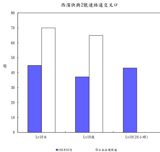
圖 2.3-1 西濱快與2號連絡道交叉口日本季振動調查結果分析圖
