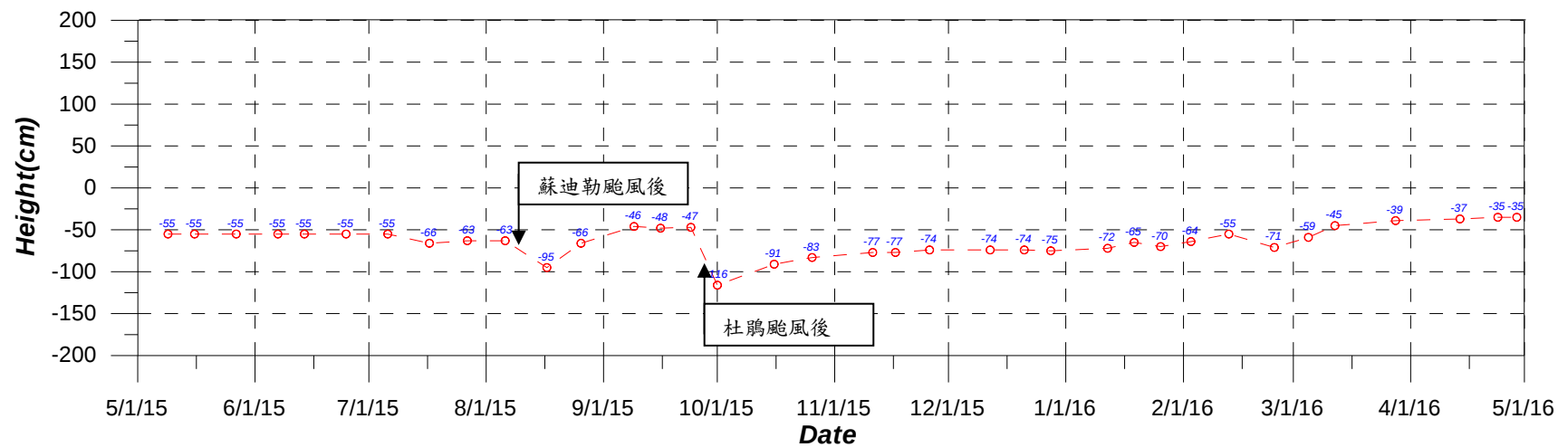
監測區 #O4 樁觀測紀錄圖
