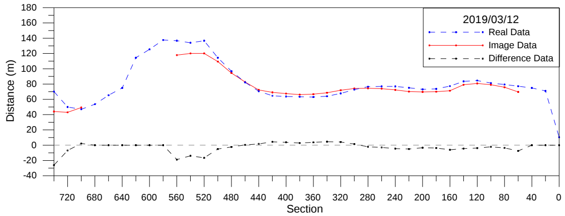
圖 3-23 海岸線分析比較圖(2019/3/12)
