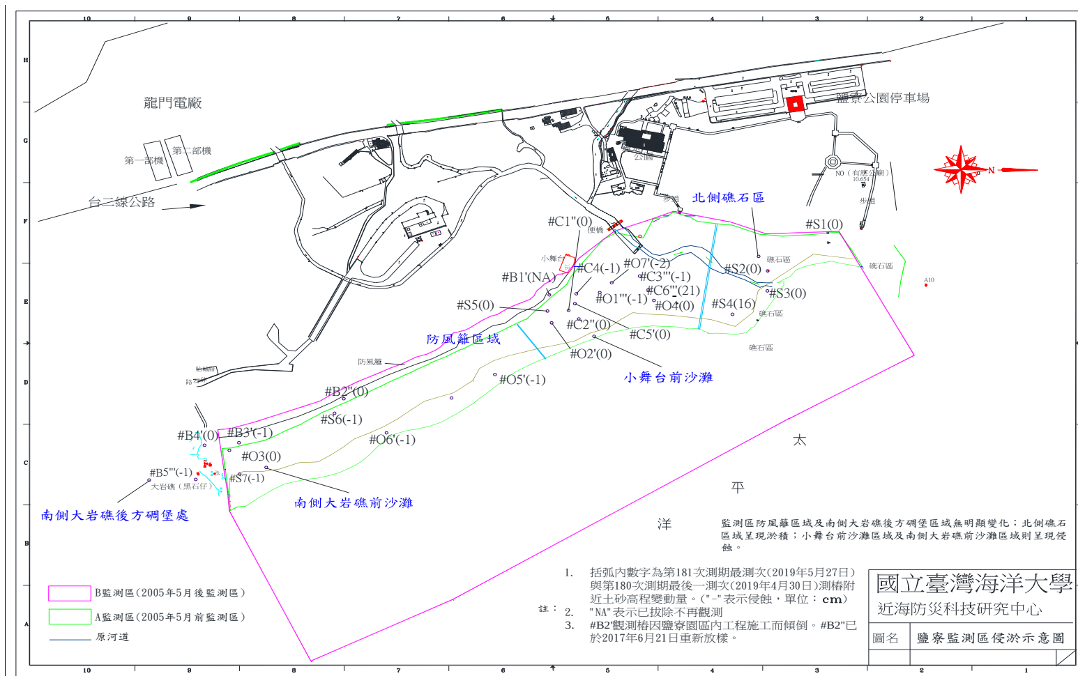
圖 1-1 鹽寮海岸短期性養灘監測各區域土砂高程變化圖
