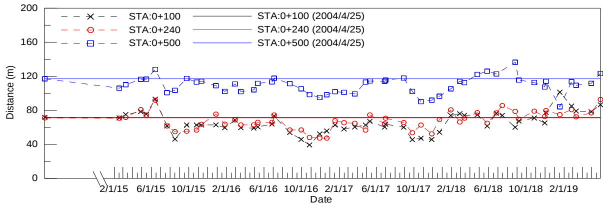
圖 4-16 海岸線斷面沙灘寬度變化圖(斷面編號：0+100、0+240、0+500)
