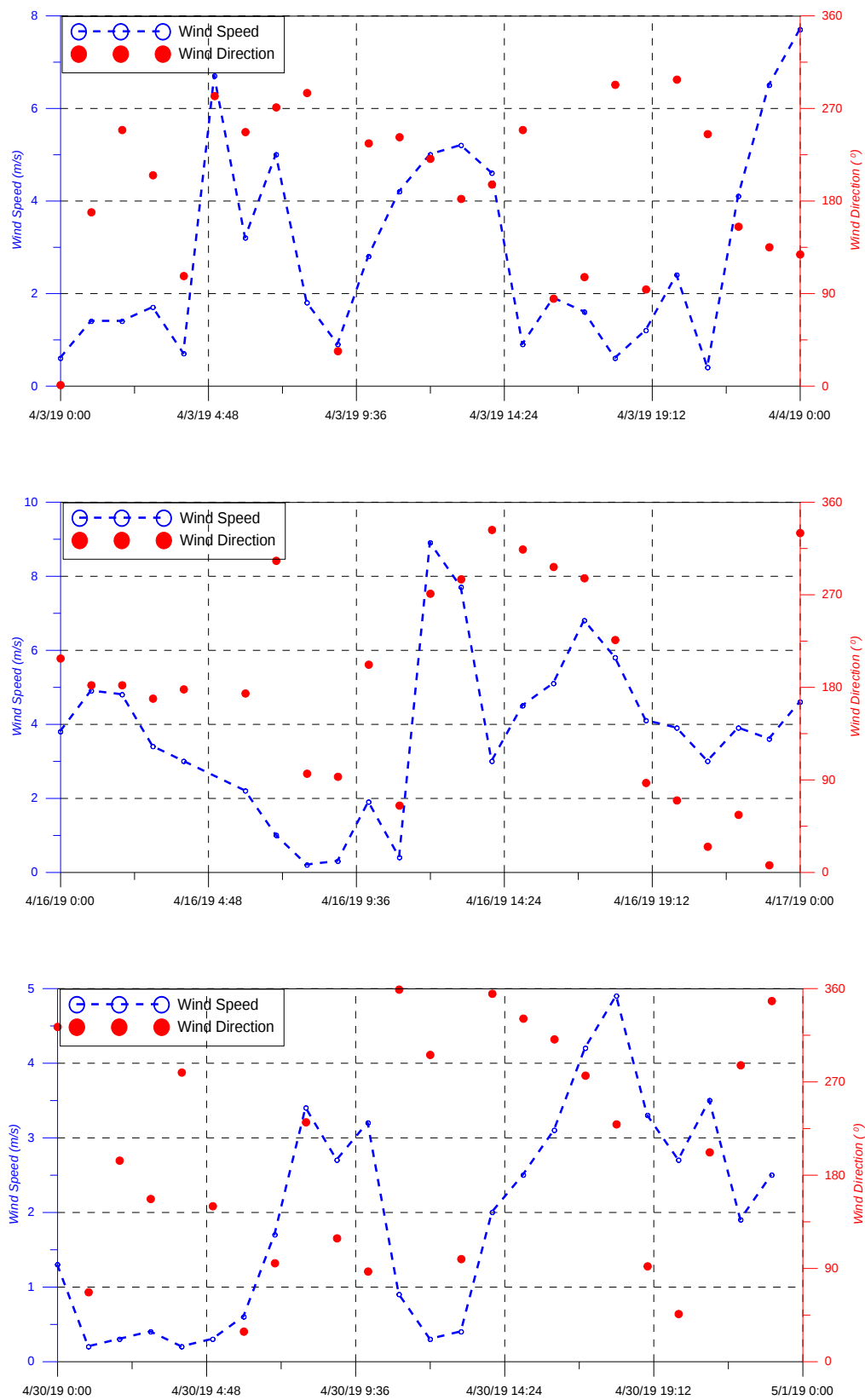
圖 2-2 風速風向時序序列變化圖
