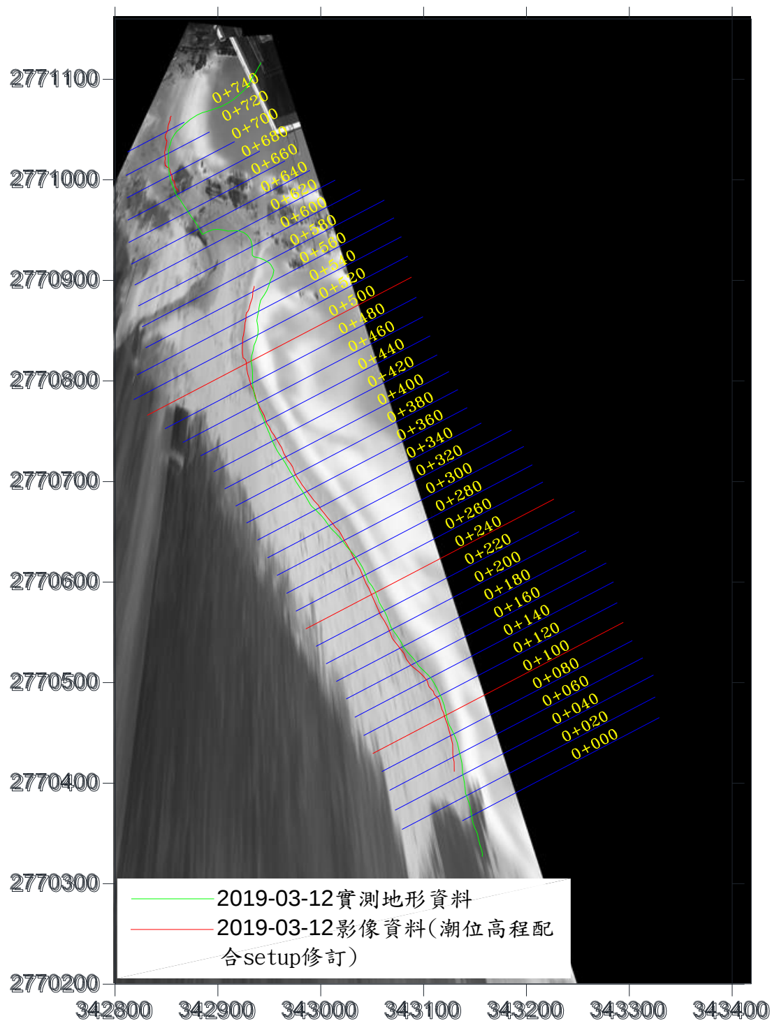
圖 3-22 水位線分析結果圖(2019/3/12)
