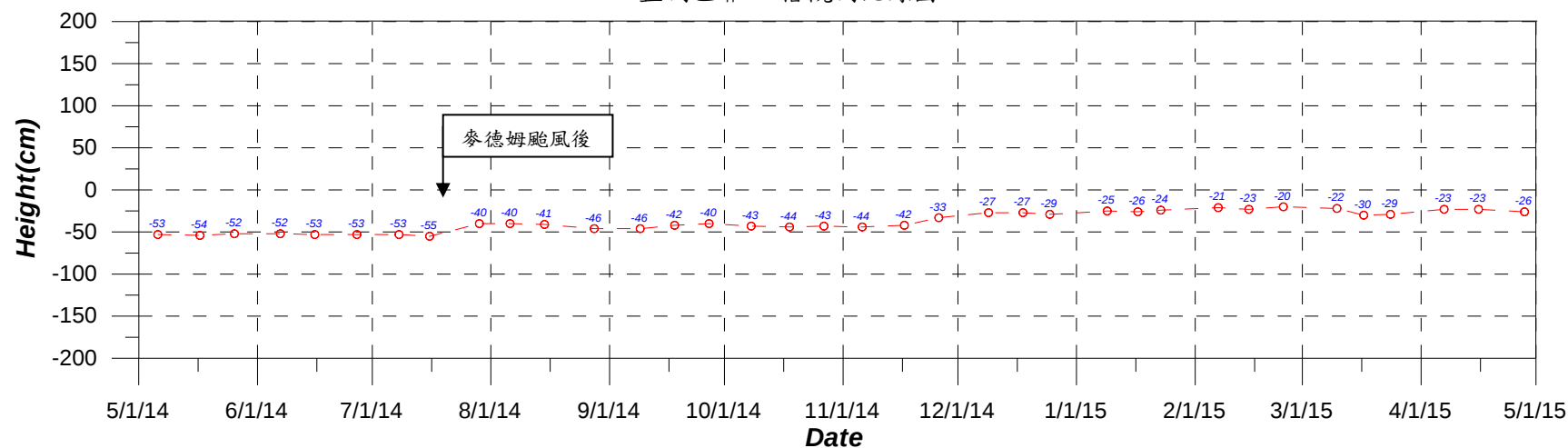
監測區 #S6 椿觀測紀錄圖
