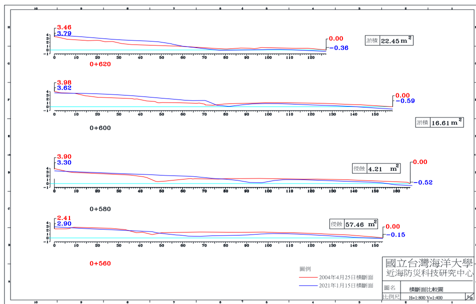
圖 4-4(c) 2021 年 1 月 15 日 A 監測區橫斷面比較圖
