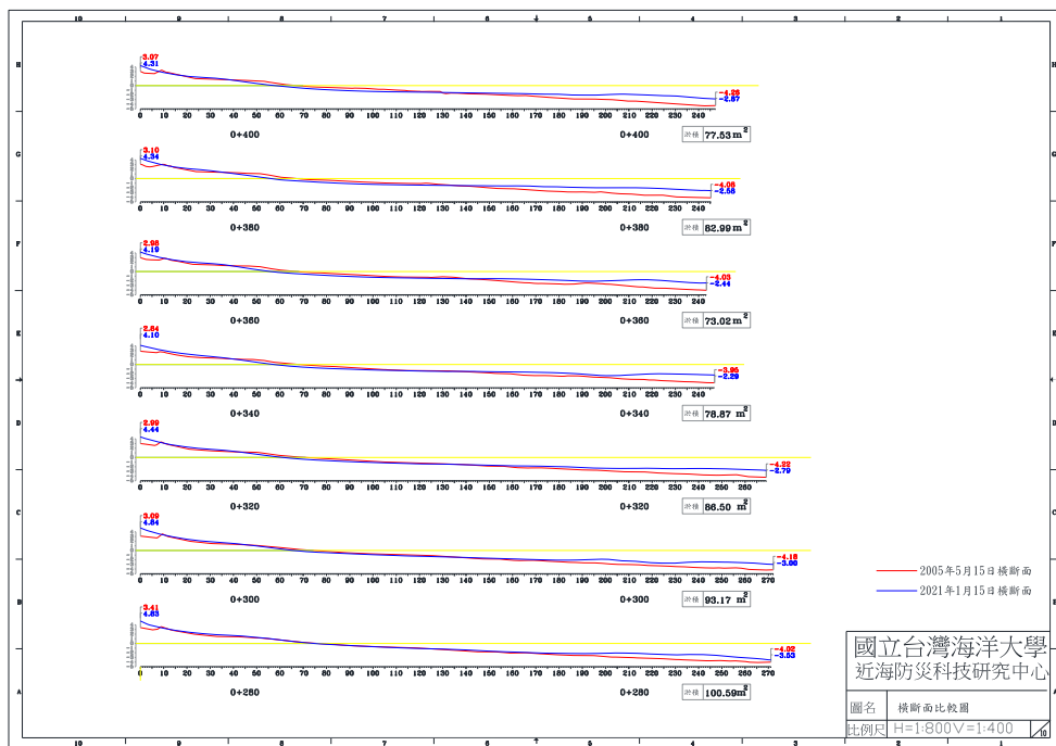
圖 4-5(d) 2021 年 1 月 15 日 B 監測區橫斷面比較圖
