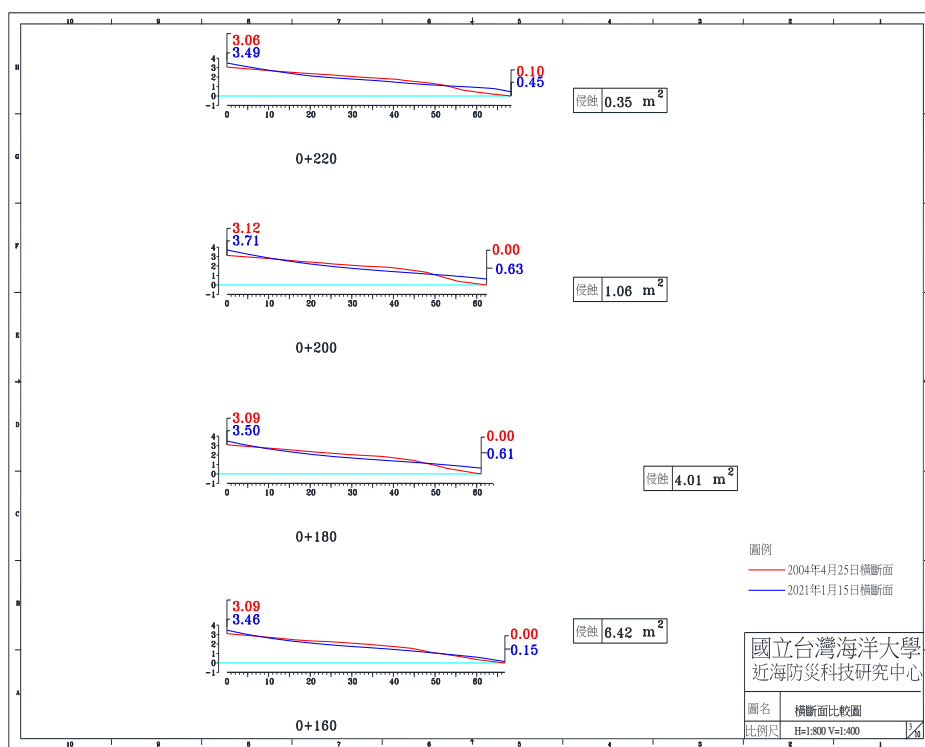
圖 4-4(h) 2021 年 1 月 15 日 A 監測區橫斷面比較圖
