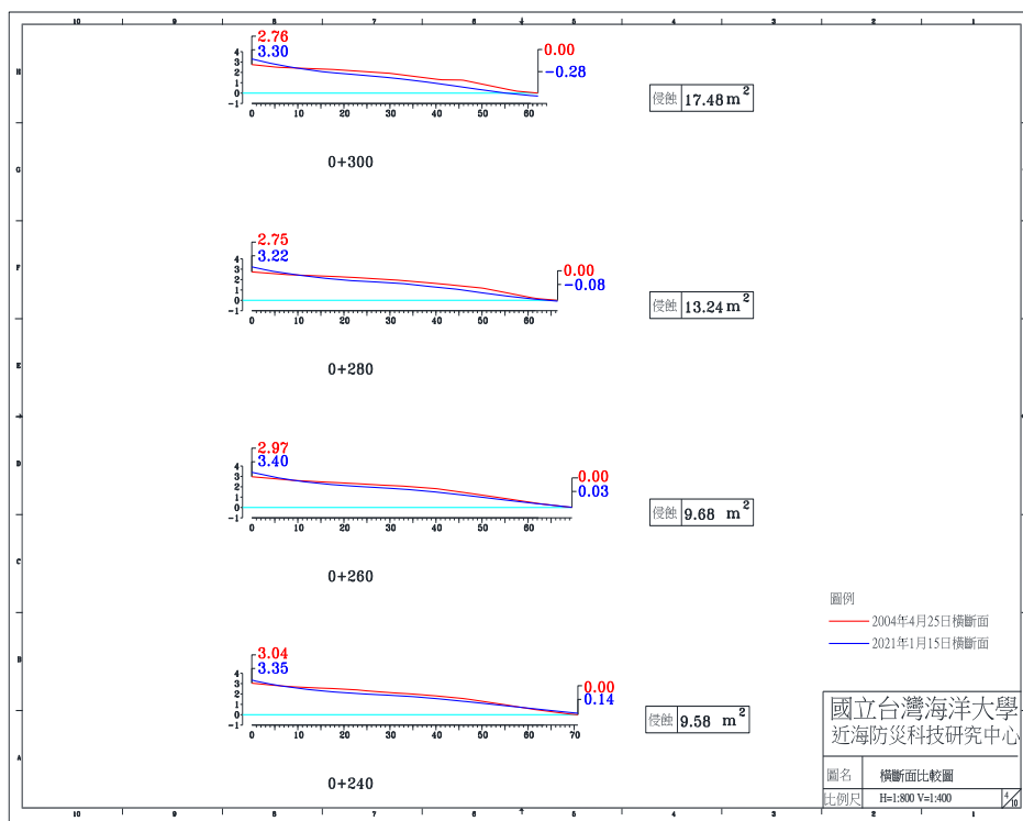
圖 4-4(g) 2021 年 1 月 15 日 A 監測區橫斷面比較圖
