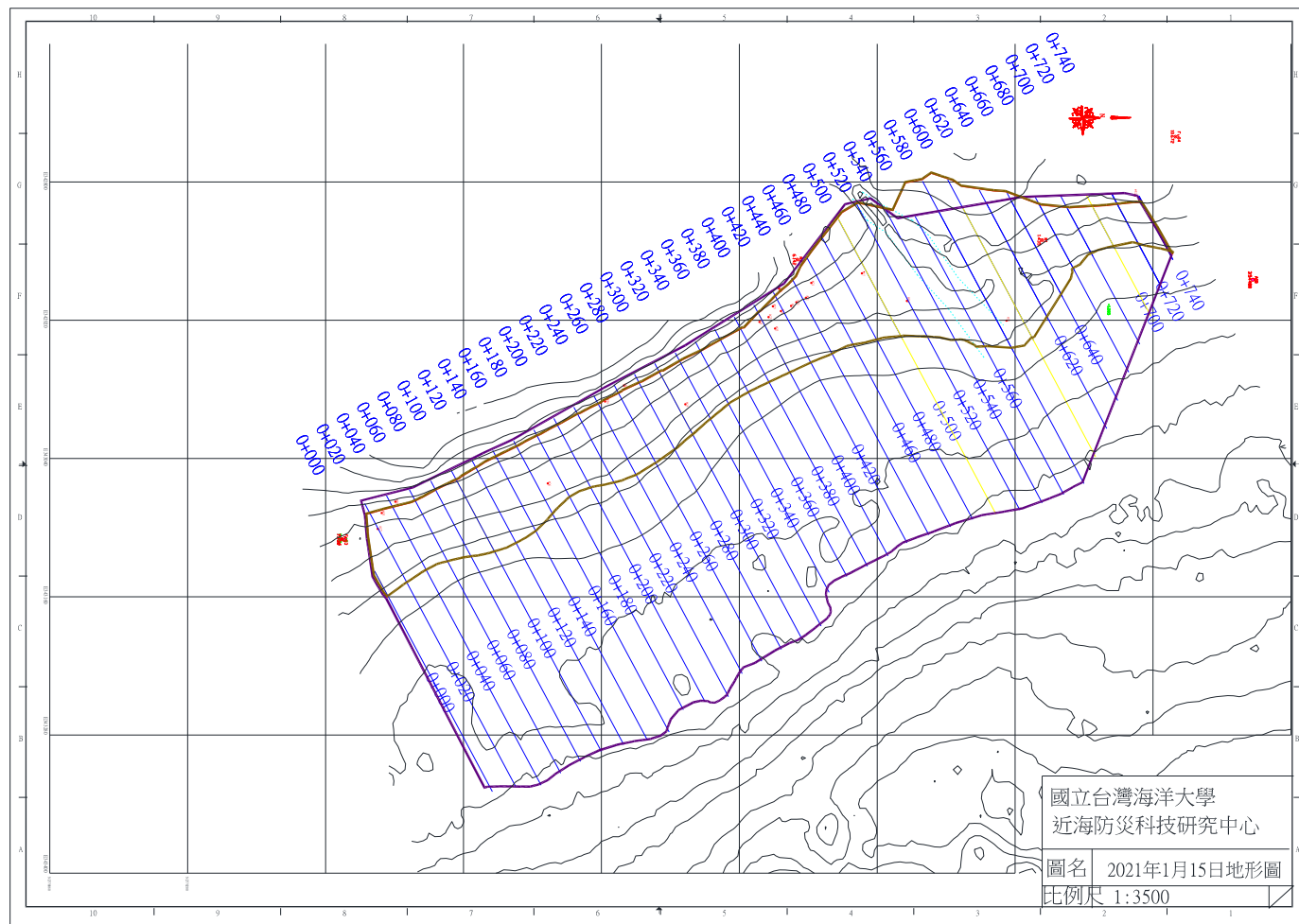
圖 4-1 2021 年 1 月 15 日監測地形圖
