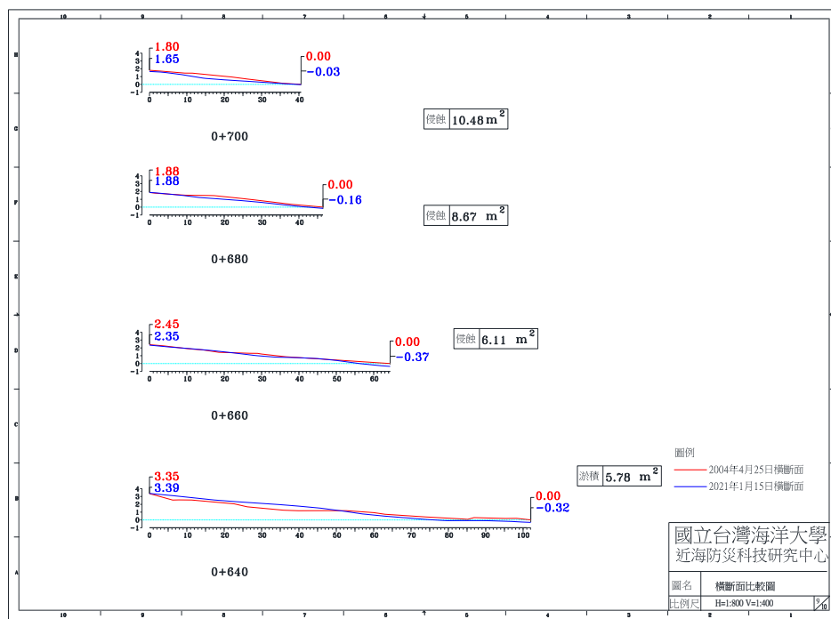
圖 4-4(b) 2021 年 1 月 15 日 A 監測區橫斷面比較圖
