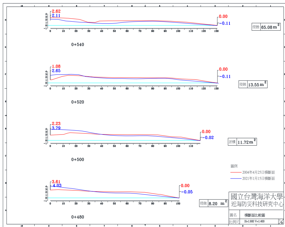
圖 4-4(d) 2021 年 1 月 15 日 A 監測區橫斷面比較圖
