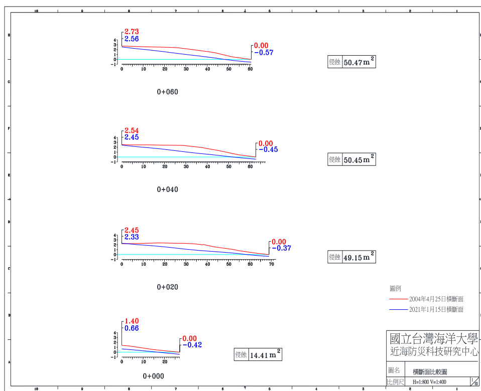
圖 4-4(j) 2021 年 1 月 15 日 A 監測區橫斷面比較圖
