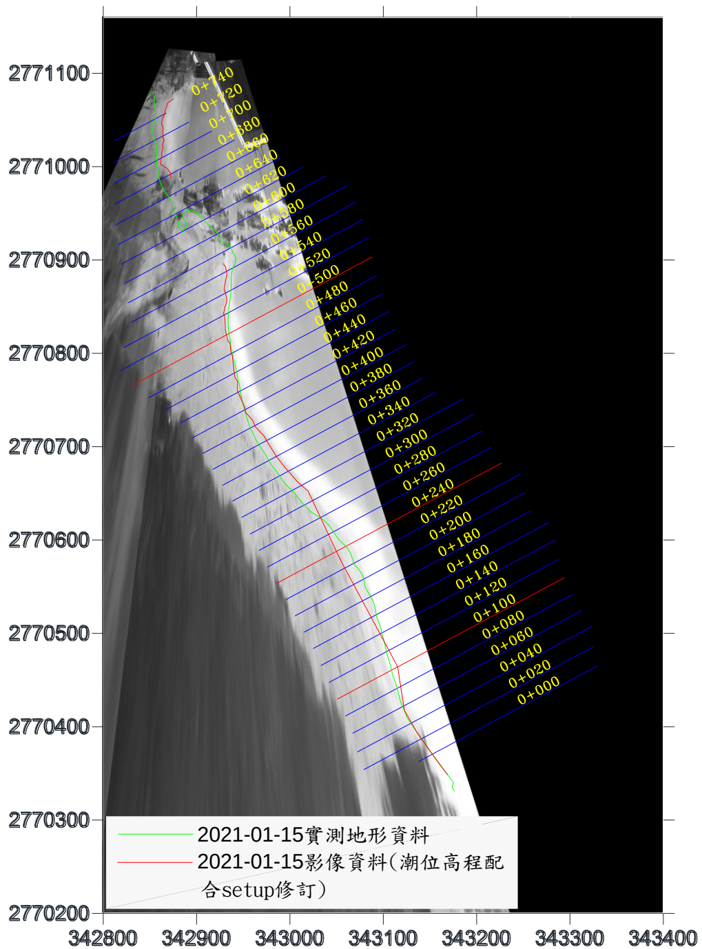
圖 3-22 水位線分析結果圖(2021/1/15)
