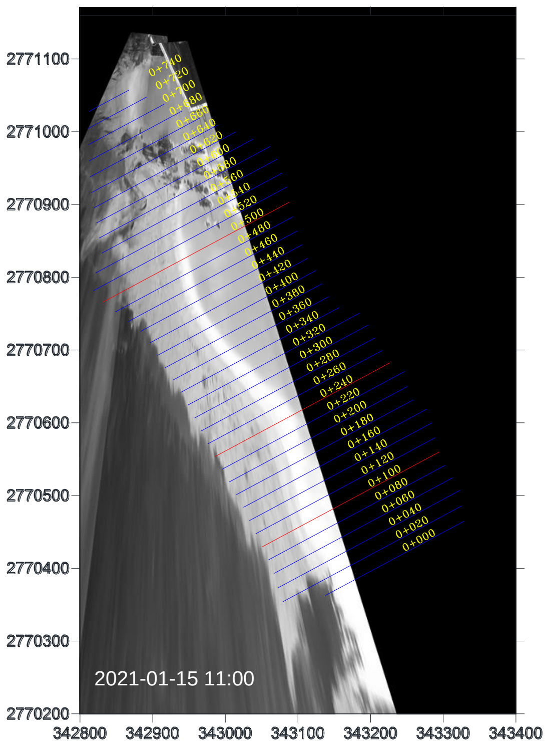
圖 4-19 鹽寮海岸地形影像全景圖(2021/01/15 11:00)
