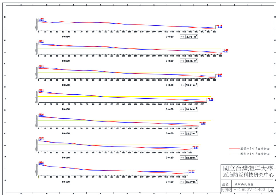
圖 4-5(c) 2021 年 1 月 15 日 B 監測區橫斷面比較圖
