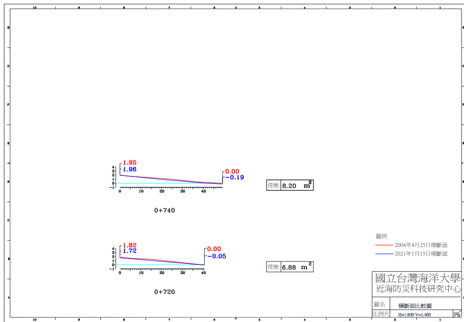
圖 4-4(a) 2021 年 1 月 15 日 A 監測區橫斷面比較圖
