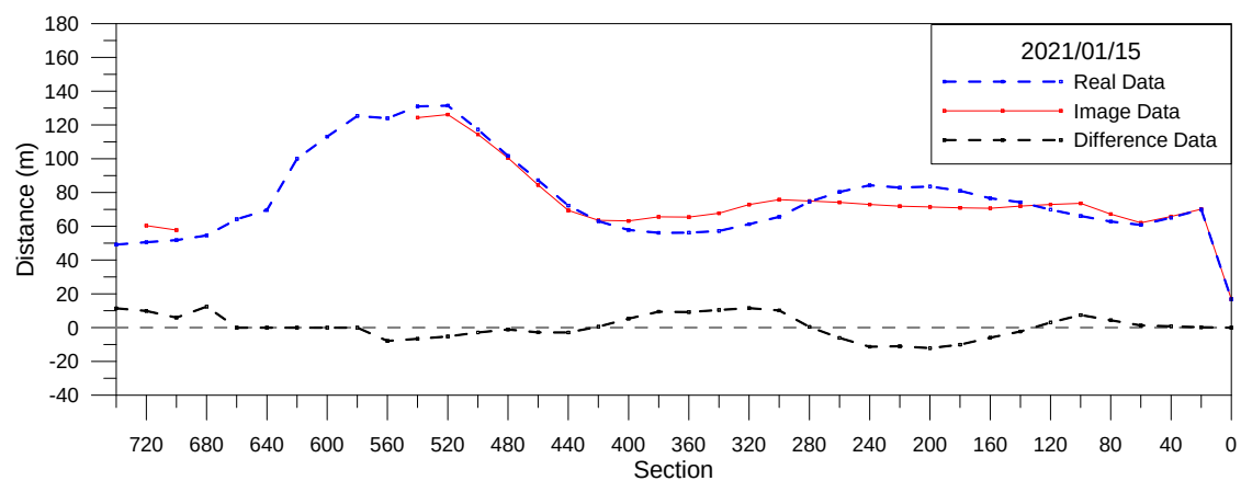
圖 3-23 海岸線分析比較圖(2021/1/15)
