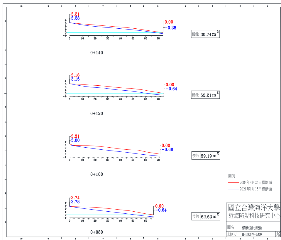
圖 4-4(i) 2021 年 1 月 15 日 A 監測區橫斷面比較圖
