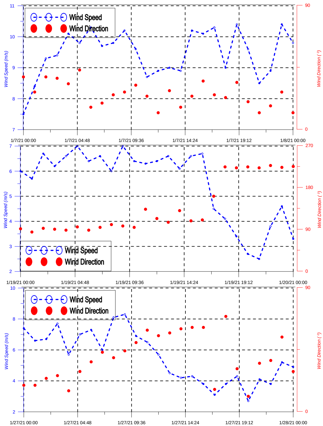
圖 2-2 風速風向時序列變化圖
