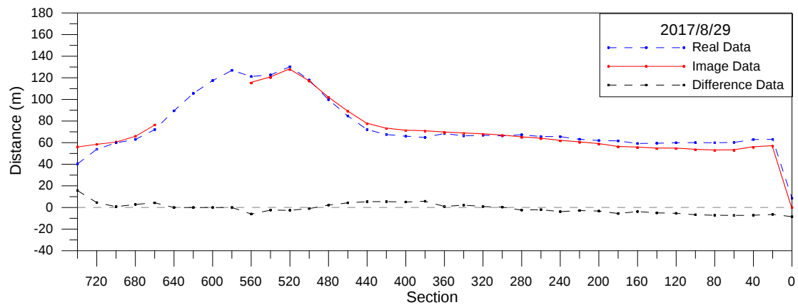
圖 3-23 海岸線分析比較圖(2017/8/29)
