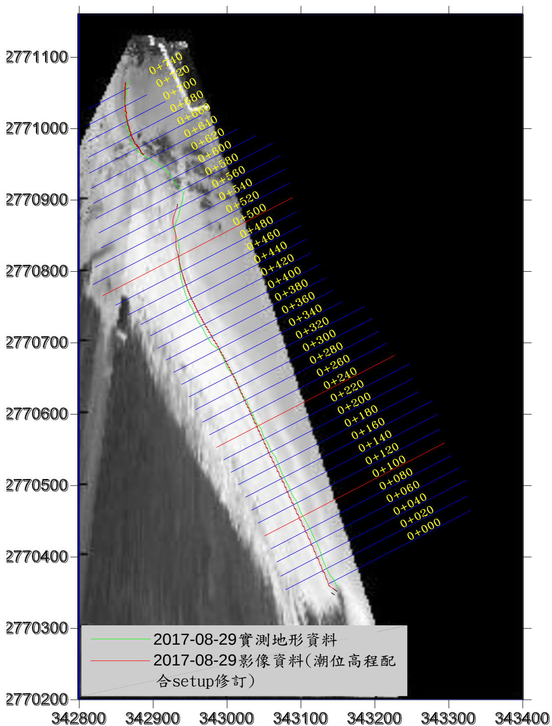
圖 3-22 水位線分析結果圖(2017/8/29)
