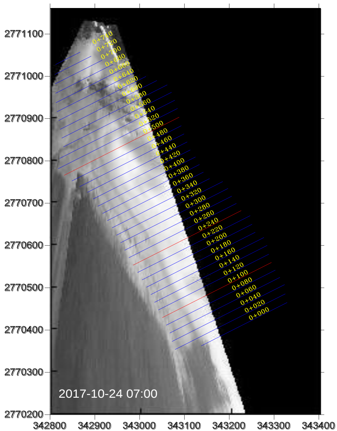
圖 4-14 鹽寮海岸地形影像全景圖(2017/10/24 7:00)
