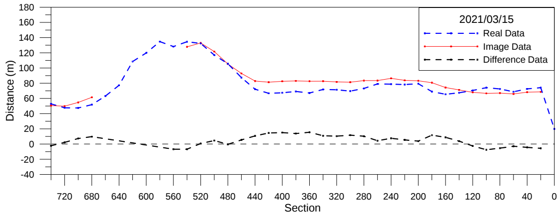
圖 3-23 海岸線分析比較圖(2021/03/15)
