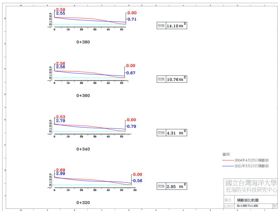
圖 4-4(f) 2021 年 5 月 13 日 A 監測區橫斷面比較圖
