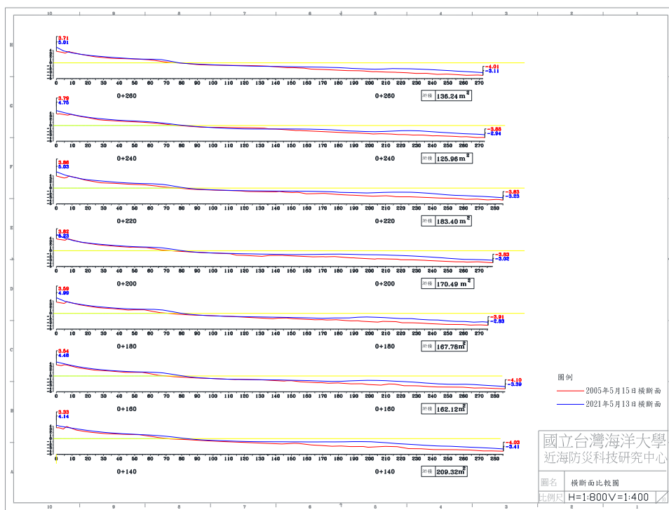
圖 4-5(e) 2021 年 5 月 13 日 B 監測區橫断面比較圖
