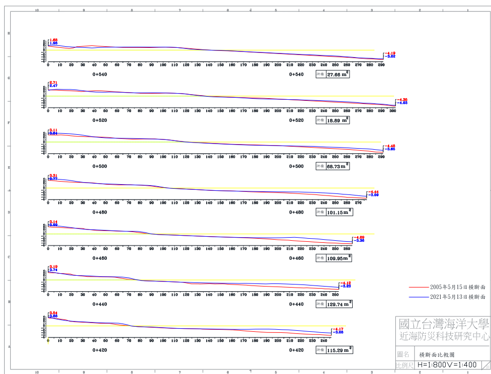
圖 4-5(c) 2021 年 5 月 13 日 B 監測區橫斷面比較圖
