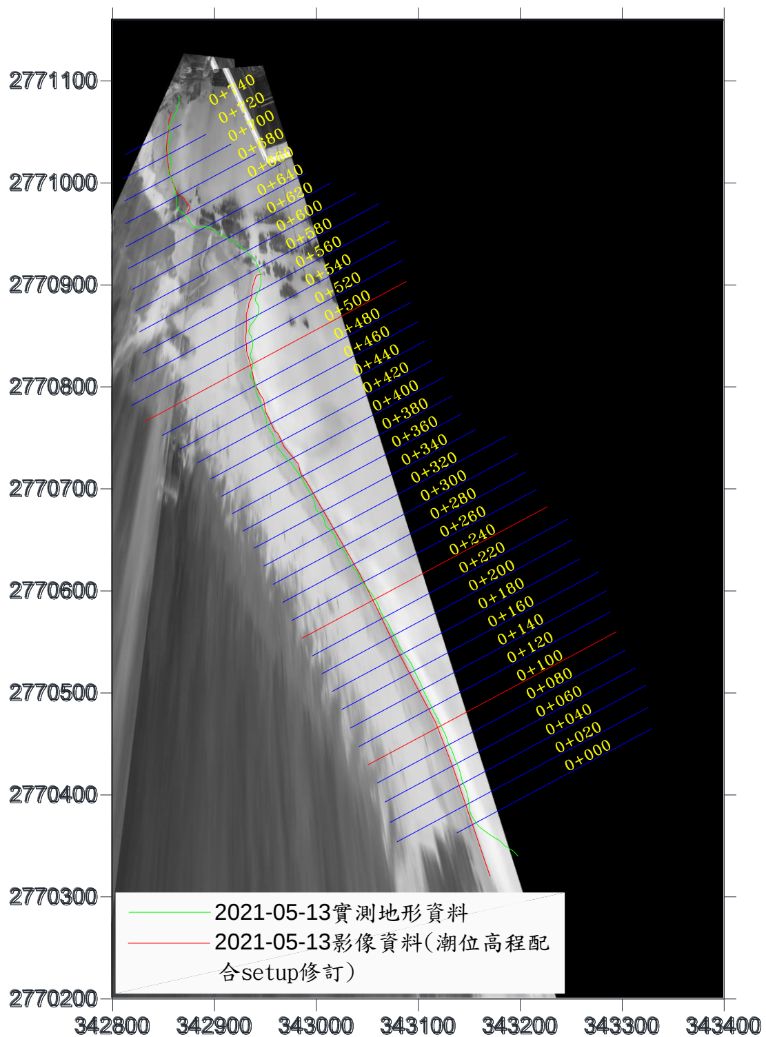
圖 3-22 水位線分析結果圖(2021/05/13)
