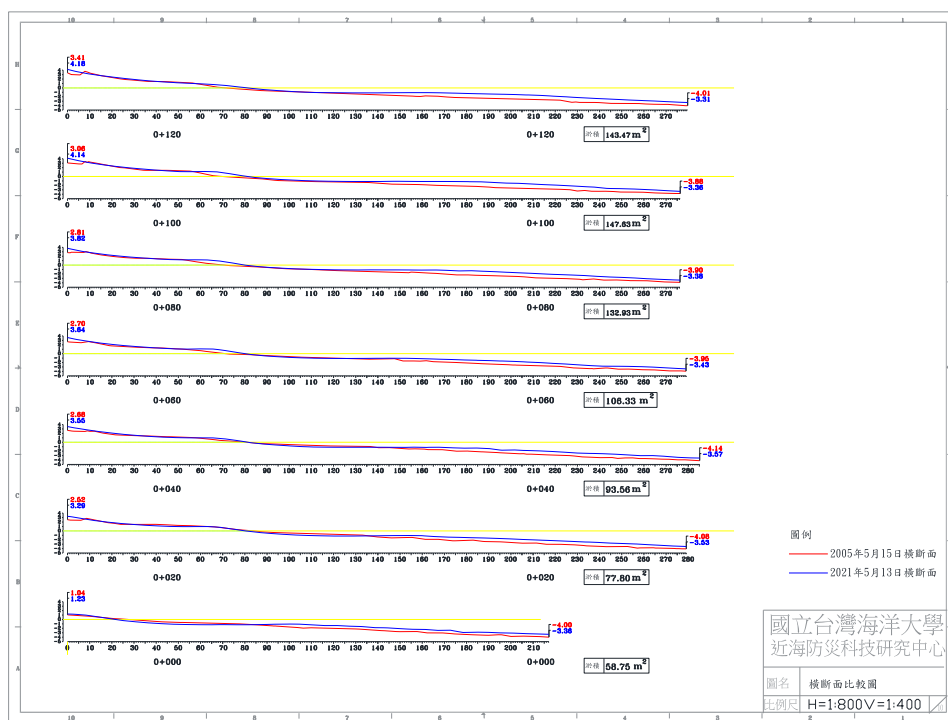
圖 4-5(f) 2021 年 5 月 13 日 B 監測區橫断面比較圖
