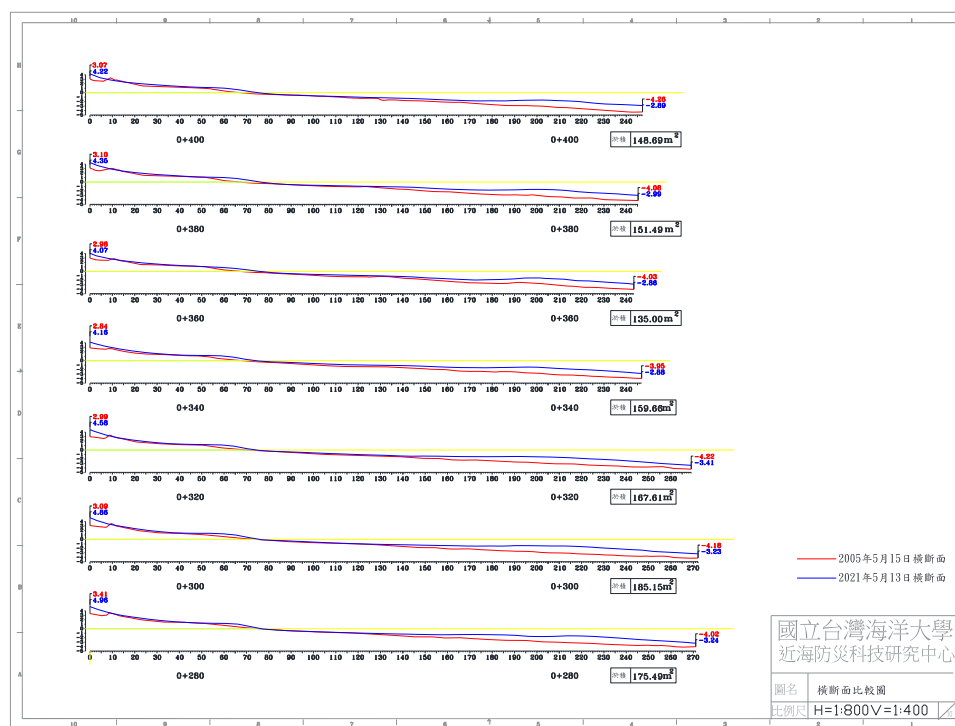
圖 4-5(d) 2021 年 5 月 13 日 B 監測區橫斷面比較圖
