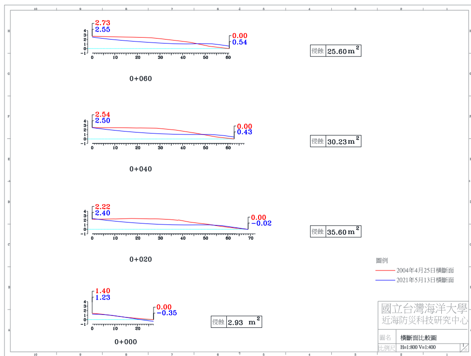
圖 4-4(j) 2021 年 5 月 13 日 A 監測區橫斷面比較圖
