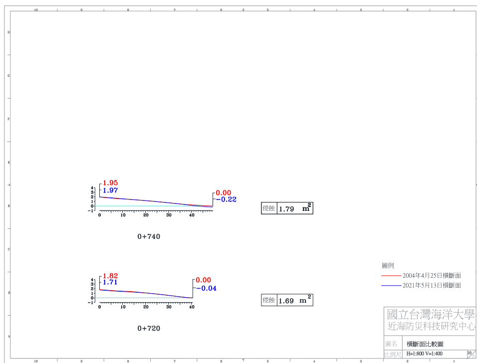
圖 4-4(a) 2021 年 5 月 13 日 A 監測區橫斷面比較圖
