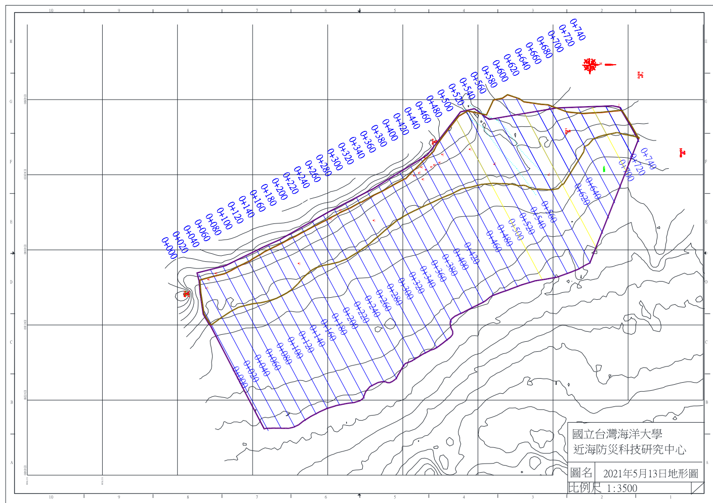
圖 4-1 2021 年 5 月 13 日監測地形圖
