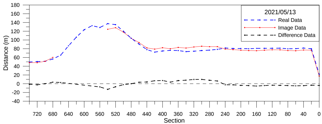
圖 3-23 海岸線分析比較圖(2021/05/13)
