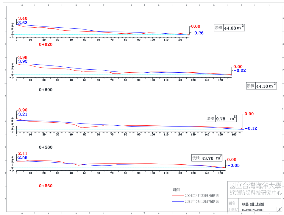
圖 4-4(c) 2021 年 5 月 13 日 A 監測區橫斷面比較圖
