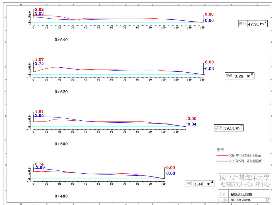
圖 4-4(d) 2021 年 5 月 13 日 A 監測區橫斷面比較圖
