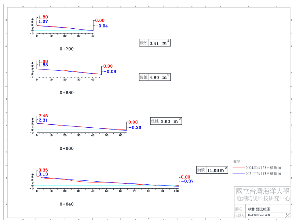
圖 4-4(b) 2021 年 5 月 13 日 A 監測區橫斷面比較圖
