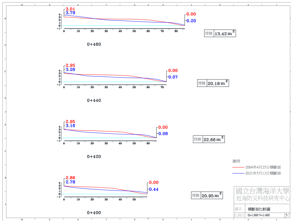
圖 4-4(e) 2021 年 5 月 13 日 A 監測區橫斷面比較圖
