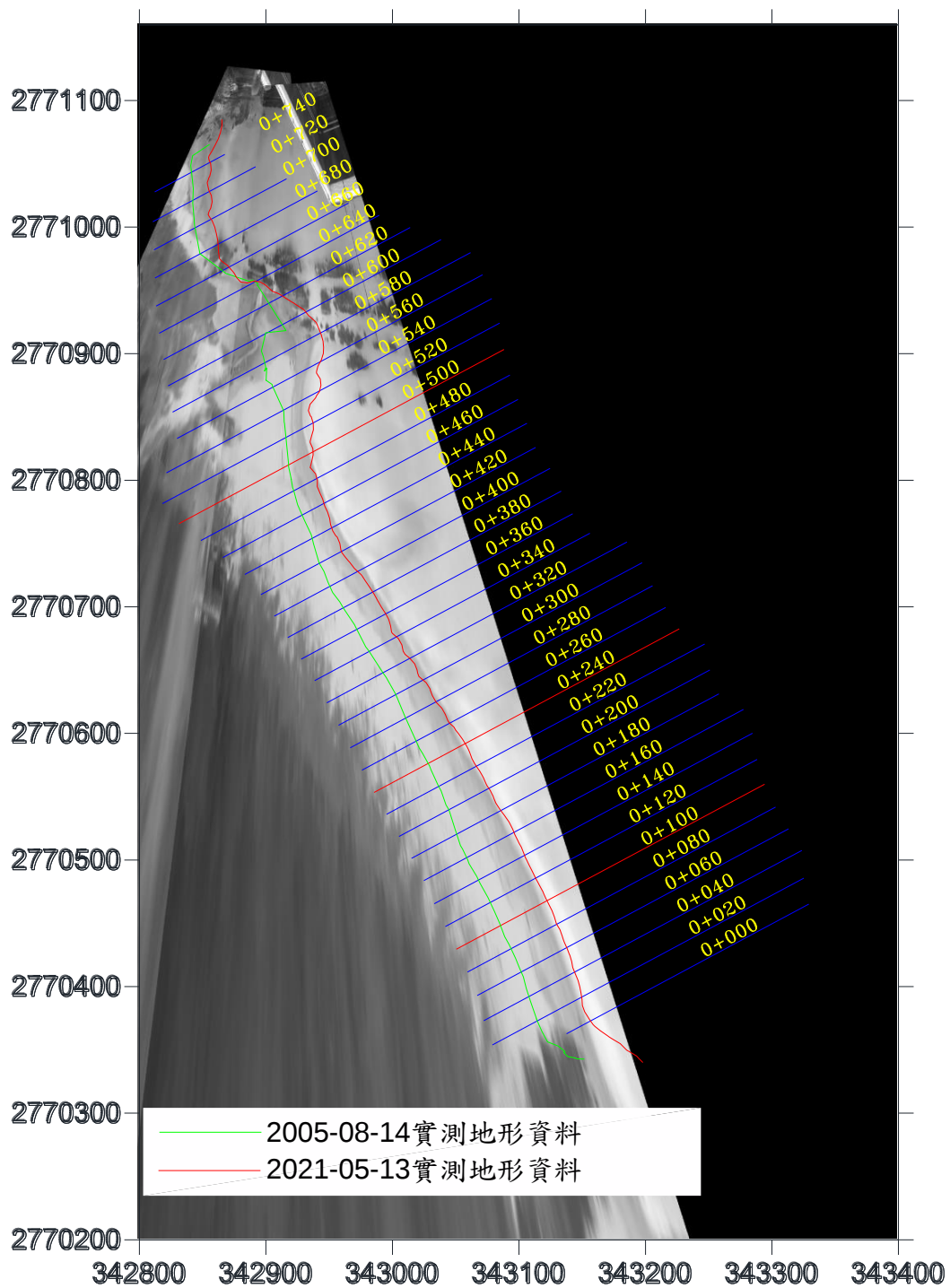
圖 4-22 實測地形水位線分析結果圖(2021/05/13)
