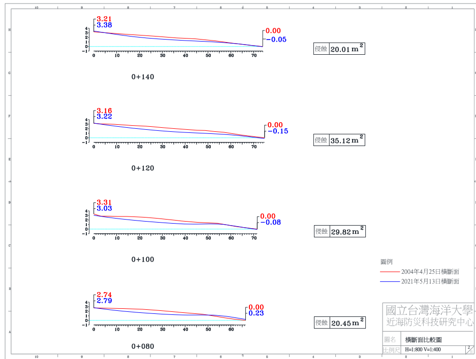
圖 4-4(i) 2021 年 5 月 13 日 A 監測區橫斷面比較圖
