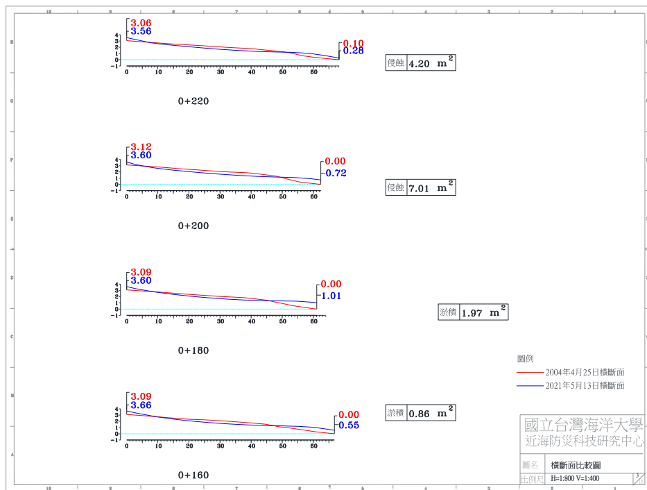
圖 4-4(h) 2021 年 5 月 13 日 A 監測區橫斷面比較圖
