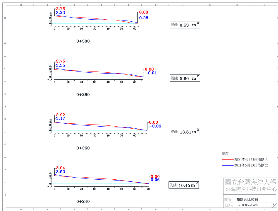
圖 4-4(g) 2021 年 5 月 13 日 A 監測區橫斷面比較圖
